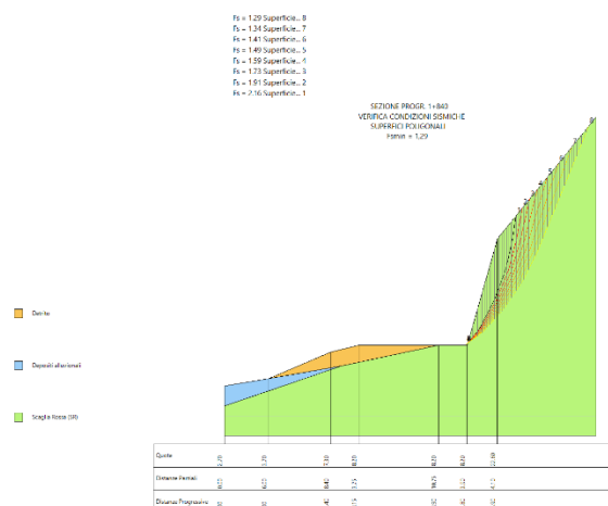
Figura 11.17 – Progressiva Km 1+840 – Verifica con Hoek & Bray
