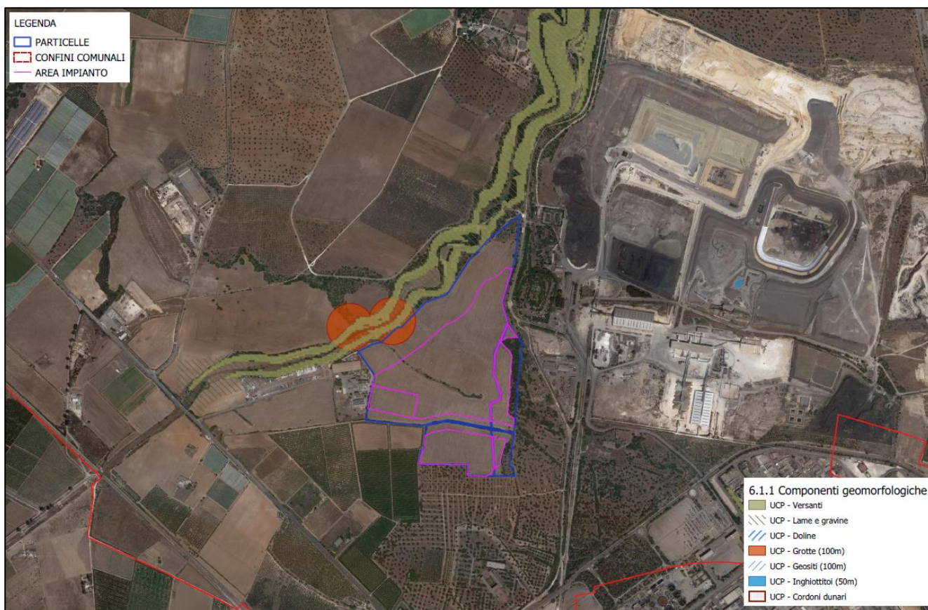
Figura 3-4: Componenti geomorfologiche - individuazione di BP e UCP nell'area di impianto
