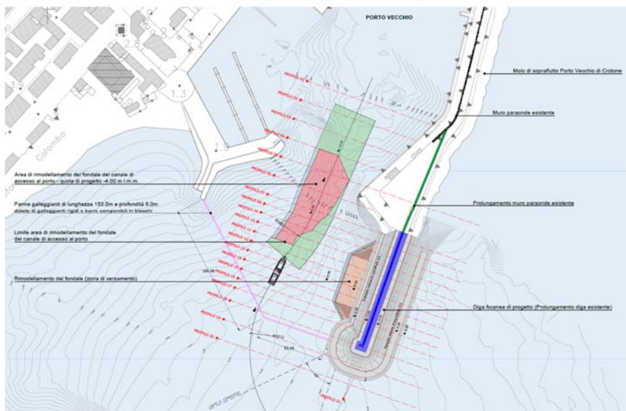
Figura 3.5 - Planimetria di progetto di rimodellamento dei fondali
