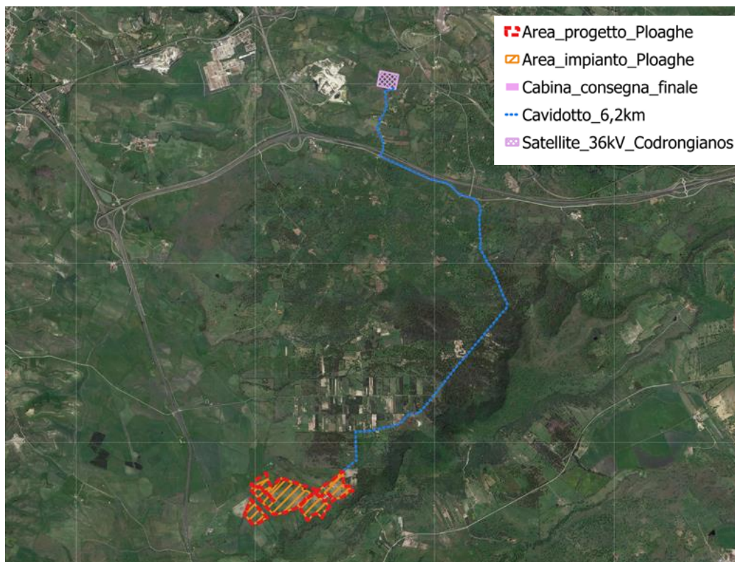
FIGURA 34 – ALTERNATIVA 2 DI IMPIANTO PER IL PROGETTO PLOAGHE (IMMAGINE AGGIORNATA)
