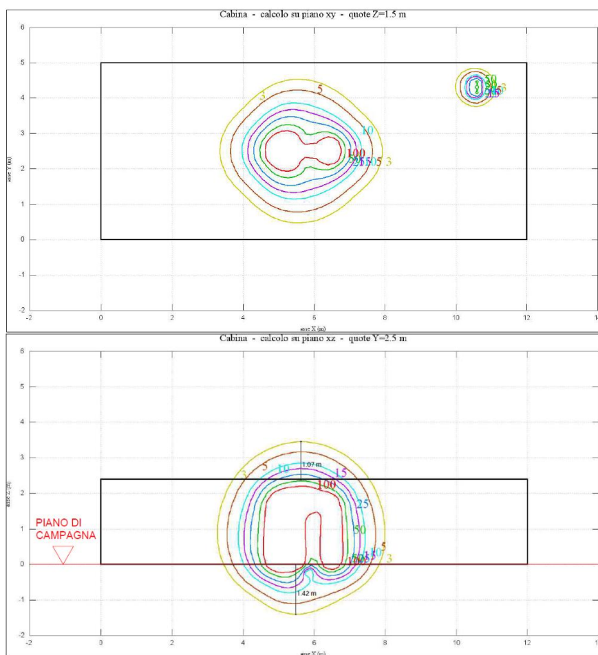
FIGURA 86 – CURVE ISOINDUZIONE CABINA AT CONSEGNA – PIANTE (IN ALTO) E PROSPETTO FRONTALE (IN BASSO). STRALCIO DELL'ELABORATO PLOAGHE-PDT13.
