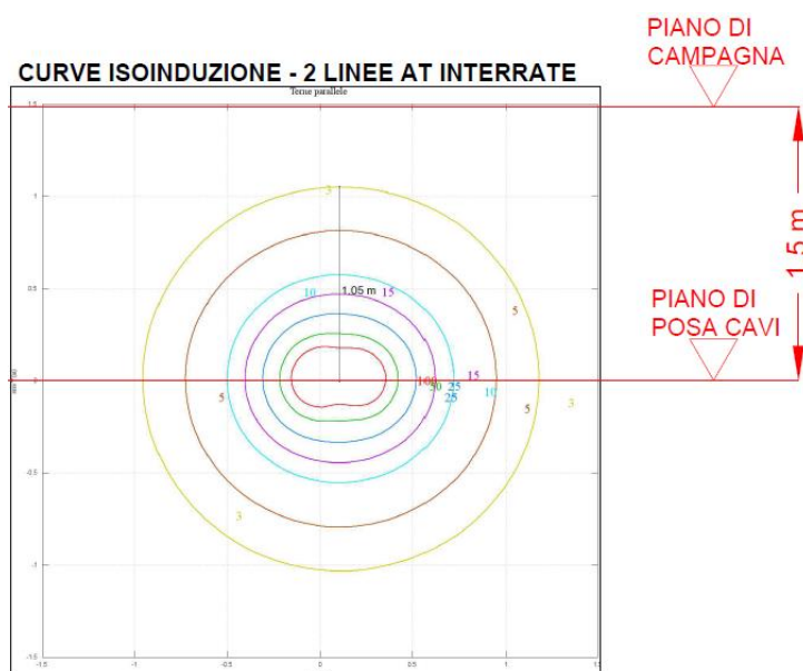
FIGURA 84 – CURVE ISOINDUZIONE – 2 LINEE AT INTERRATE (STRALCIO DELL'ELABORATO CARTOGRAFICO PLOAGHE-PDT13)
