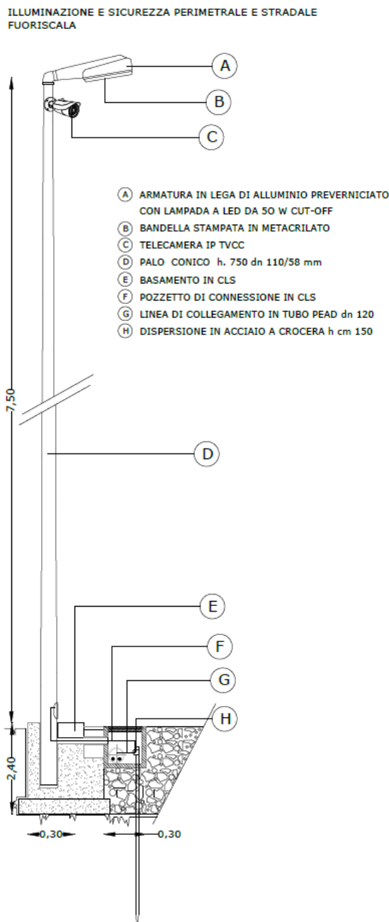
FIGURA 44 – ESEMPIO IMPIANTO DI ILLUMINAZIONE INTEGRATO CON SISTEMA DI VIDEOSORVEGLIANZA – ESTRATTO DALL'ELABORATO TECNICO PLOGHE-PDR02-R1
