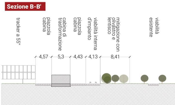
FIGURA 72 – PARTICOLARE FASCIA DI MITIGAZIONE CON VEGETAZIONE ESISTENTE E SEZIONE N-S DELL'IMPIANTO – ESTRATTO DALL'ELABORATO GRAFICO PLOAGHE-PDT11-R1) (IMMAGINE AGGIORNATA)
