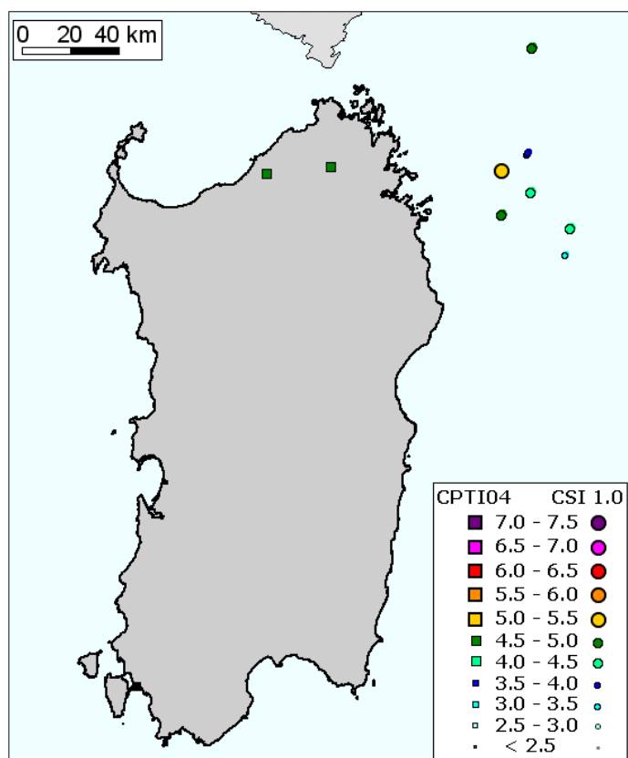
FIGURA 68 – DISTRIBUZIONE DEI TERREMOTI IN SARDEGNA E NEI MARI ADIACENTI.
