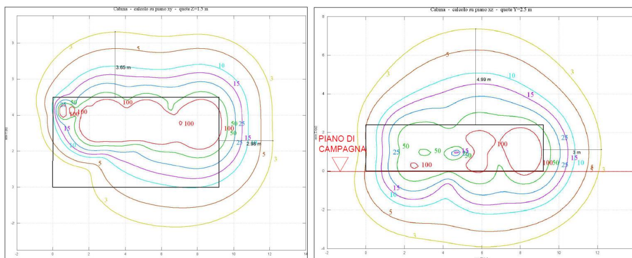
FIGURA 85 – CURVE ISOINDUZIONE AT/BT CABINA DI SOTTOCAMPO – VISTA IN PIANTA (A SX) E PROSPETTO (A DX). STRALCIO DELL'ELABORATO PLOAGHE-PDT13
