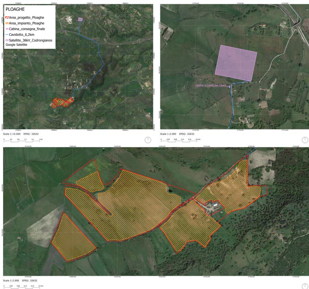
FIGURA 2 - ESTRATTO DALL'ELABORATO PLOAGHE-PDT01-R1_INQUADRAMENTO TERRITORIALE INTERVENTO SU ORTOFOTO (IMMAGINE AGGIORNATA)
