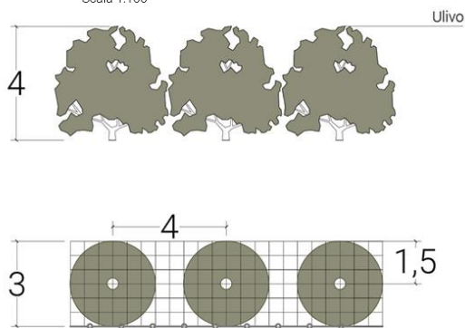
FIGURA 70 – PLANIMETRIA GENERALE SISTEMAZIONE A VERDE OPERE DI MITIGAZIONE E SCHEMA D'IMPIANTO (ESTRATTO DALL'ELABORATO GRAFICO PLOAGHE-PDT11-R1) (IMMAGINE AGGIORNATA)
