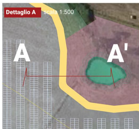
FIGURA 71 – PARTICOLARE FASCIA DI MITIGAZIONE DI NUOVO IMPIANTO E VIABILITÀ PERIMETRALE - SEZIONE O-E DELL'IMPIANTO (ESTRATTO DALL'ELABORATO GRAFICO PLOAGHE-PDT11-R1) (IMMAGINE AGGIORNATA)
