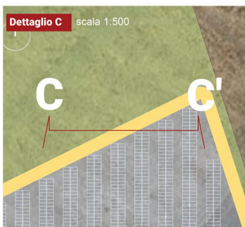
FIGURA 73 – PARTICOLARE AREA CABINA DI TRASFORMAZIONE E RELATIVA SEZIONE N-S DELL'IMPIANTO – ESTRATTO DALL'ELABORATO GRAFICO PLOAGHE-PDT11-R1) (IMMAGINE AGGIORNATA)
