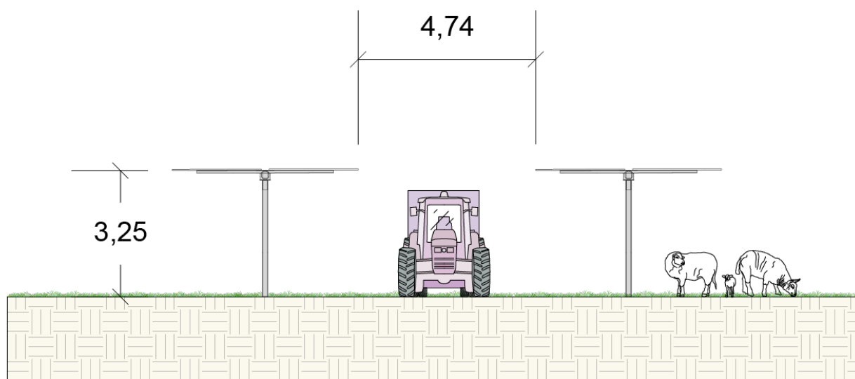
FIGURA 39 – SISTEMA AGRIVOLTAICO ELEVATO, SEZIONE TIPOLOGICA DELL'IMPIANTO
