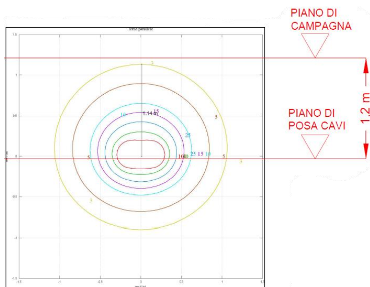
FIGURA 83 – CURVE ISOINDUZIONE – 3 LINEE BT INTERRATE (STRALCIO DELL'ELABORATO CARTOGRAFICO PLOAGHE-PDT13)
