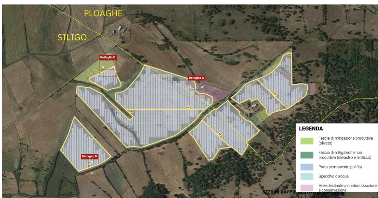
FIGURA 24 - PARTICOLARE FASCE DI MITIGAZIONE NON PRODUTTIVA (OLIVASTRO E LENTISCO) - ESTRATTO ELABORATO PLOAGHE-PDT11-R1
