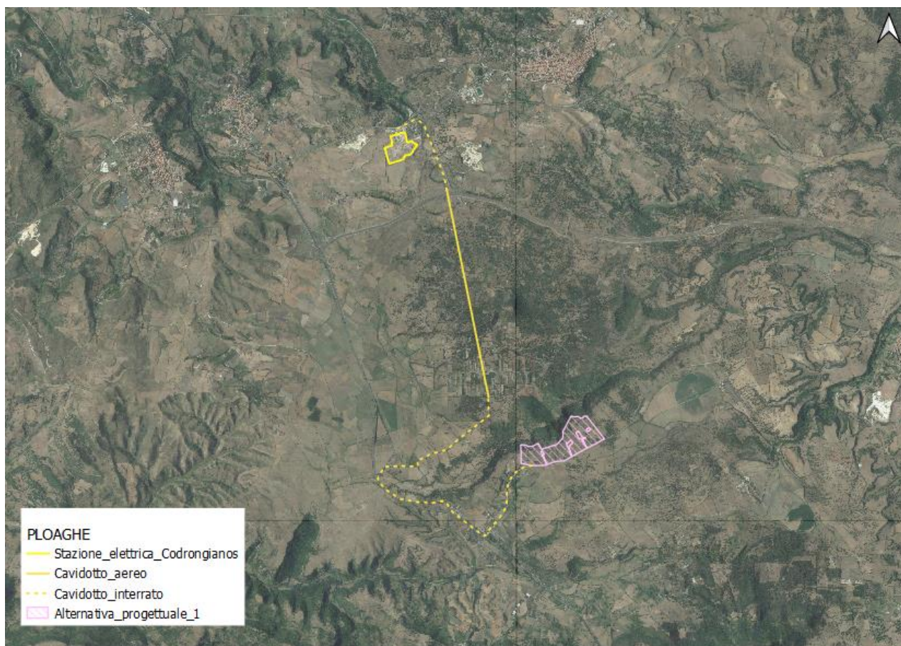
FIGURA 30 – ALTERNATIVA 1 DI IMPIANTO PER IL PROGETTO PLOAGHE
