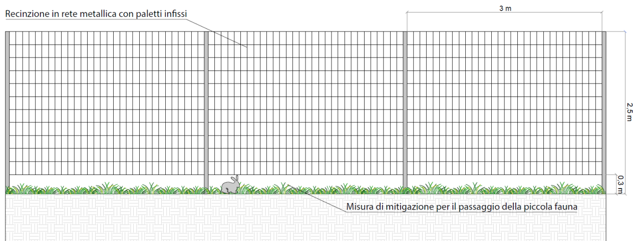
FIGURA 43 – ESEMPIO RECINZIONE METALLICA CHE DELIMITA L'AREA DI PERTINENZA DELL'IMPIANTO
