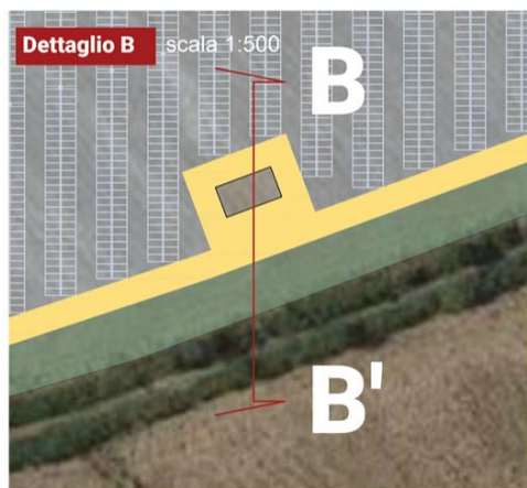
FIGURA 72 – PARTICOLARE FASCIA DI MITIGAZIONE CON VEGETAZIONE ESISTENTE E SEZIONE N-S DELL'IMPIANTO – ESTRATTO DALL'ELABORATO GRAFICO PLOAGHE-PDT11-R1) (IMMAGINE AGGIORNATA)
