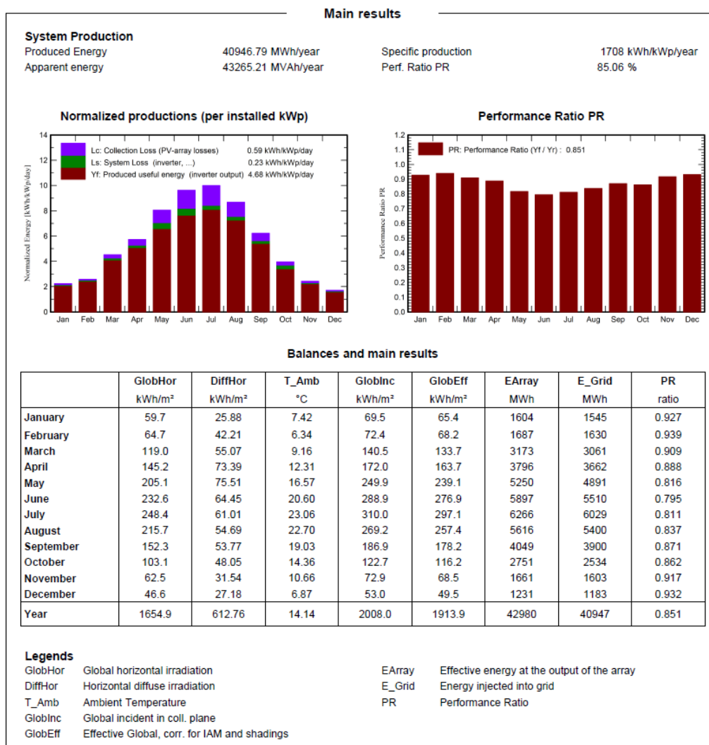
FIGURA 42 - PRODUCIBILITA' ELETTRICA DELL'IMPIANTO AGRIVOLTAICO VALUTATA TRAMITE PVSYST (IMMAGINE AGGIORNATA)
