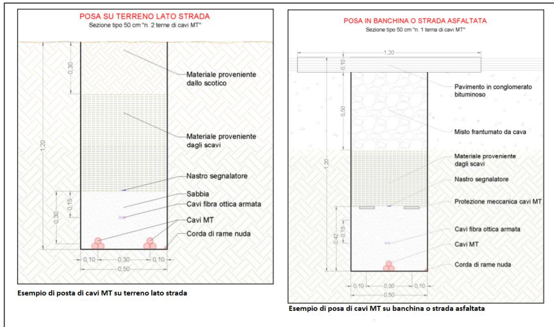
FIGURA 3: ESEMPIO TIPOLOGIA DI POSA PREVISTE ALL'INTERNO DEL SITO
