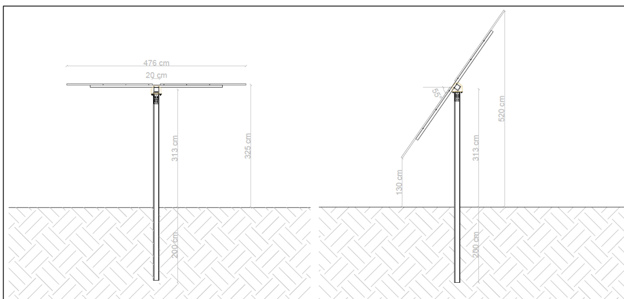
FIGURA 2 SCHEMA TIPO TRACKER AD ASSE VARIABILE
