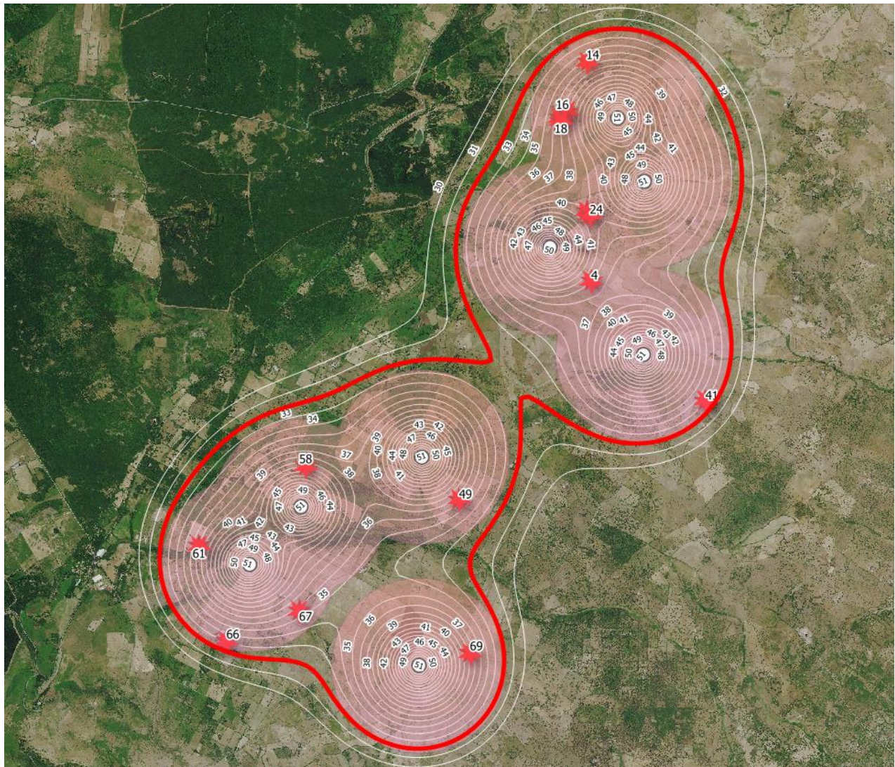
Figura 4.5 – Campo sonoro generato dall’impianto. In rosso l’isofonica dei 32 dBA, attestata ad una distanza indicativa di 1.000 m dalle postazioni eoliche in progetto
