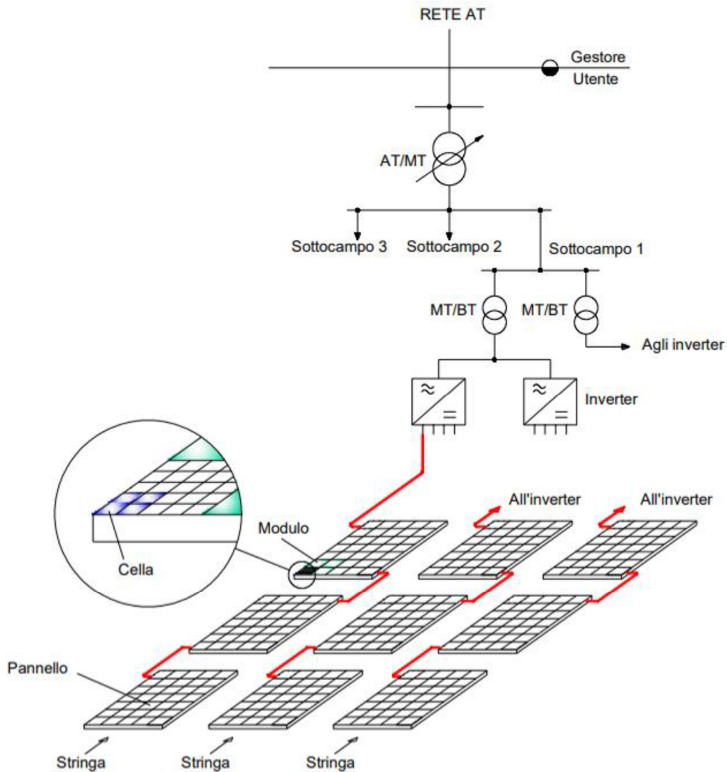
Immagine 4.7.1 Schema di impianto fotovoltaico.
