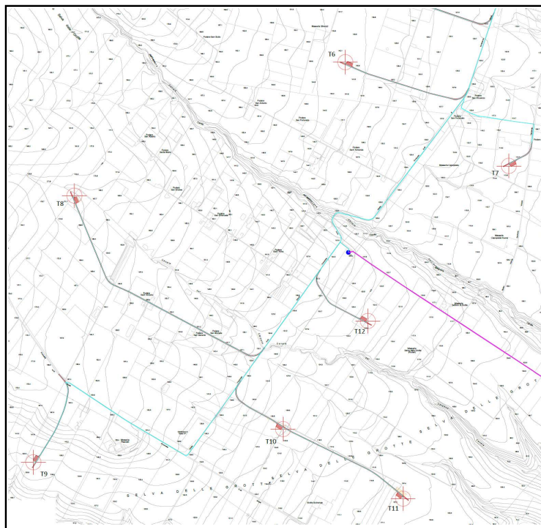
Figura 3.2 – Layout Impianto su CTR
