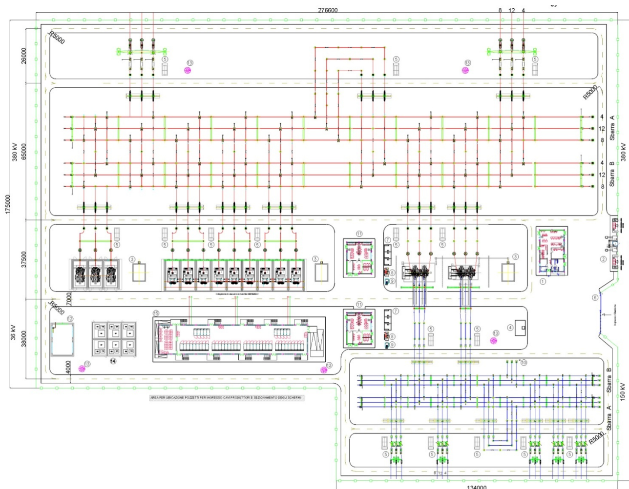
Figura 12 - Stazione Elettrica RTN 380/36 kV
