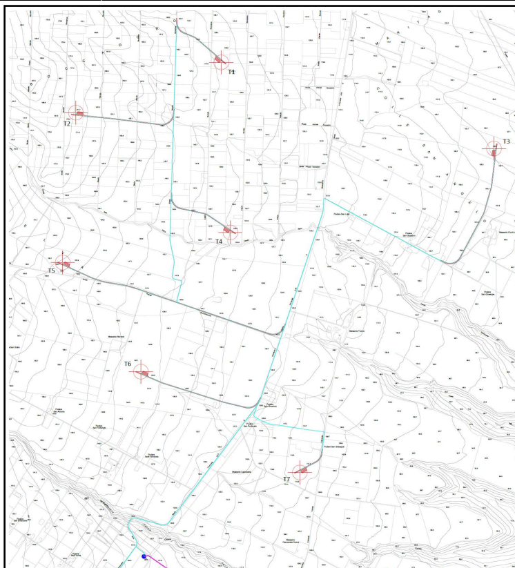
Figura 3.1 – Layout Impianto su CTR
