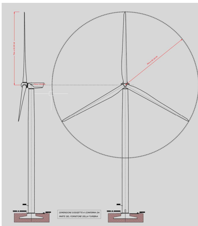
Figura 4 – Caratteristiche aerogeneratore tipo
