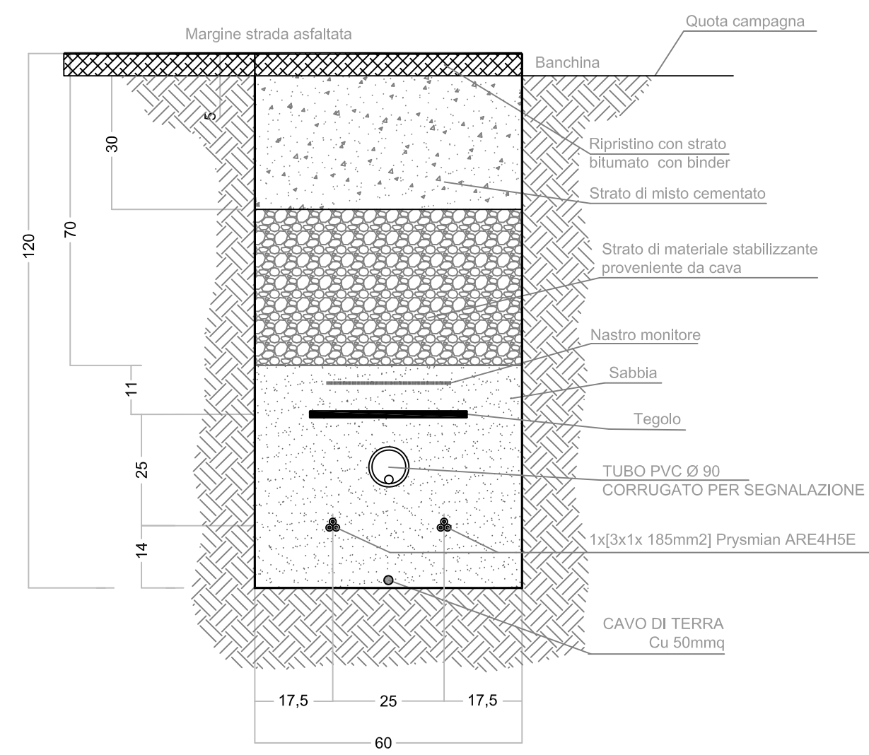
Sezione tipo doppia terna lungo strada asfaltata
