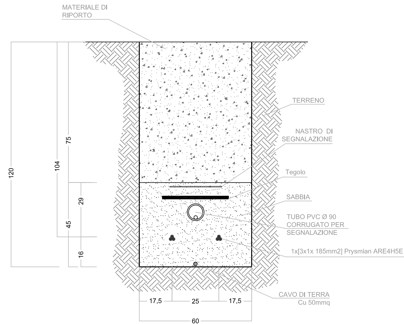
Sezione tipo doppia terna in terreno vegetale
