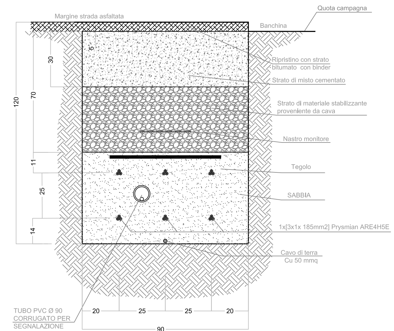
Sezione tipo sei terne lungo strada asfaltata
