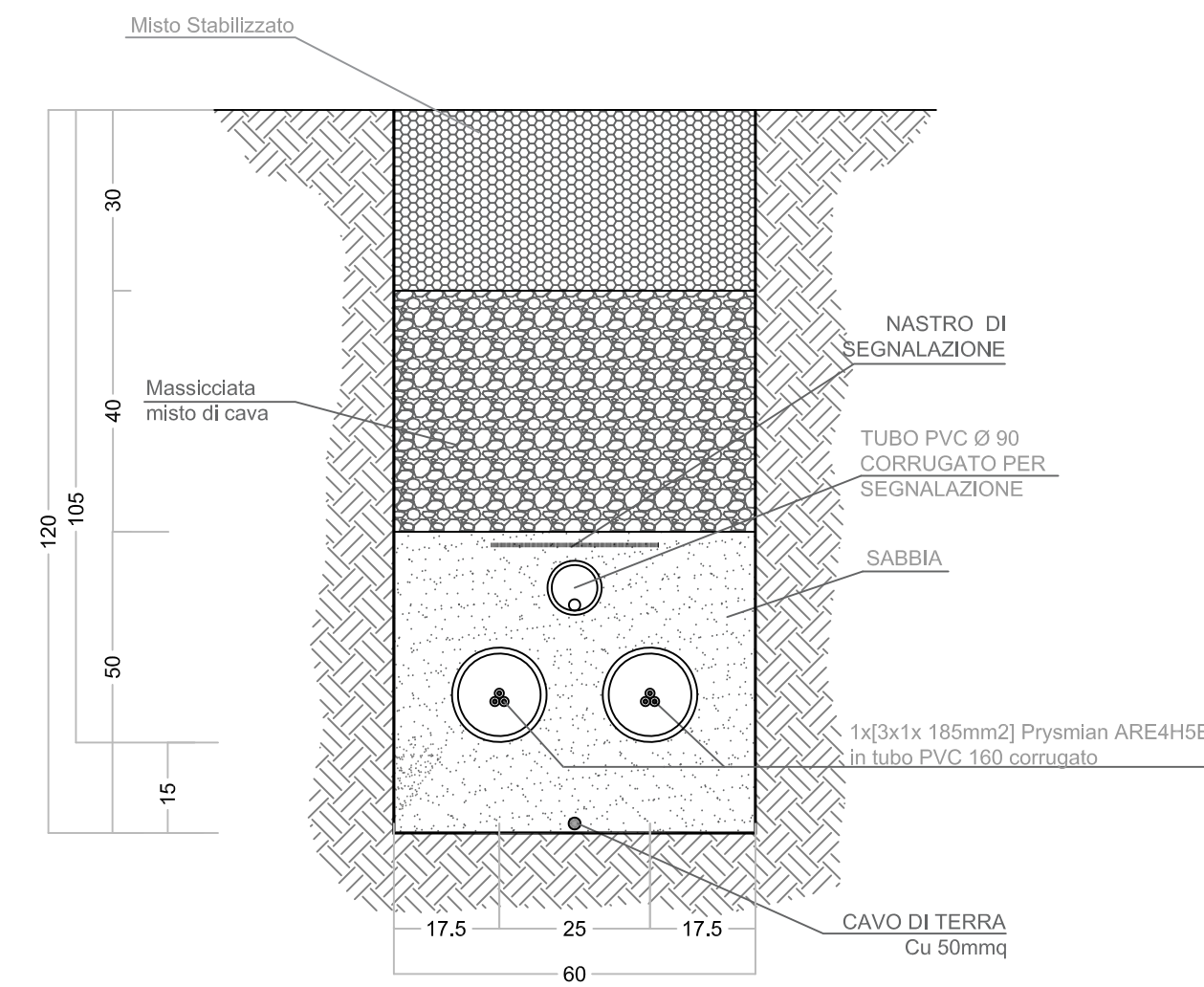
Sezione tipo doppia terna lungo asse di nuova formazione
