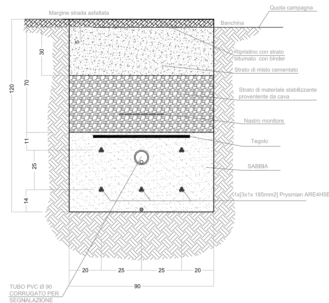
Sezione tipo cinque terne lungo strada asfaltata
