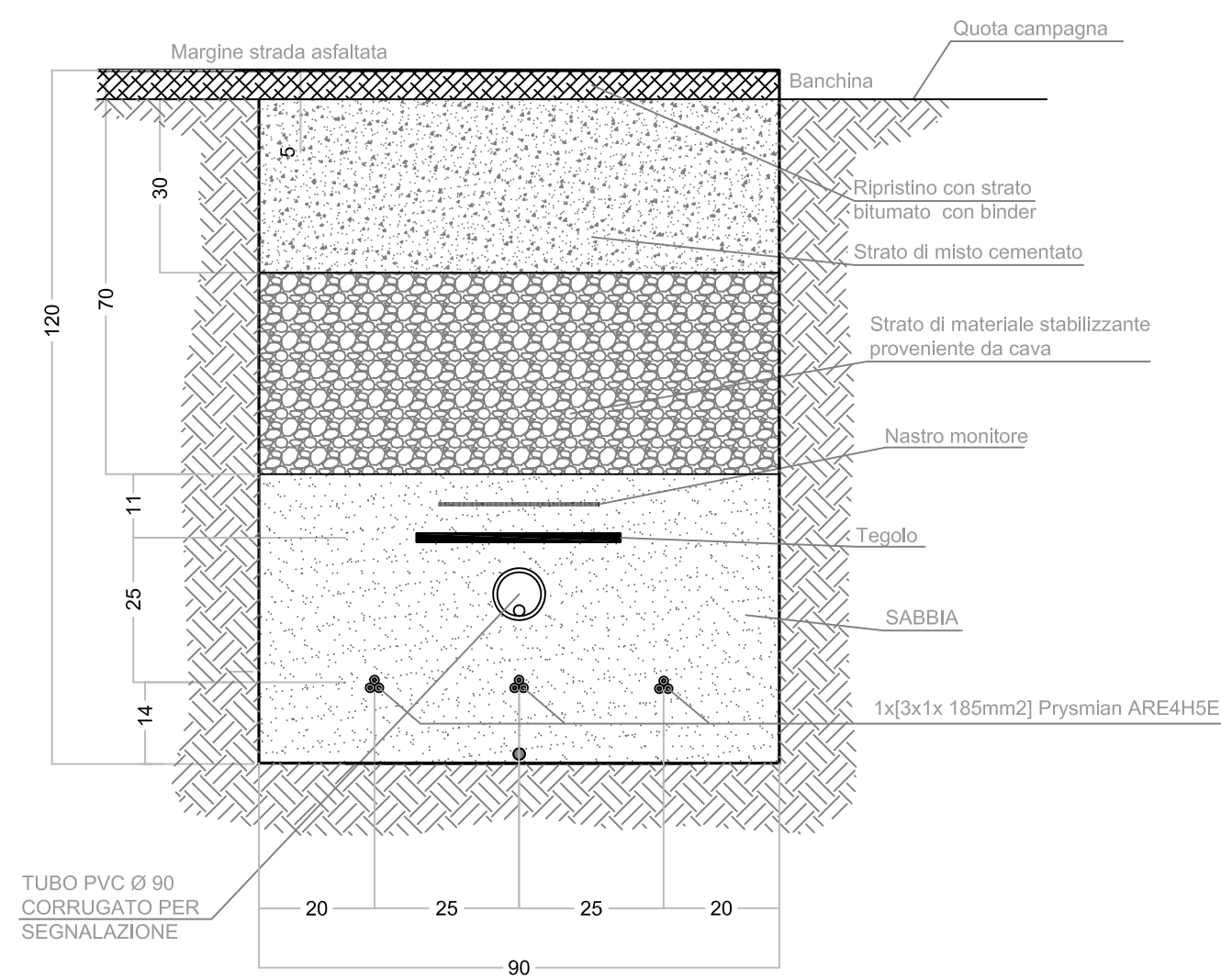
Sezione tipo tre terne lungo strada asfaltata
