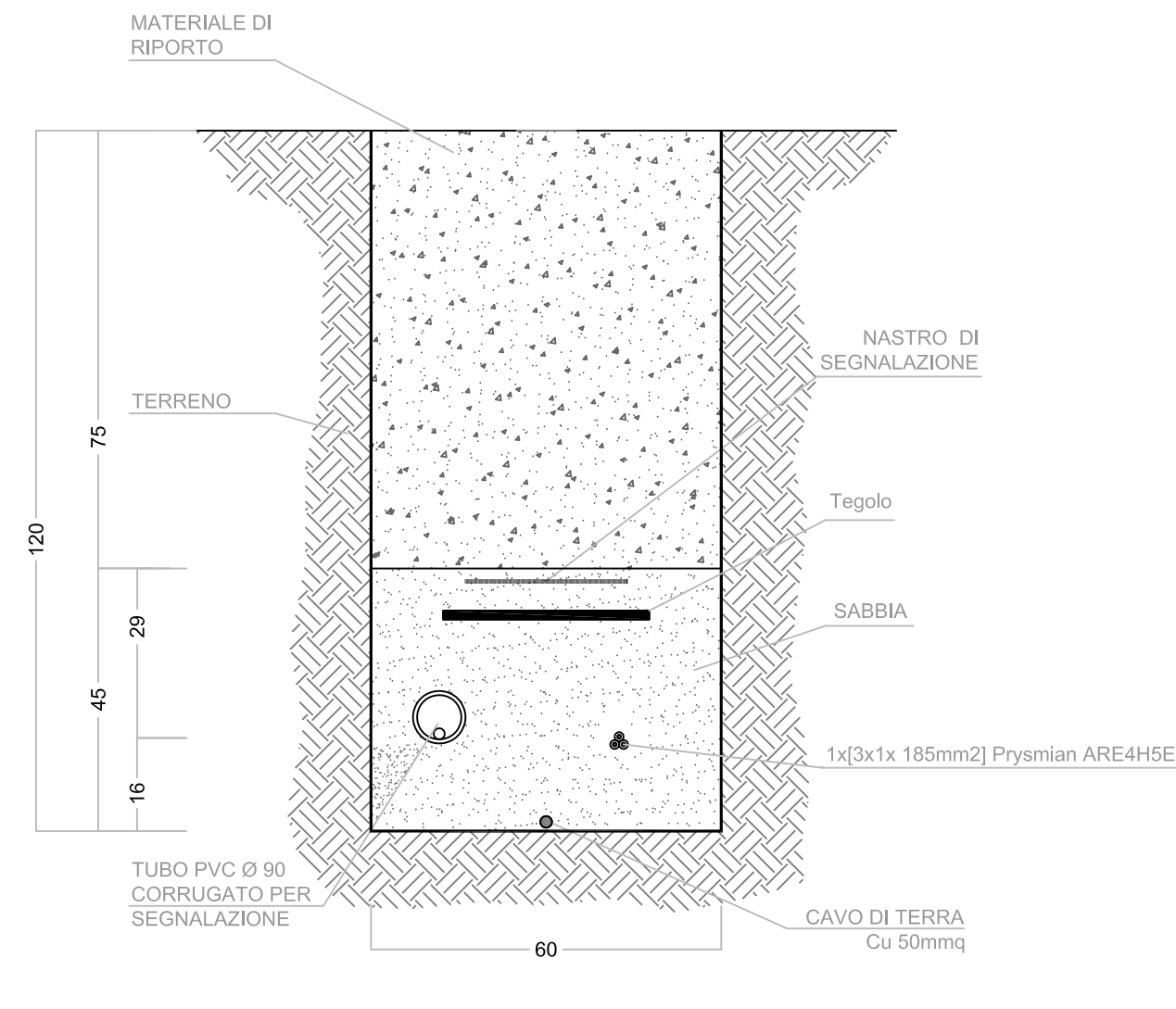
Sezione tipo singola terna in terreno vegetale
