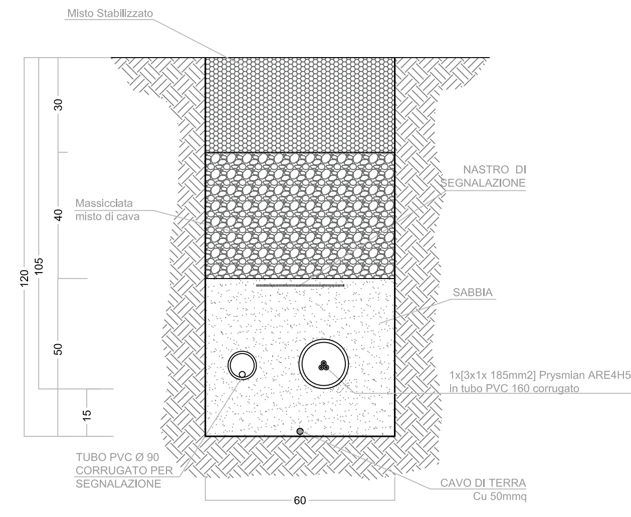
Sezione tipo singola terna lungo asse di nuova formazione
