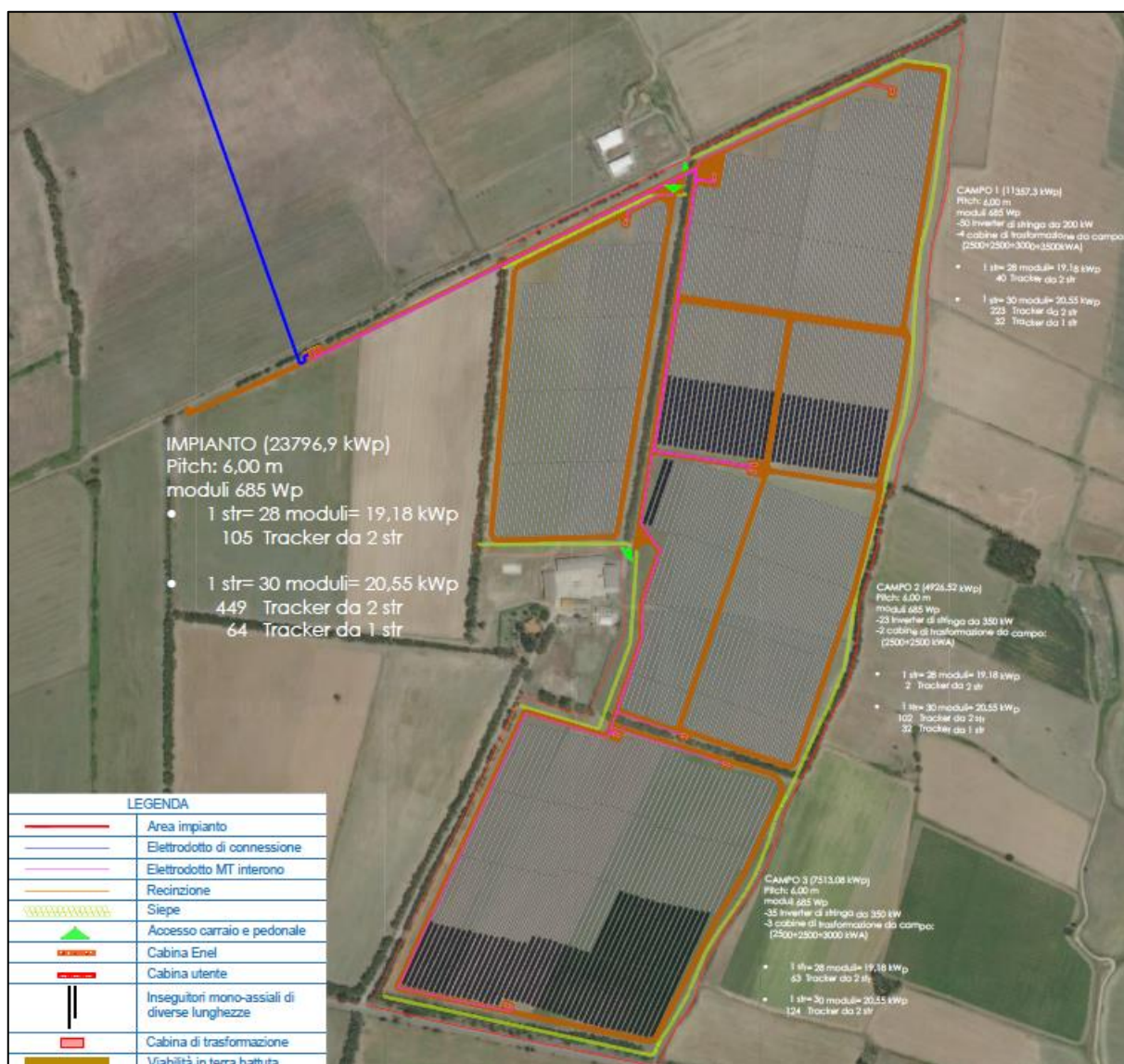
Fig. 7: Layout dell'impianto Agrovoltaico San Vero Milis
