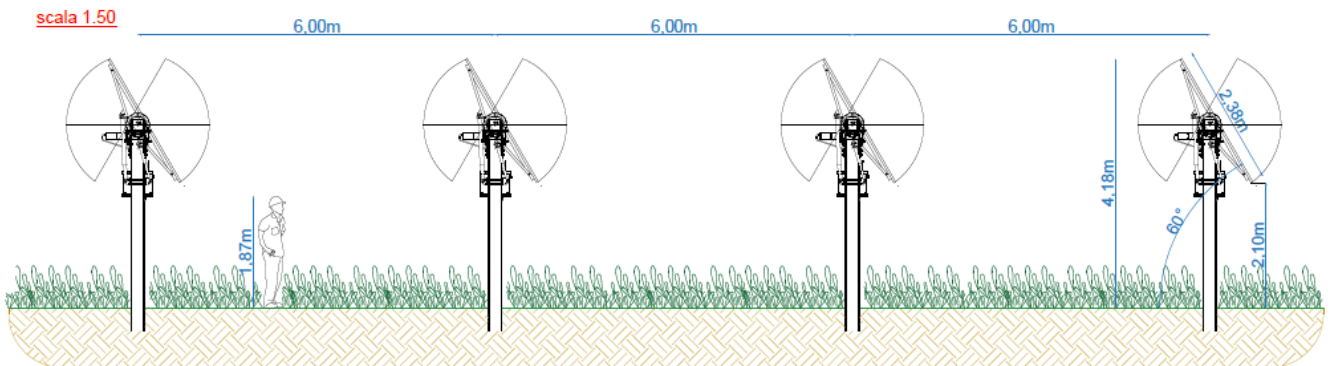
Fig. 9: Vista trasversale del sesto d'impianto fotovoltaico
