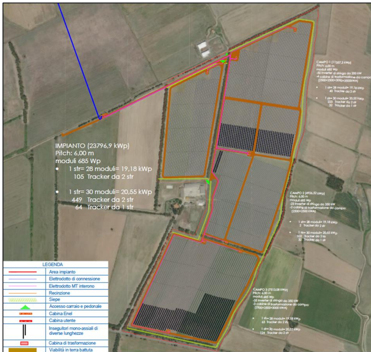
Fig. 1: layout dell'impianto Agrovoltaico San Vero Milis
