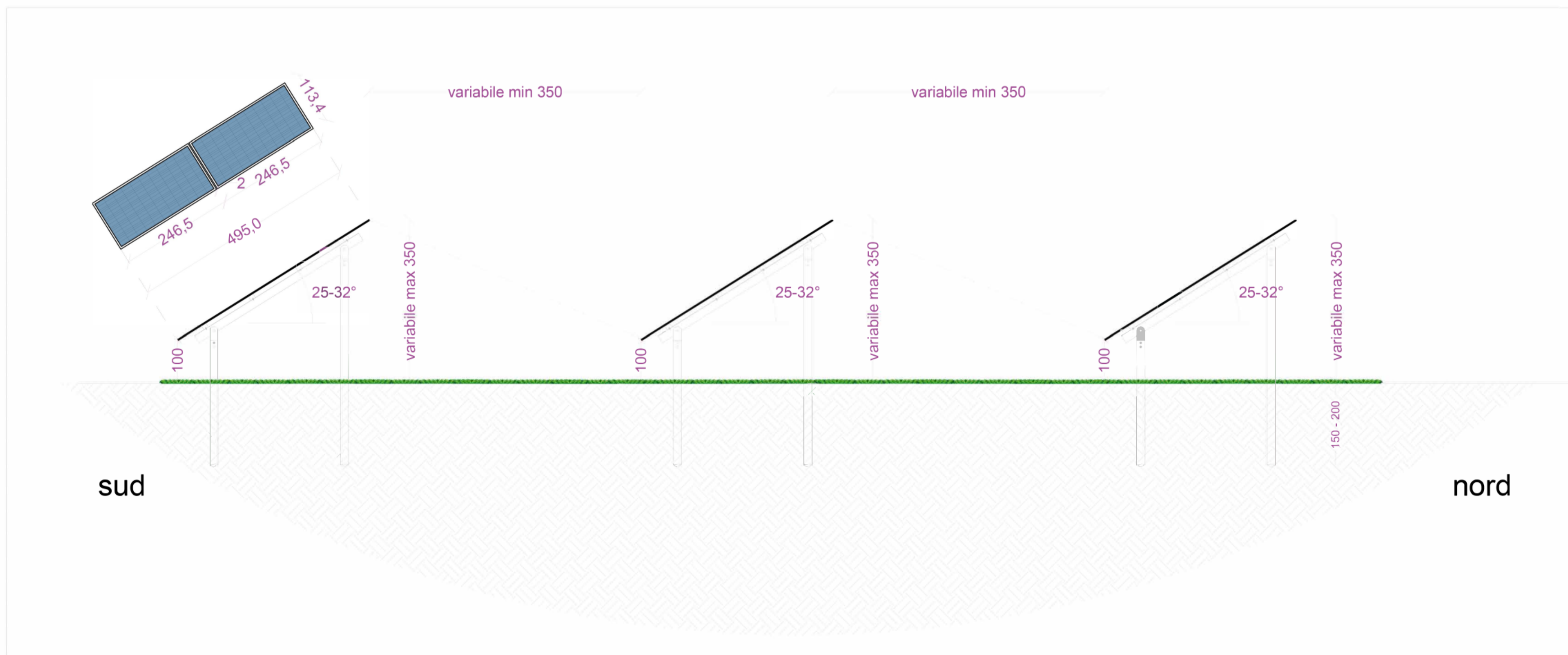
SCHEMA DI SEZIONE TIPO DISPOSIZIONE FILARI NELLA CONFIGURAZIONE FISSA - SCALA 1:50
