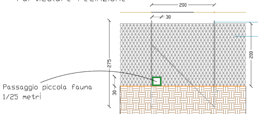
Figura 7: Particolare recinzione d'impianto (fuori scala).
