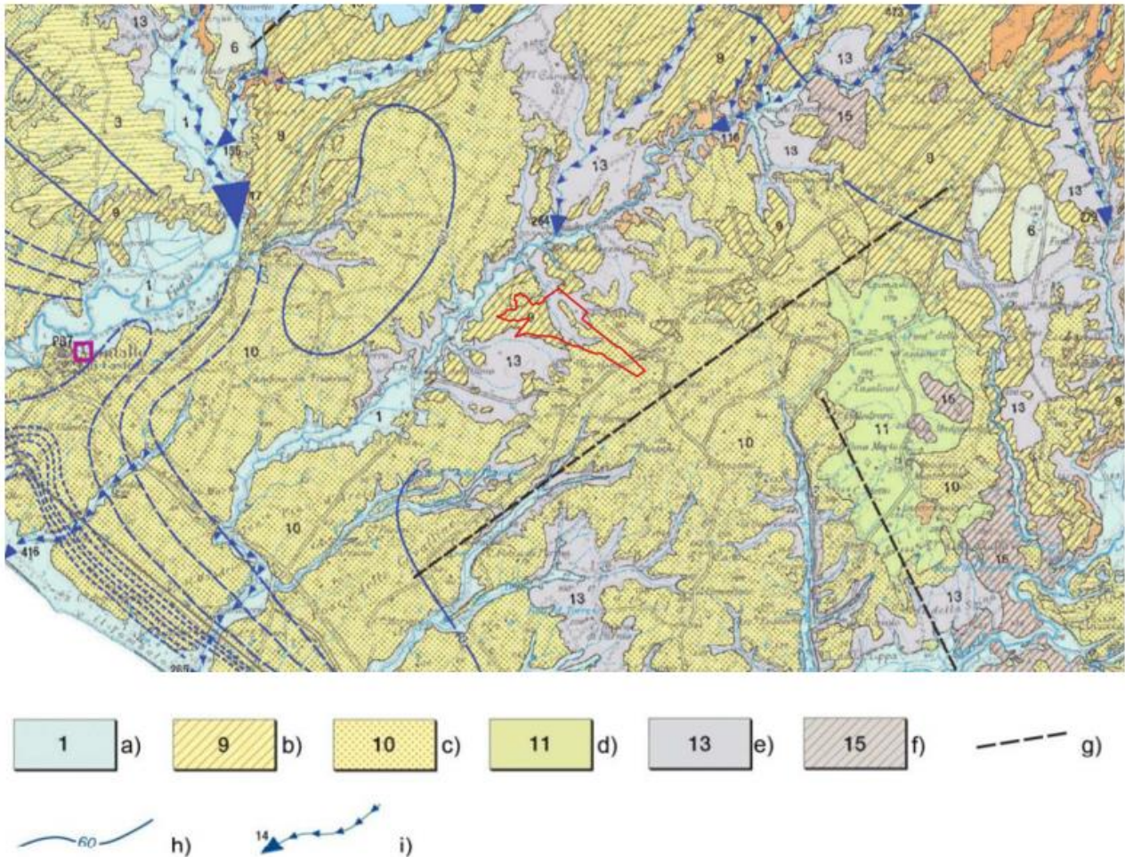
Figure 10 - Stralcio della Carta Idrogeologica del Territorio della Regione Lazio (2012), modificato. In rosso l'ubicazione dell'area di studio.
