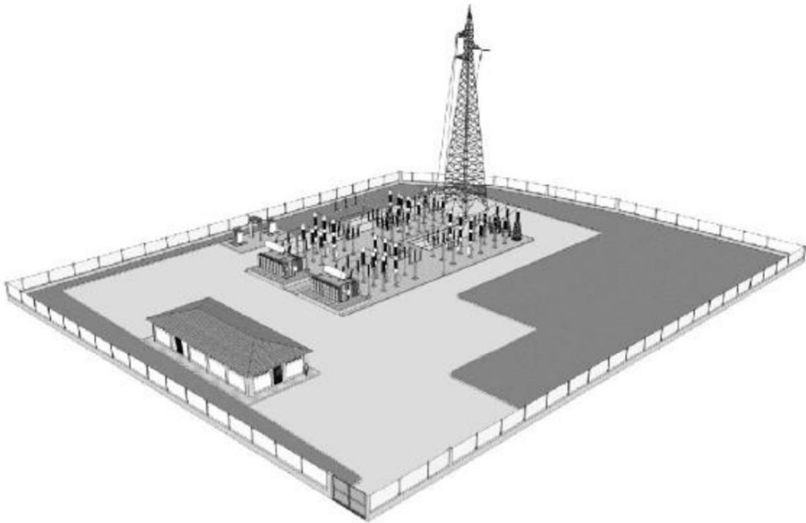
Fig. 3a: Rappresentazione di una tipica Stazione di Utenza 150/30 kV con apparecchiature isolate in aria
