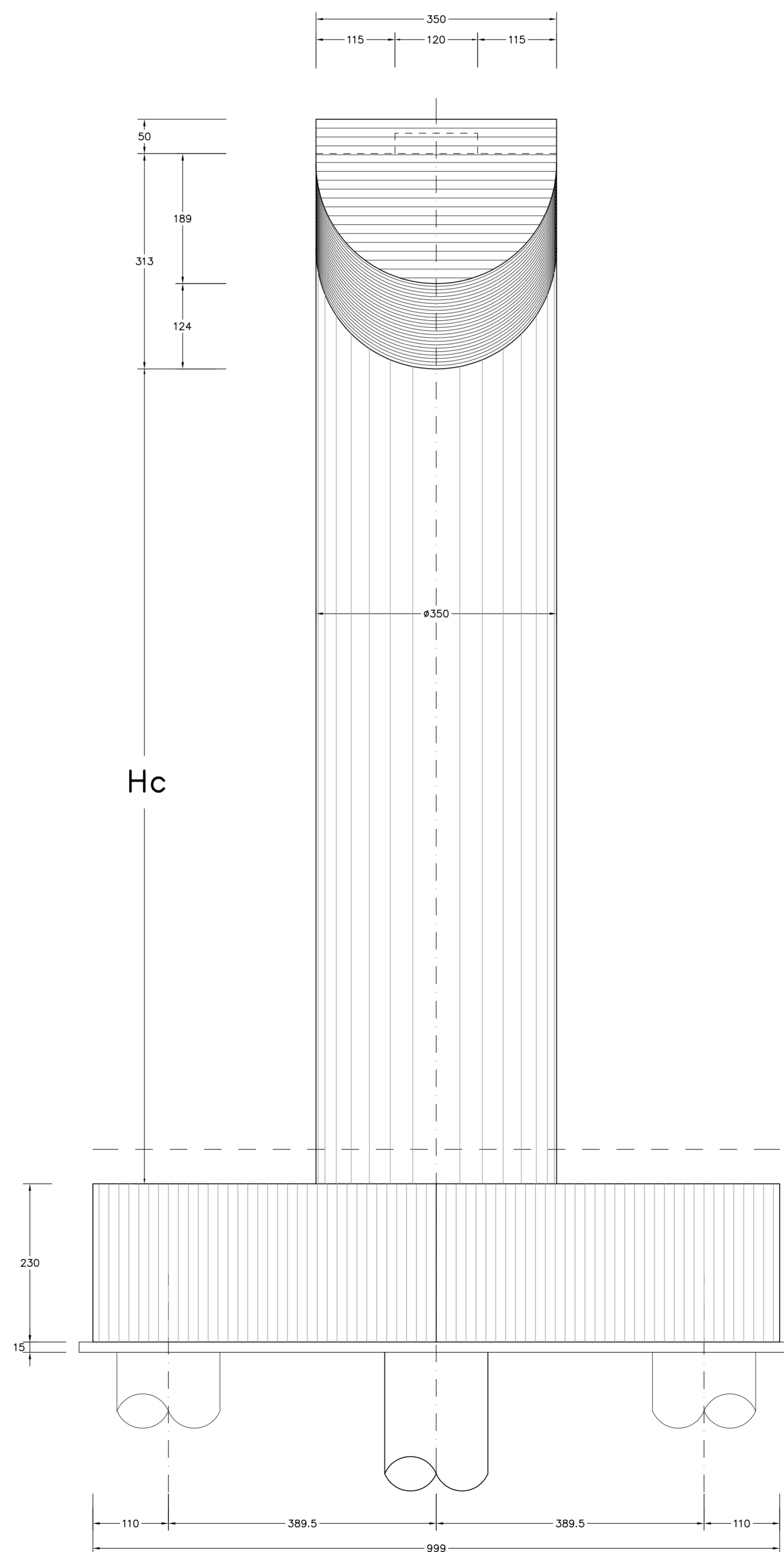
VISTA LATERALE B-B SCALA 1:50
