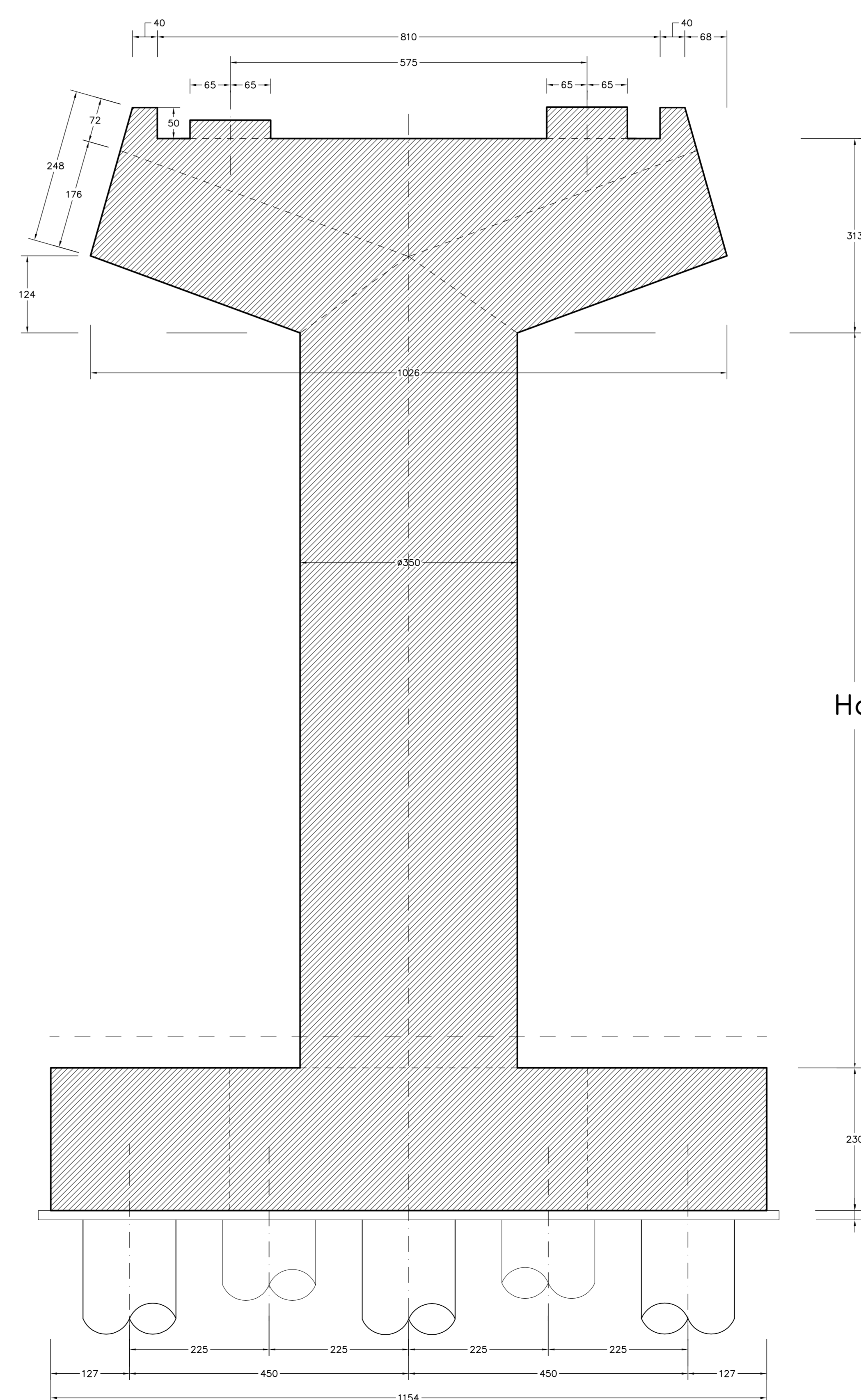
SEZIONE TRASVERSALE SCALA 1:50
