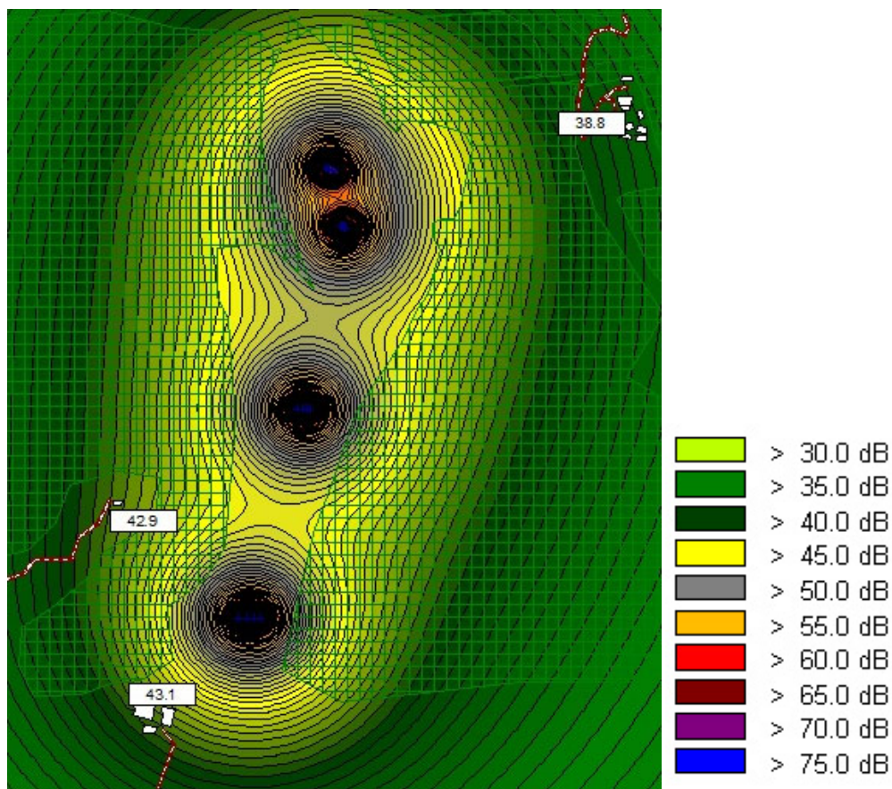
Fig. 6 – Scenario acustico previsionale ai ricettori Sottocampo 1 e 2
