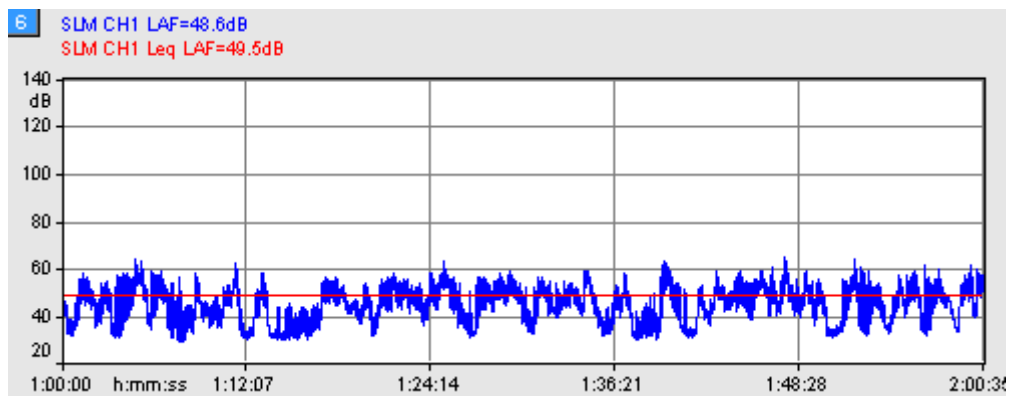
Graf.3 – Rilievi rumore residuo al ricevitore R2=48,6 dB
