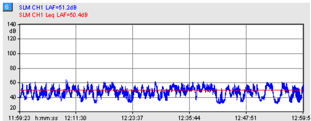
Graf.3 – Rilievi rumore residuo al ricevitore R3=50,4 dB
