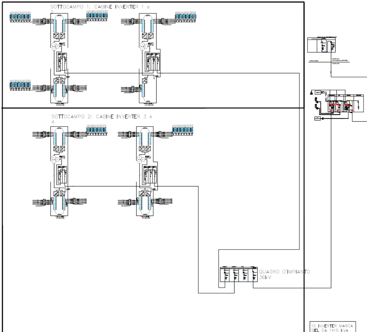
Figura 3 – Schema Elettrico Unifilare
