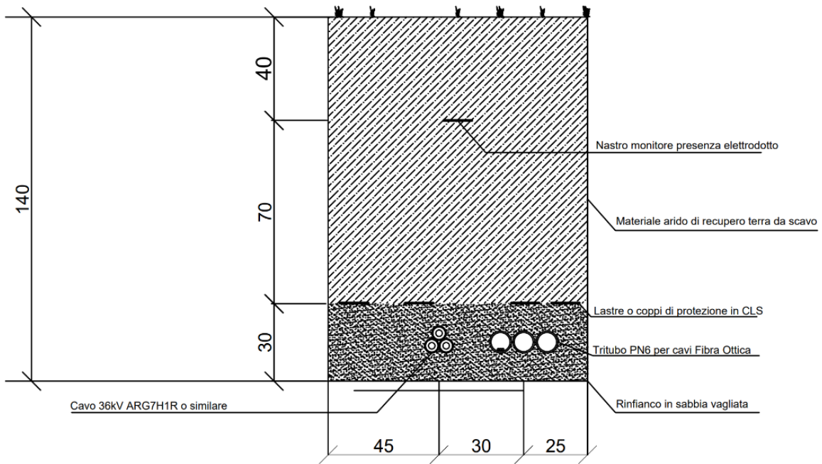
Figura 6 – Sezione tipo su terreno vegetale
