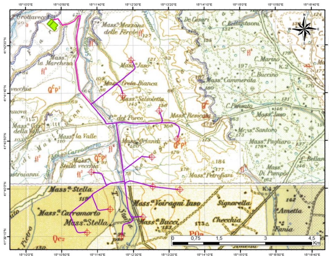
Figura 1 – Stralcio della Carta Geologica d'Italia
