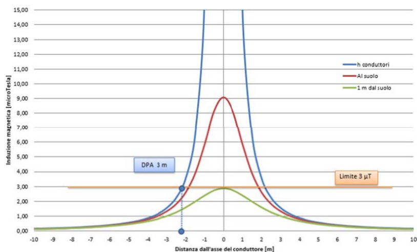
Figura 9: Andamento del campo magnetico in funzione della distanza dall’asse dei conduttori relativa alla simulazione S5
