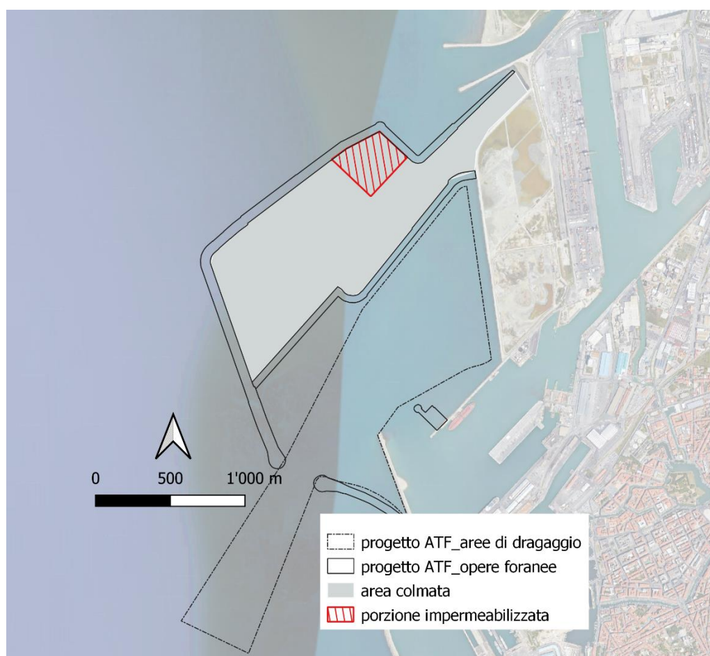
Figura 29: rappresentazione del layout di progetto con indicazione dell'area conterminata (area di Colmata) dove verranno collocati i sedimenti
