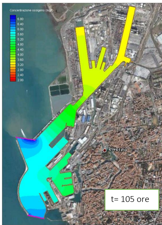
Figura 3.5 – Configurazione attuale con la sola forzante di marea (concentrazione dell'ossigeno disciolto t=105 ore - valori in mg/l).
