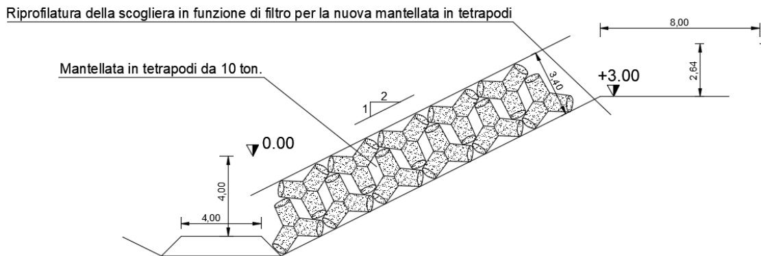
Figura 46 WBS 7 – Progetto 2005 – realizzazione mantellata in tetrapodi / tipologico.
