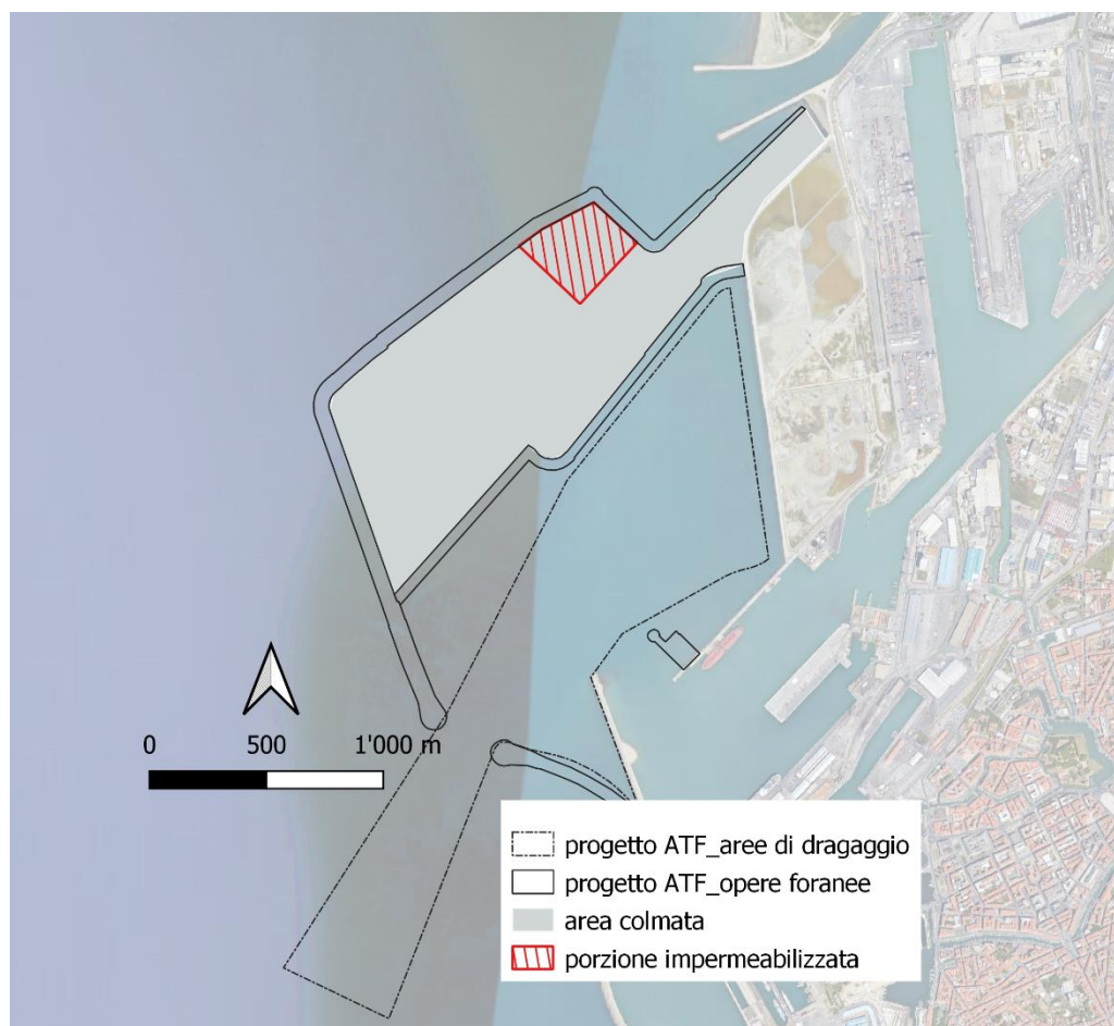
Figura 39: rappresentazione del layout di progetto con indicazione dell'area conterminata (area di Colmata) dove verranno collocati i sedimenti
