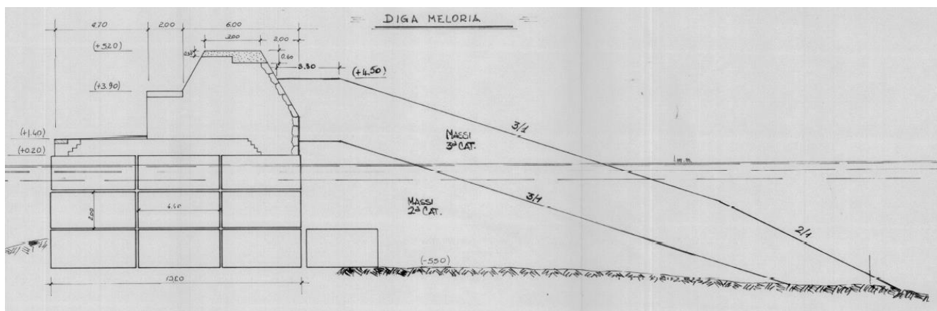
Figura 45 WBS 7 – Progetto 1994 / ripristino mantellata esterna – sezione tipologica.
