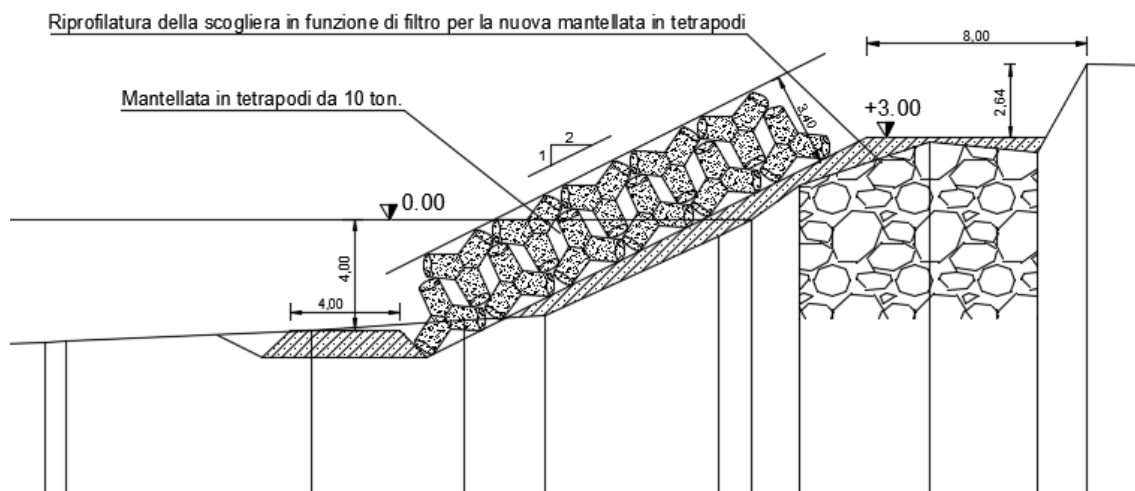
Figura 47 WBS 7 – Progetto 2005 – realizzazione mantellata in tetrapodi / prog. 199.973
