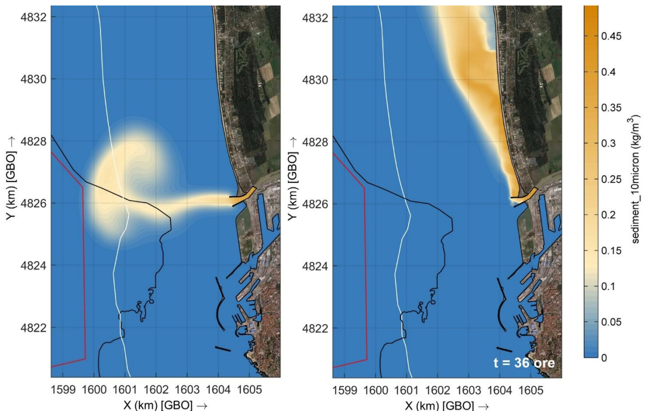
Figura 18 Concentrazione dei sedimenti fluviali coesivi durante la piena dello Scolmatore d'Arno (mareggiata di Ponente, Q = 414 \text{ m}^3/\text{s} , C_{\text{sed}} = 0.5 \text{ kg}/\text{m}^3 ) – condizioni di calma (sinistra) e con mareggiata di Ponente (destra)
