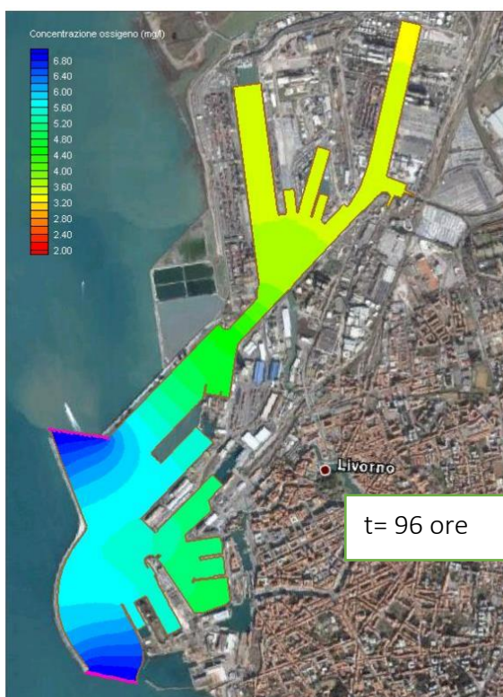
Figura 3.2 – Configurazione attuale con la sola forzante di marea (concentrazione dell'ossigeno disciolto t=96 ore - valori in mg/l).
