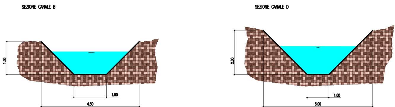
Figura 8: Sezioni canali di progetto
