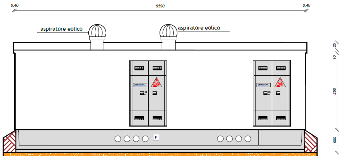
Planimetria cabina di raccolta – sezione
