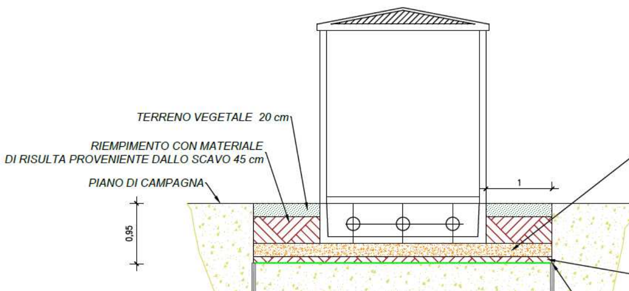
Cabina di raccolta – sezione sito di installazione
