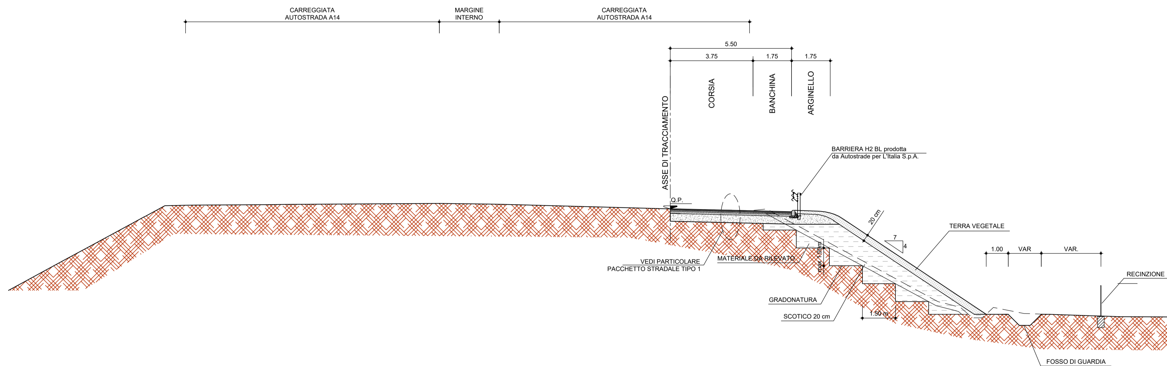
PACCHETTO STRADALE TIPO 1 scala 1:10
