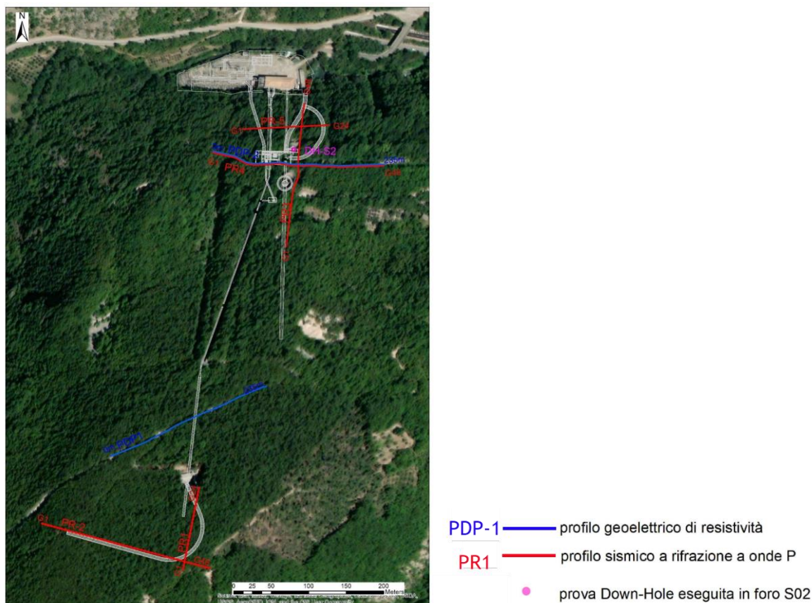
Figura 8: Ubicazione delle linee sismiche e geoelettriche (da: Pietrangeli, 2022) [45], con legenda aggiunta
