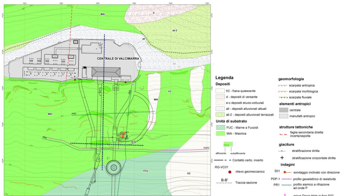
Figura 17: Mappa geologica geomorfologica di dettaglio – Area di Centrale.
