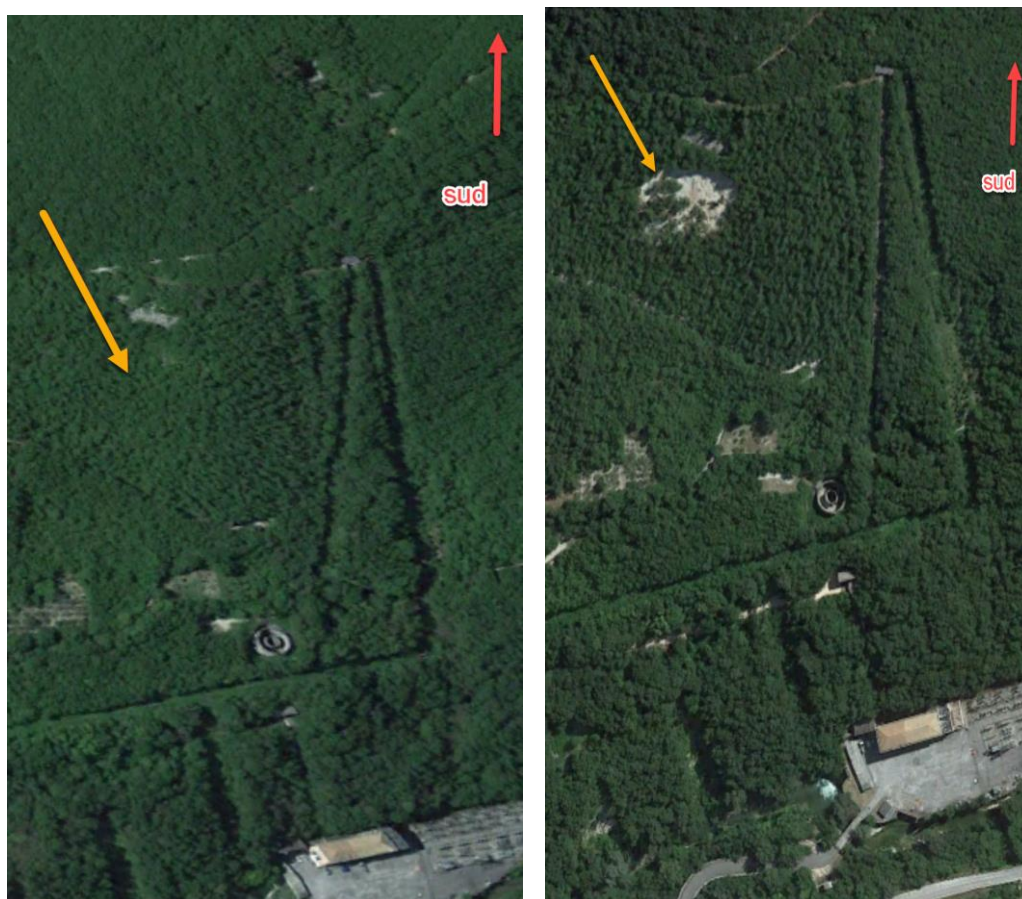
Figura 15: Sviluppo della frana situata sul versante ad est delle opere esistenti. A sinistra lo stato nel maggio 2016, a destra nell'agosto 2017.
