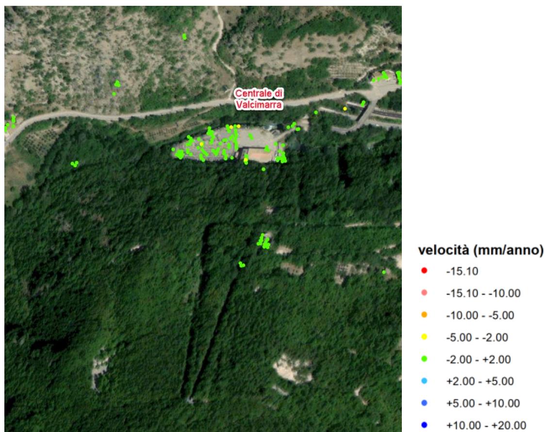
Figura 13: Permanent Scatterers relativi al monitoraggio InSar – Ministero dell’Ambiente. Le velocità sono espresse in mm/anno.
