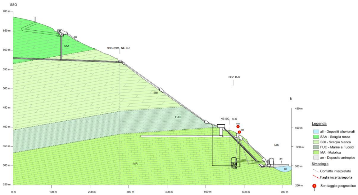
Figura 18: Sezione geologica generale lungo il versante.
