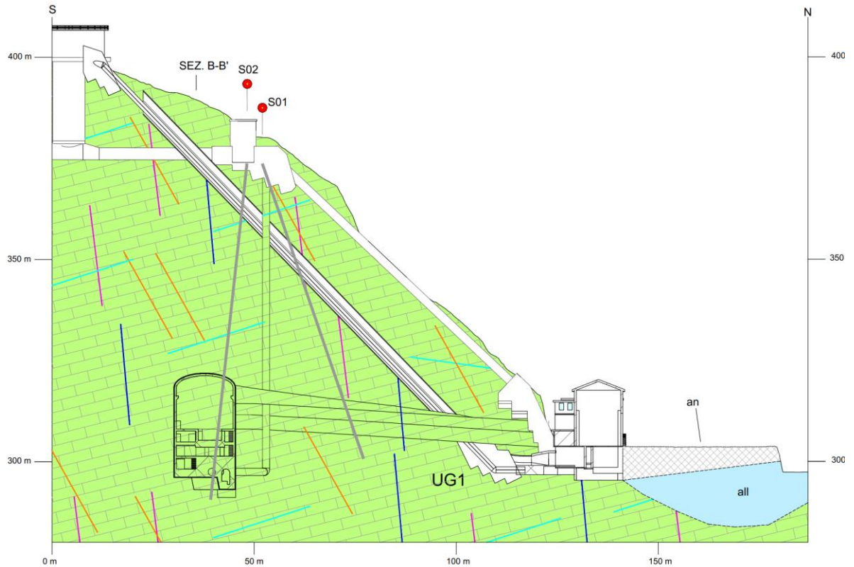
Figura 20: Sezione geologico-geotecnica trasversale lungo la centrale in progetto
