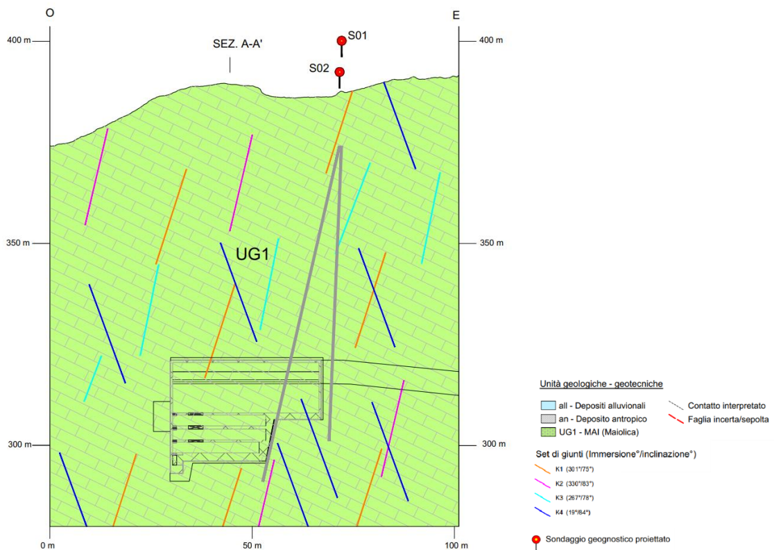
Figura 19: Sezione geologico-geotecnica longitudinale lungo la centrale in progetto.
