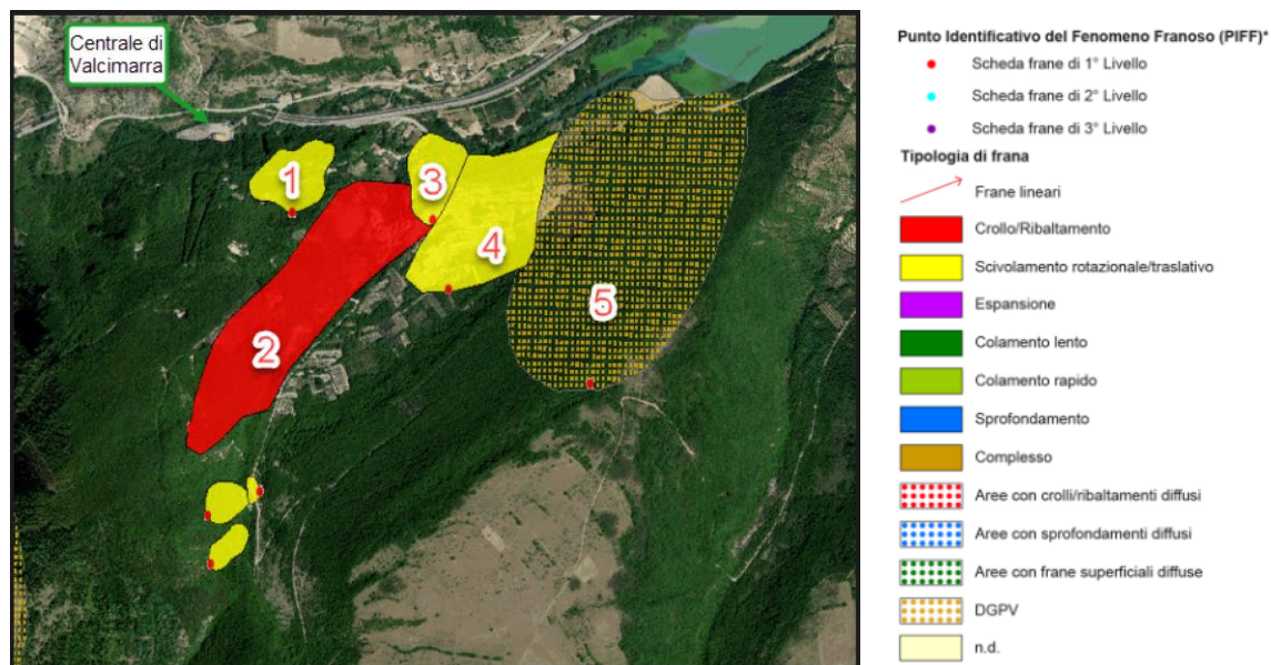
Figura 11: Stralcio della Carta Inventario dei Fenomeni Franosi Progetto IFFI (da ISPRA) [20]. In figura i dissesti presenti nella BD sono numerati come in tabella Tabella 2 ed è indicata la posizione della Centrale di Valcimarra
