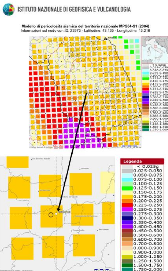
Figura 31: Accelerazione massima al suolo (PGA) con probabilità di eccedenza del 10% in 50 anni (Fonte INGV [29]).
