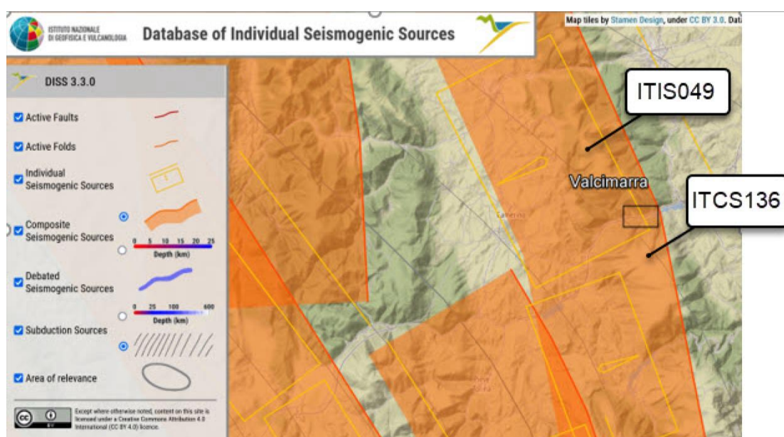
Figura 28: Estratto mappa DISS versione 3.3 – INGV. Catalogo zone sismogenetiche [30] Nel riquadro nero la zona di studio
