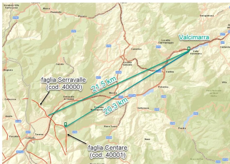
Figura 27: Estratto mappa ITHACA - Catalogo faglie capaci [32] (ridisegnato)
