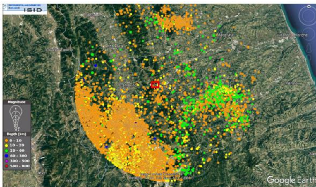
Figura 26: Distribuzione dei terremoti localizzati in tempo reale dall'INGV Centro Nazionale dei Terremoti in un raggio di 30 km dalla Centrale di Valcimarra, in rosso (data base Centro Nazionale Terremoti dati al 08/04/2022).
