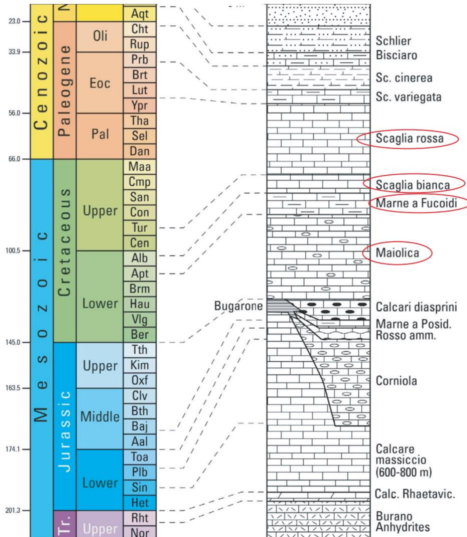
Figura 10: Stralcio della colonna stratigrafica dell’Appennino umbro-marchigiano ([24] ridisegnato). In rosso le formazioni presenti nella zona della centrale e nei suoi dintorni.
