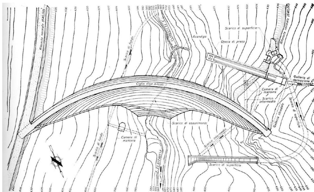
Figura 10: diga del Fiastrone – planimetria generale
