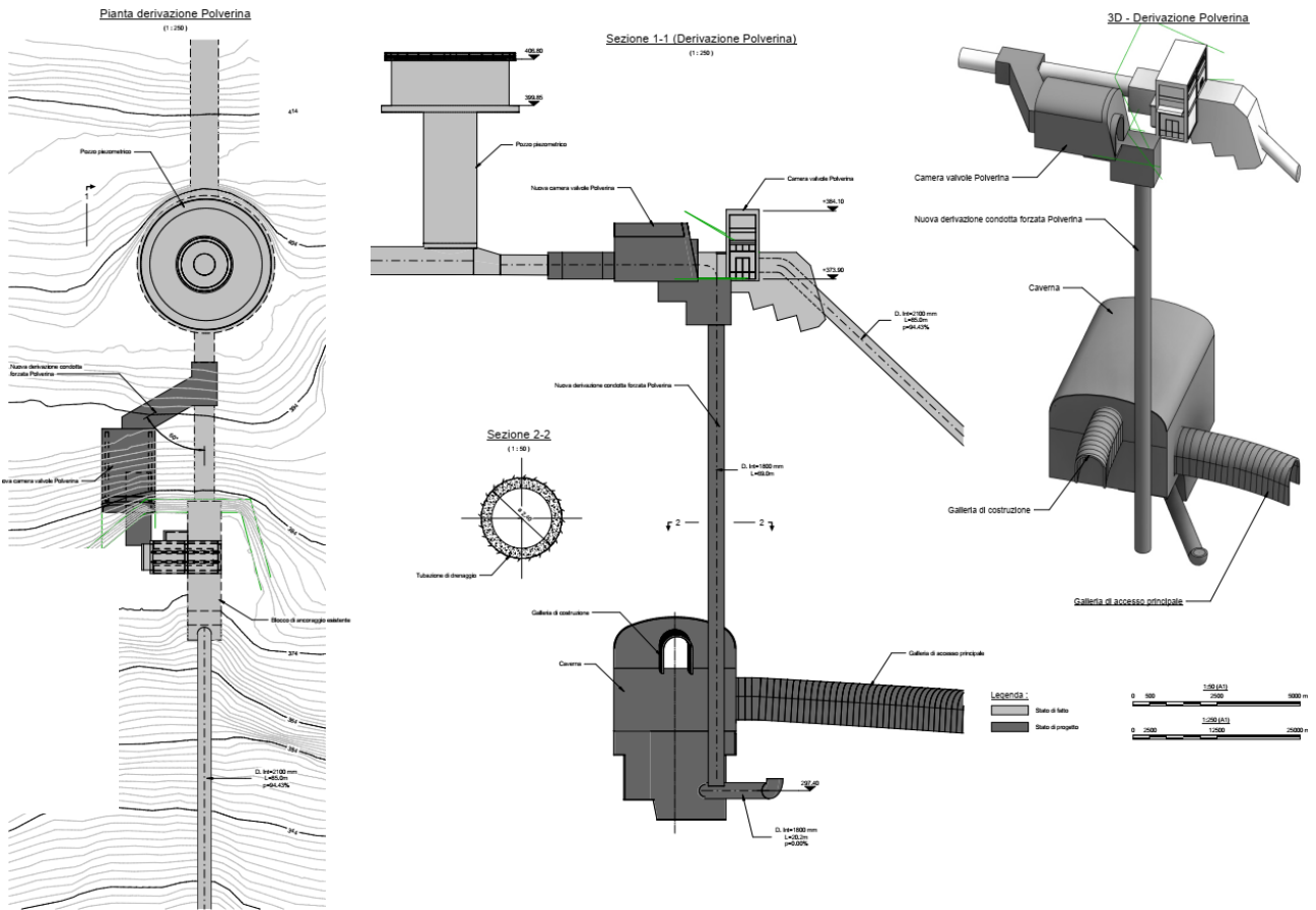
Figura 29: ampliamento C.V. Polverina e nuovo ramo C.F.
