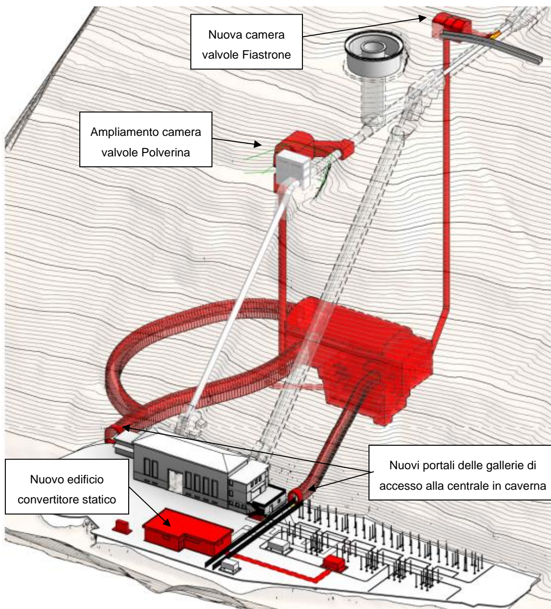
Figura 64: comparativo prospetto-versante e centrale. In rosso le nuove costruzioni, in giallo le demolizioni
