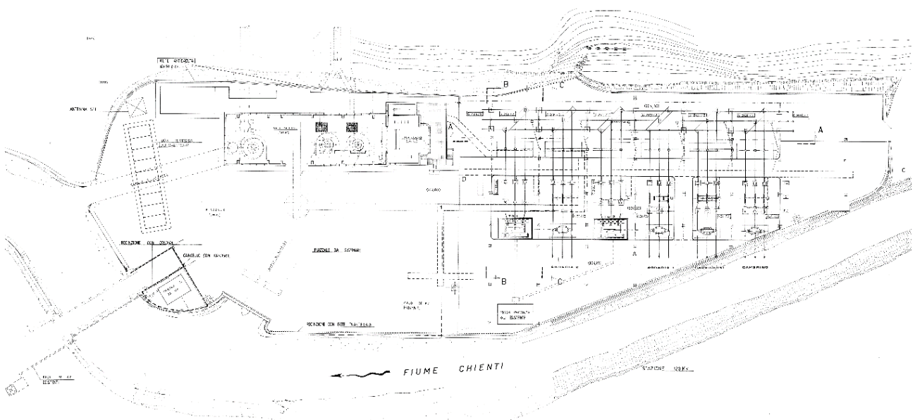
Figura 20: centrale di Valcimarra – Planimetria generale
