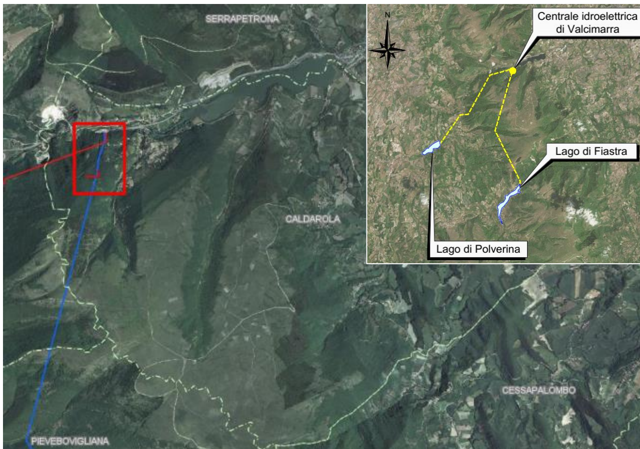
Figura 1: nel rettangolo rosso l'area interessata dal progetto nel Comune di Caldarola. In alto a destra l'inquadramento generale con indicazione degli esistenti serbatoi.
