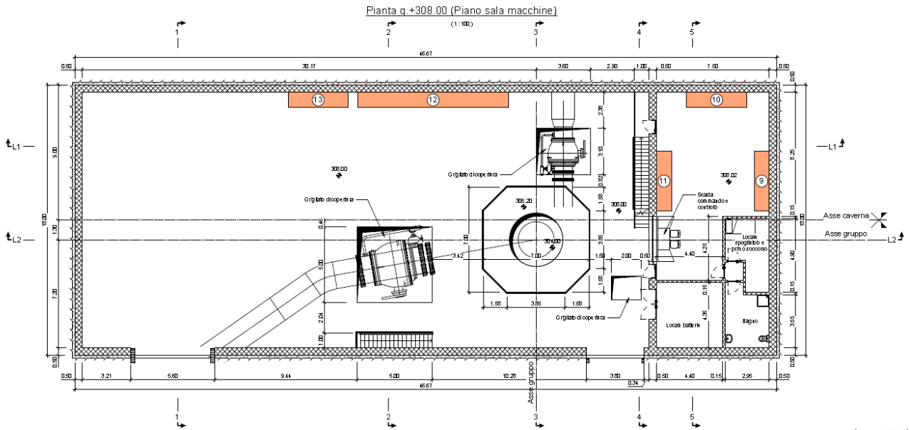
Figura 25: centrale di Valcimarra II – piano sala macchine
