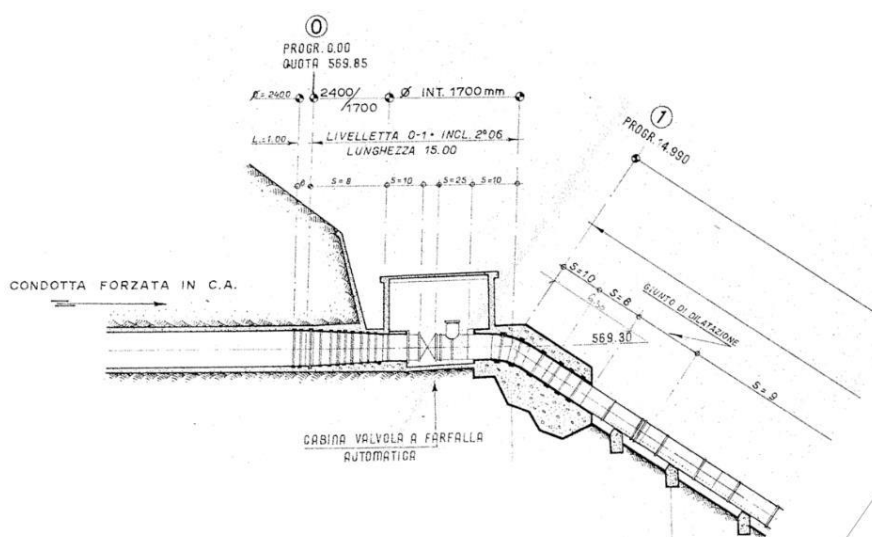
Figura 12: derivazione Fiastrone – camera valvole
