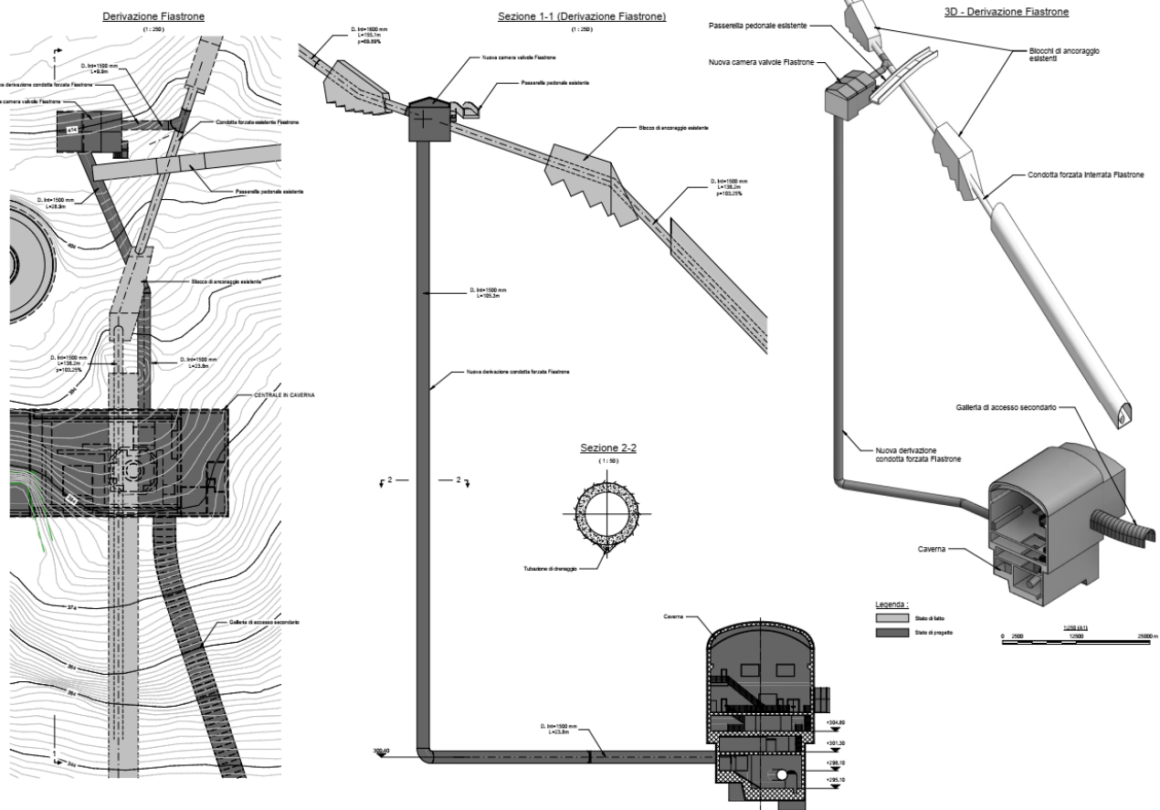
Figura 30: nuova C.V. Fiastrone e nuovo ramo C.F.
