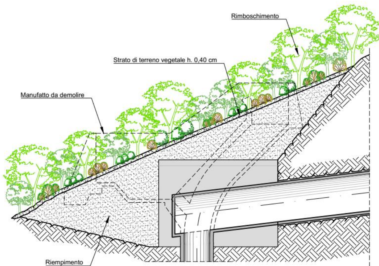
Figura 104: Sezione in corrispondenza del rimboschimento
