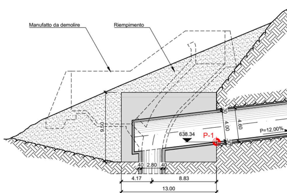
Figura 71: sezione longitudinale vasca di espansione da demolire
