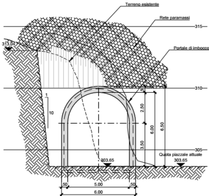
Figura 66: vista frontale imbocco galleria principale
