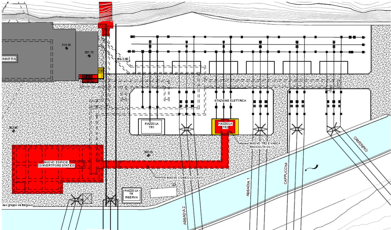
Figura 33: opere in sottostazione
