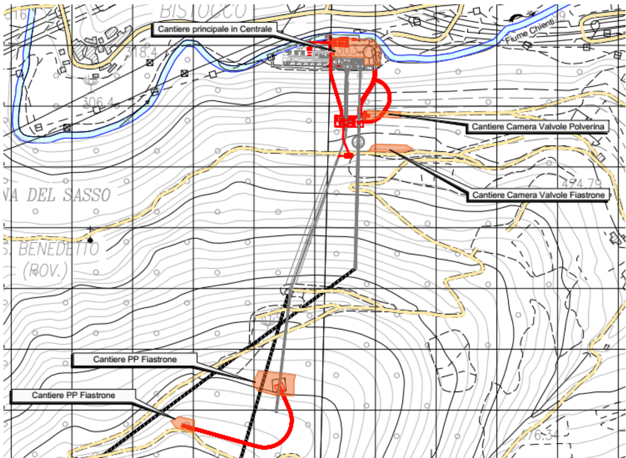
Figura 35: dettaglio ubicazione aree di cantiere
