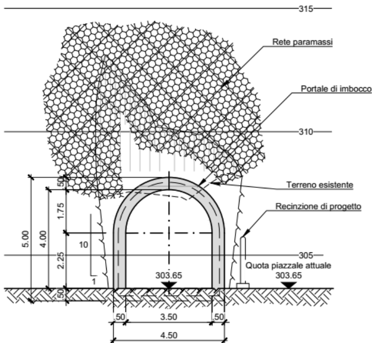
Figura 67: vista frontale imbocco galleria secondaria
