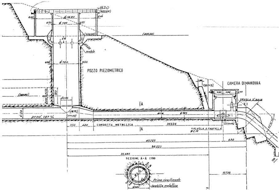
Figura 19: derivazione di Polverina – pozzo piezometrico e camera valvole
