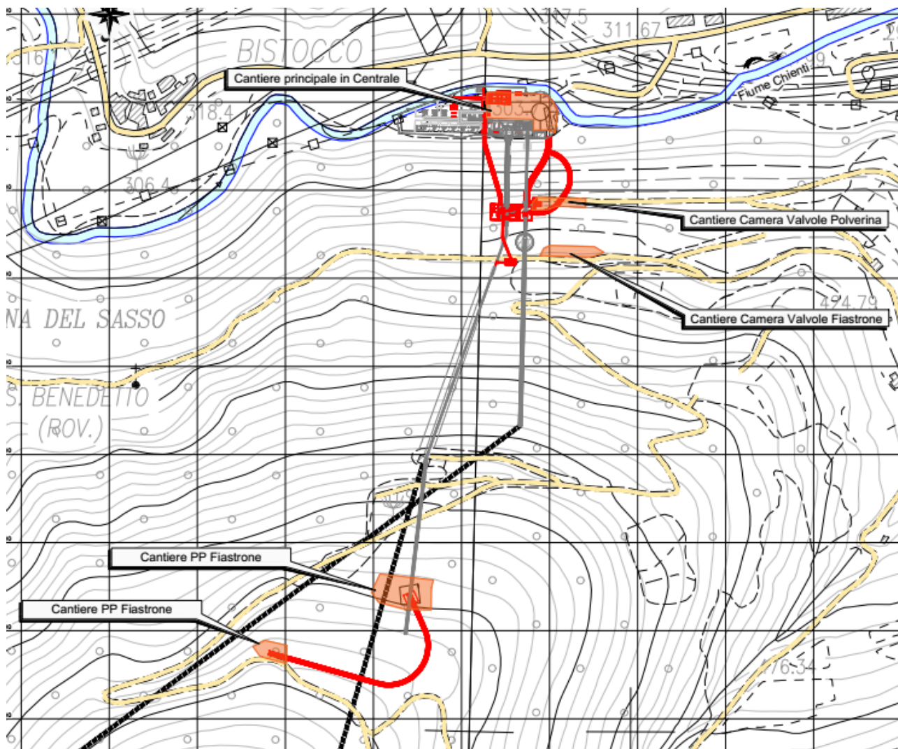
Figura 72: aree di cantiere
