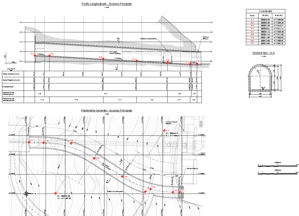
Figura 27: galleria di accesso principale
