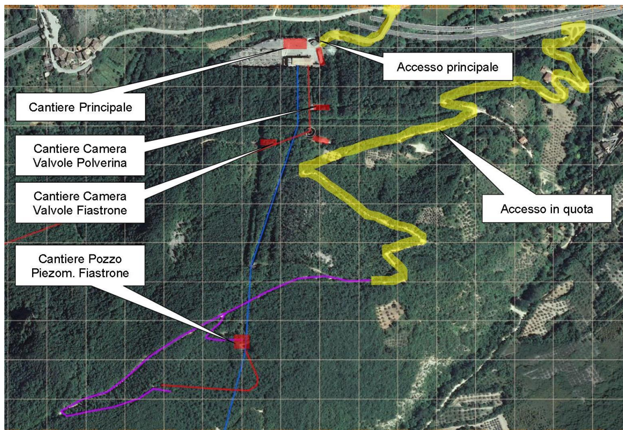
Figura 34: ubicazione delle principali aree di cantiere
