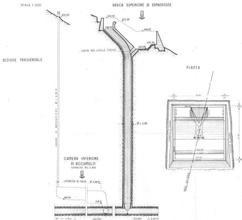
Figura 11: derivazione Fiastrone – pozzo piezometrico
