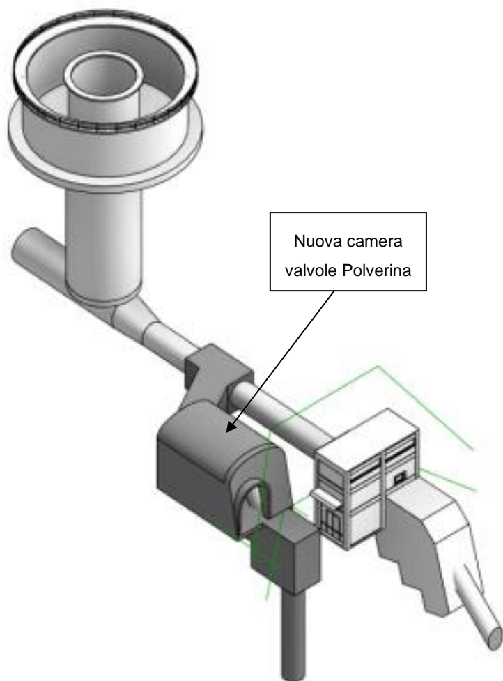
Figura 68: 3d ampliamento camera valvole Polverina
