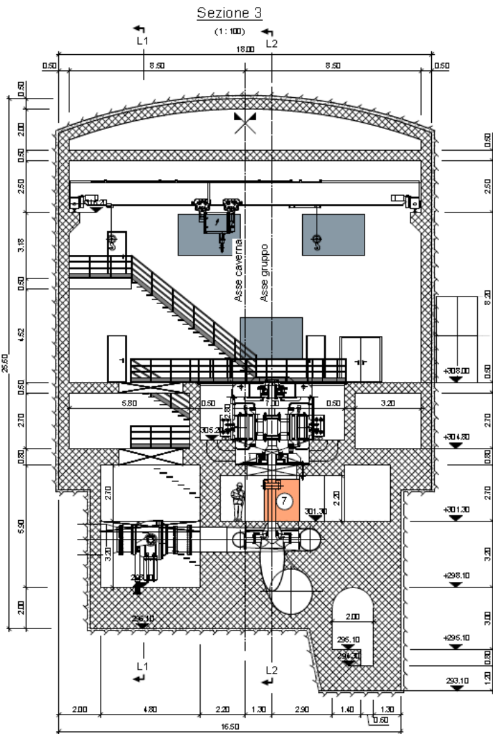
Figura 26: centrale di Valcimarra II – sezione trasversale
