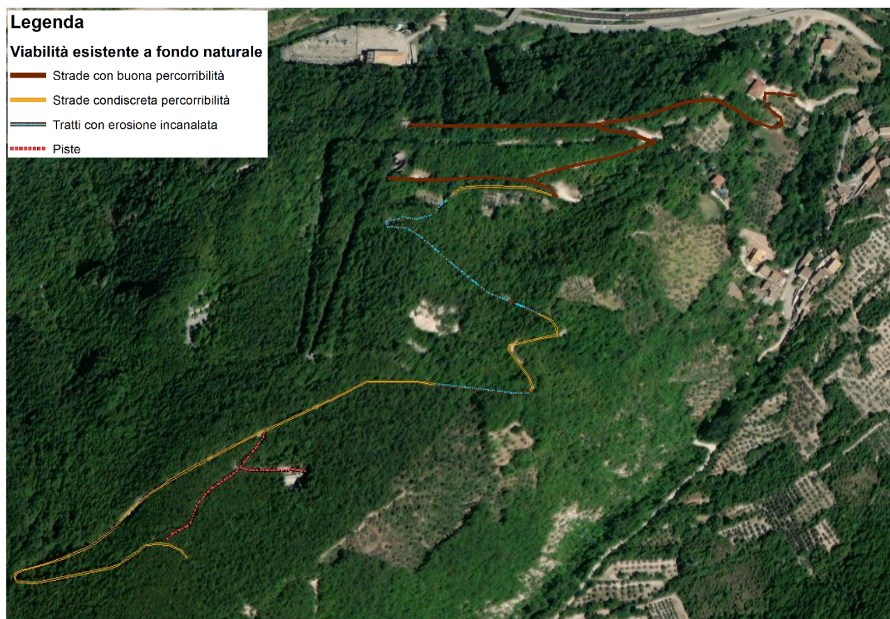
Figura 85: viabilità a fondo naturale
