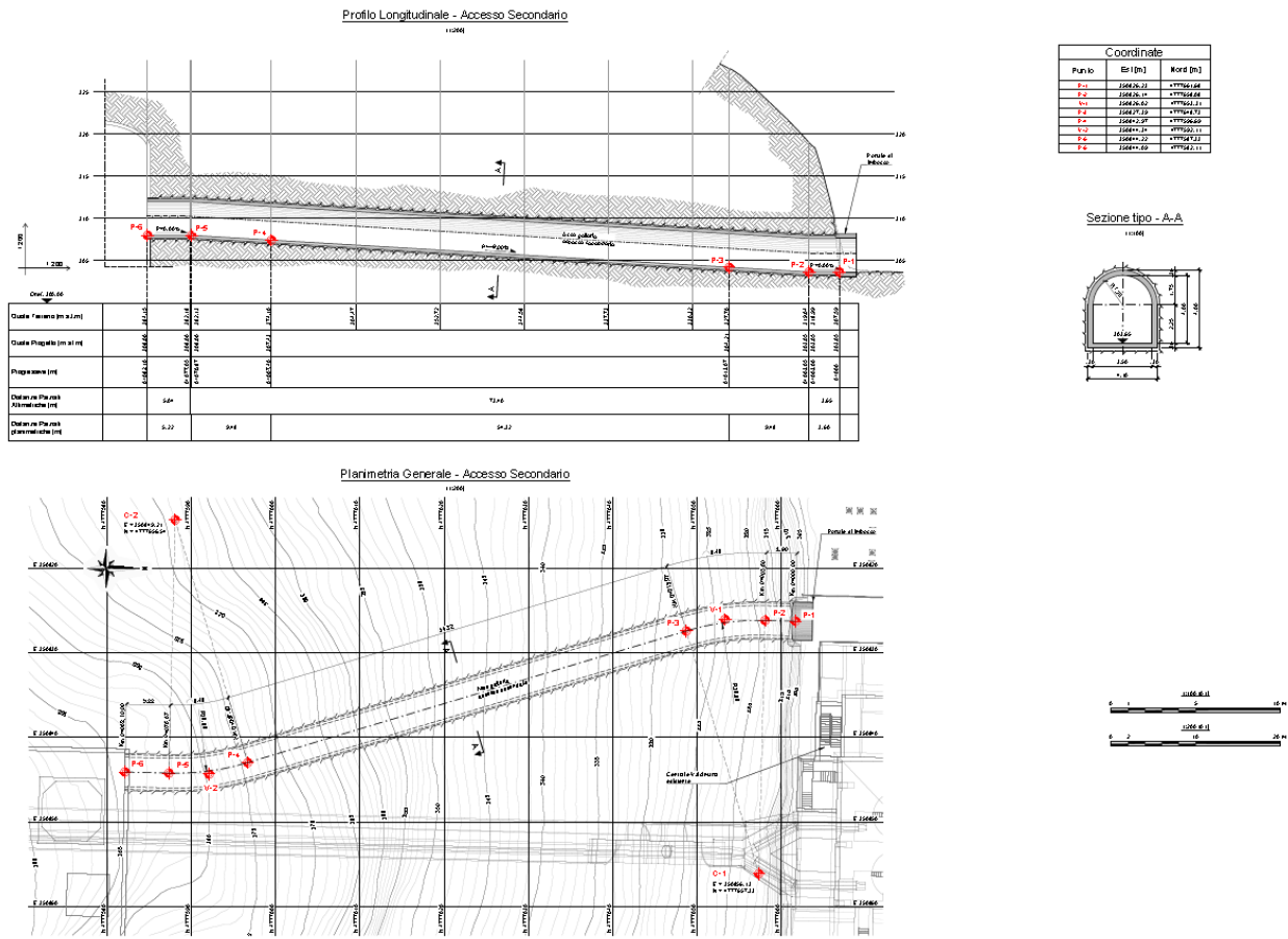
Figura 28: galleria di accesso secondaria
