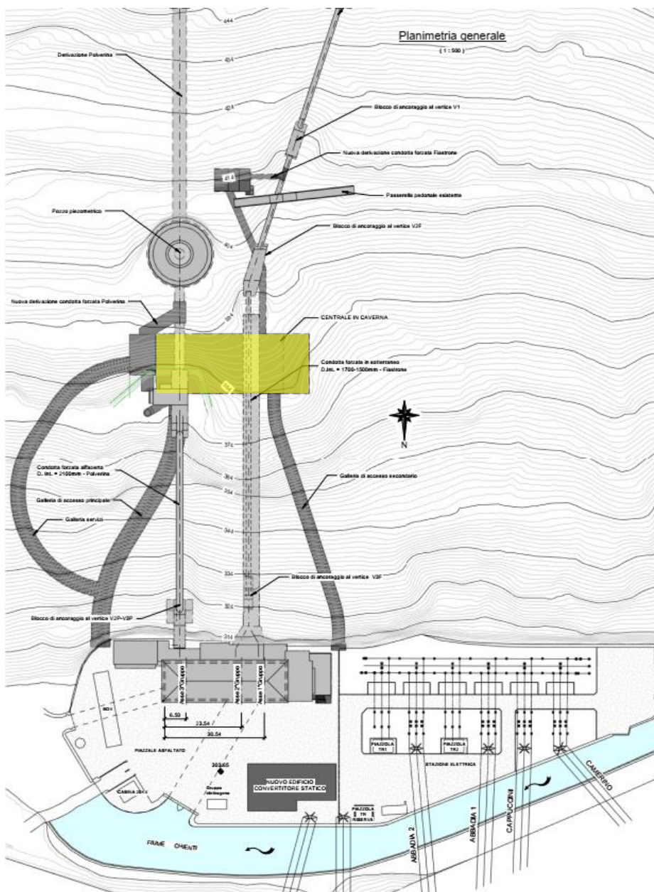
Figura 23: planimetria di progetto - nuova caverna di centrale Valcimarra II (in giallo)
