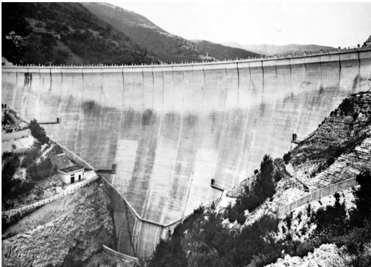
Figura 9: diga del Fiastrone - vista da valle
