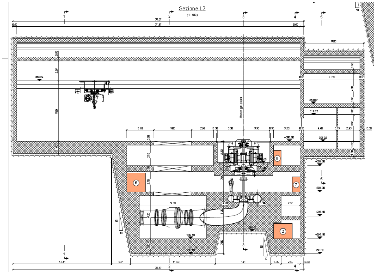
Figura 24: centrale di Valcimarra II – sezione longitudinale
