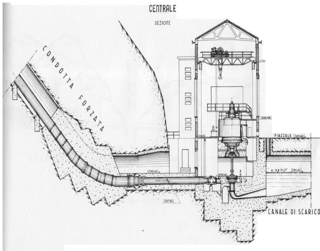
Figura 21: centrale di Valcimarra – sezione trasversale deriv. Fiastrone
