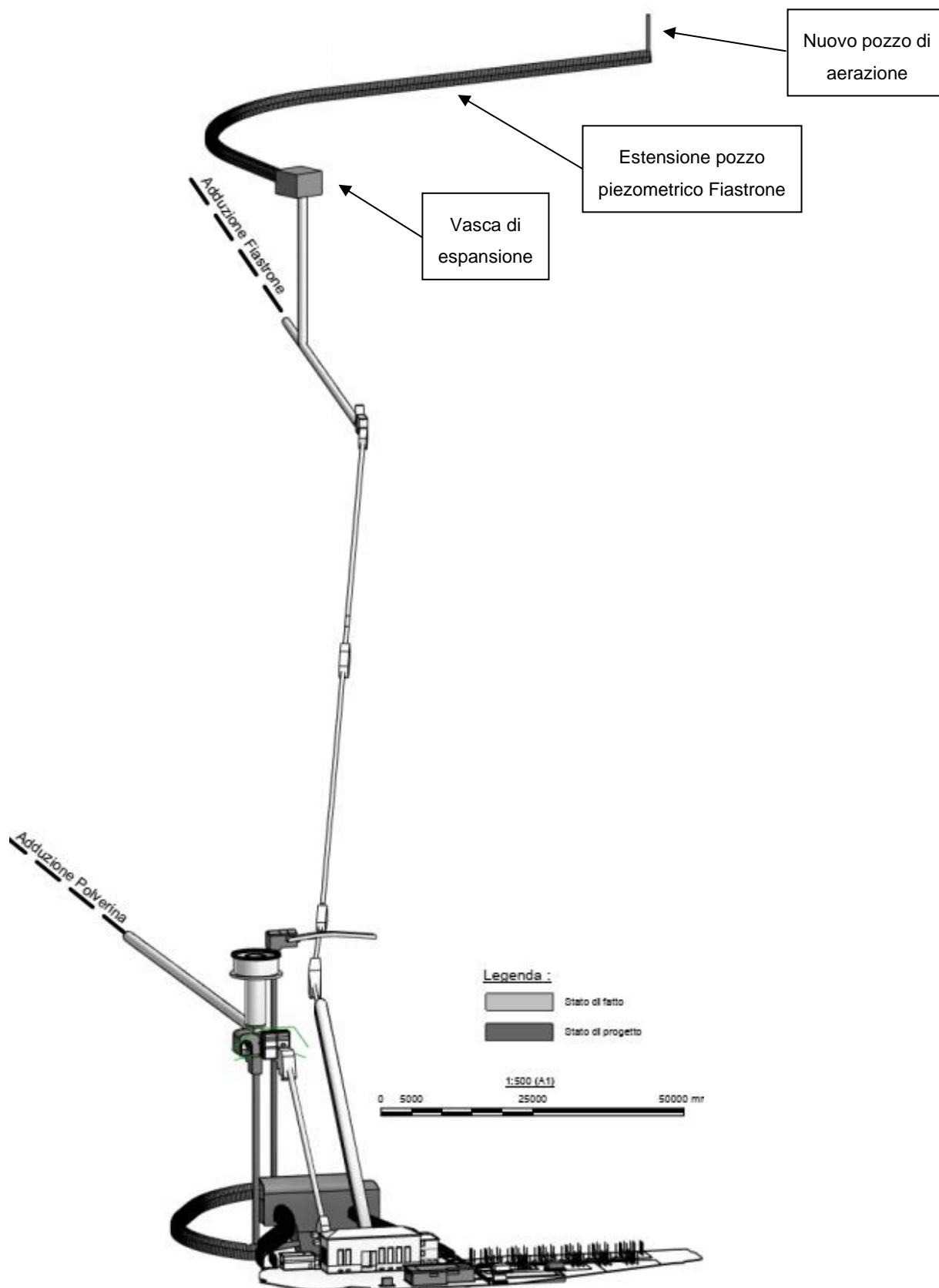
Figura 70: 3d estensione pozzo piezometrico Fiastrone
