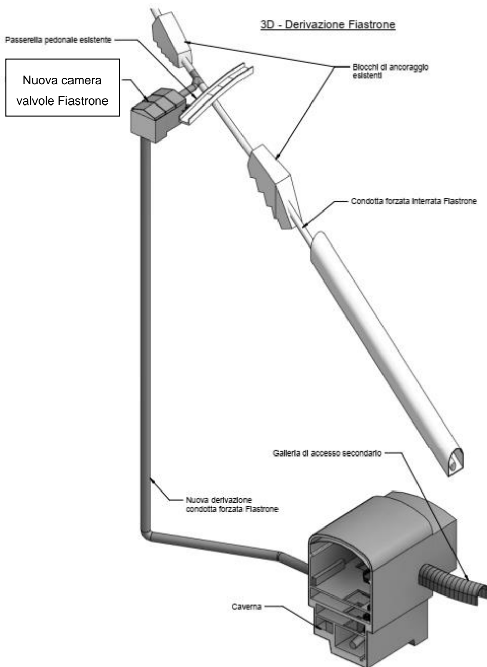
Figura 69: 3d nuova camera valvole Fiastrone
