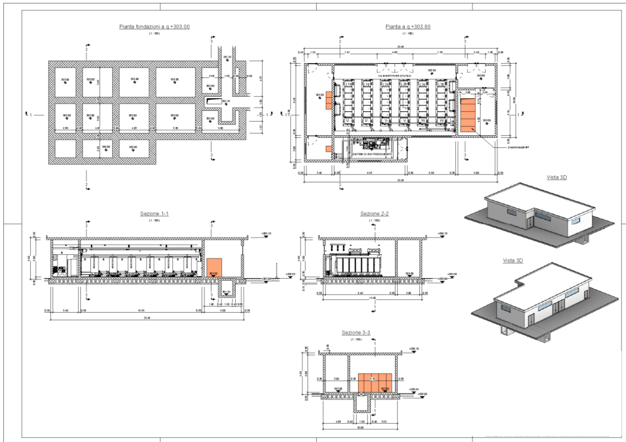
Figura 32: nuovo fabbricato convertitore statico
