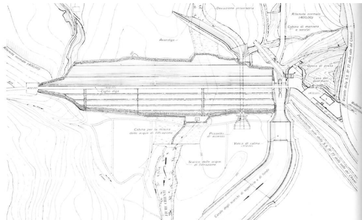
Figura 18: diga di Polverina – planimetria generale
