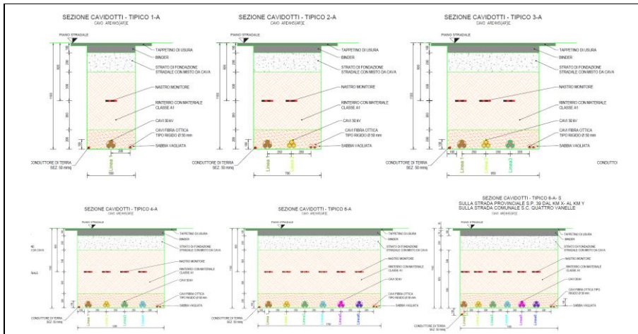
Fig. 13 – Sezioni tipo di scavo su strade asfaltate
