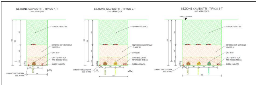
Fig. 15 – Sezioni tipo di scavo su terreno vegetale
