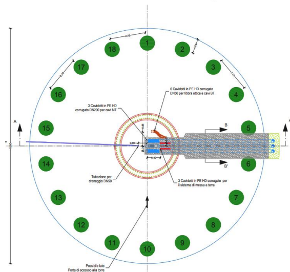
Fig.10 Pianta del plinto con indicazione dei pali di fondazione (n.16 del diametro 100 cm)
