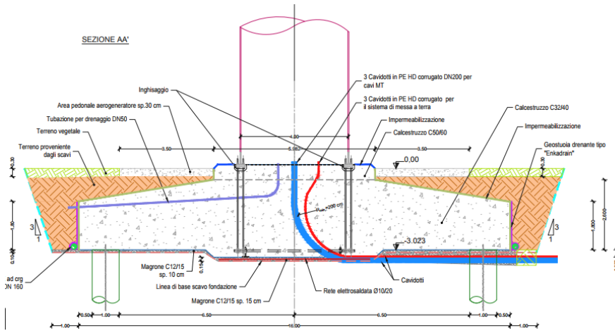
Fig.11 Sezione del plinto
