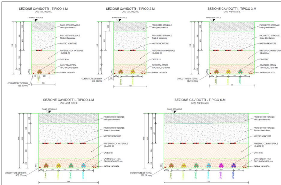
Fig. 14 – Sezioni tipo di scavo su strade sterrate
