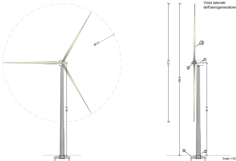
Fig.3 Schema tipo aerogeneratore
