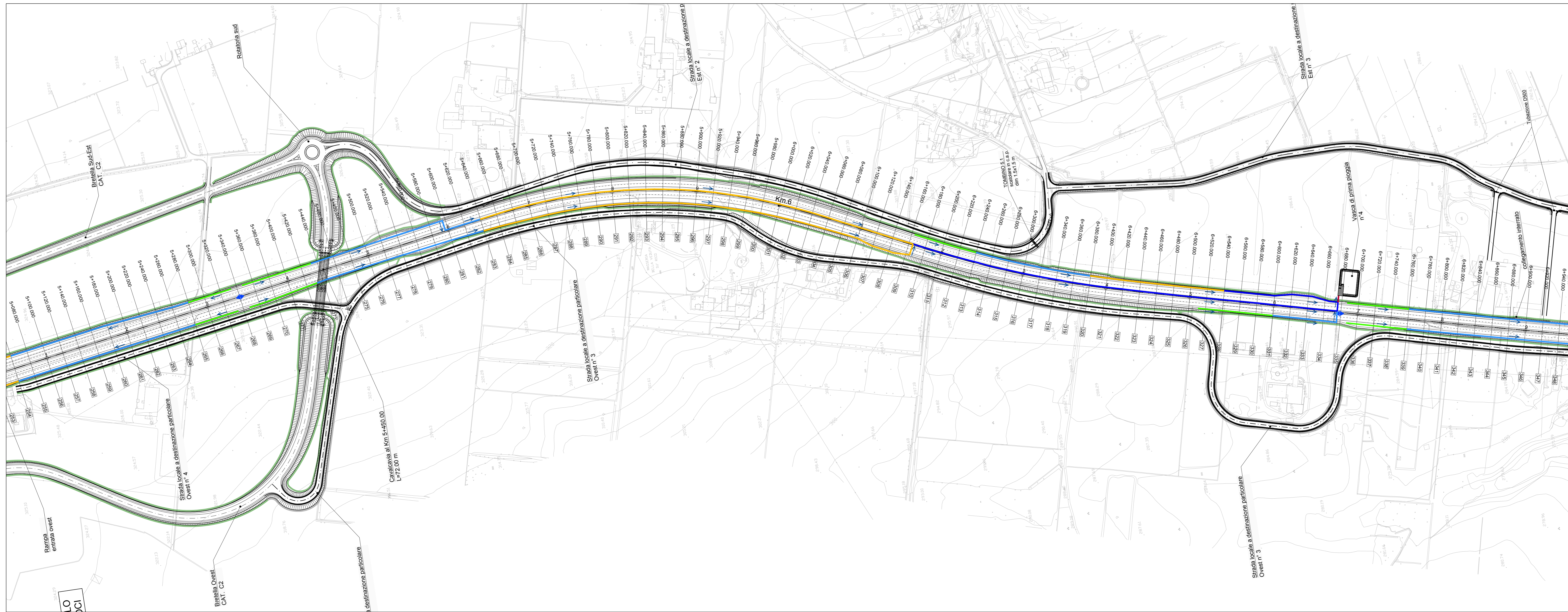
Planimetria smaltimento acque di piattaforma Riquadro 4 di 5 (SCALA 1:2000)
