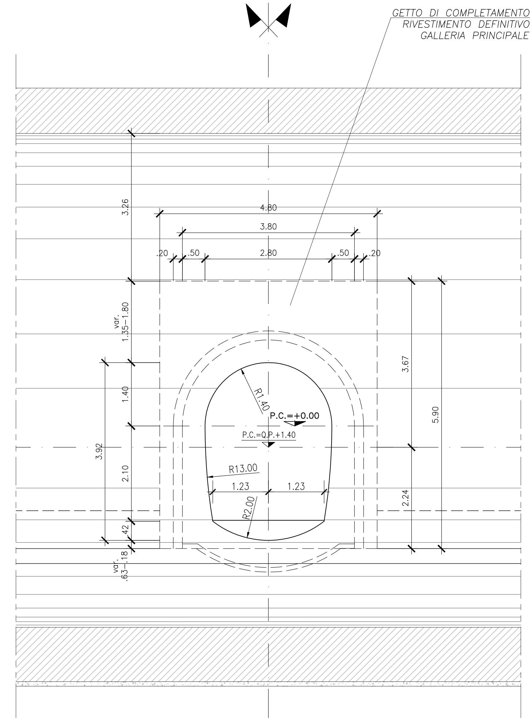
BY-PASS PEDONALE CARPENTERIA DEFINITIVA SEZIONE A-A SCALA 1/50
