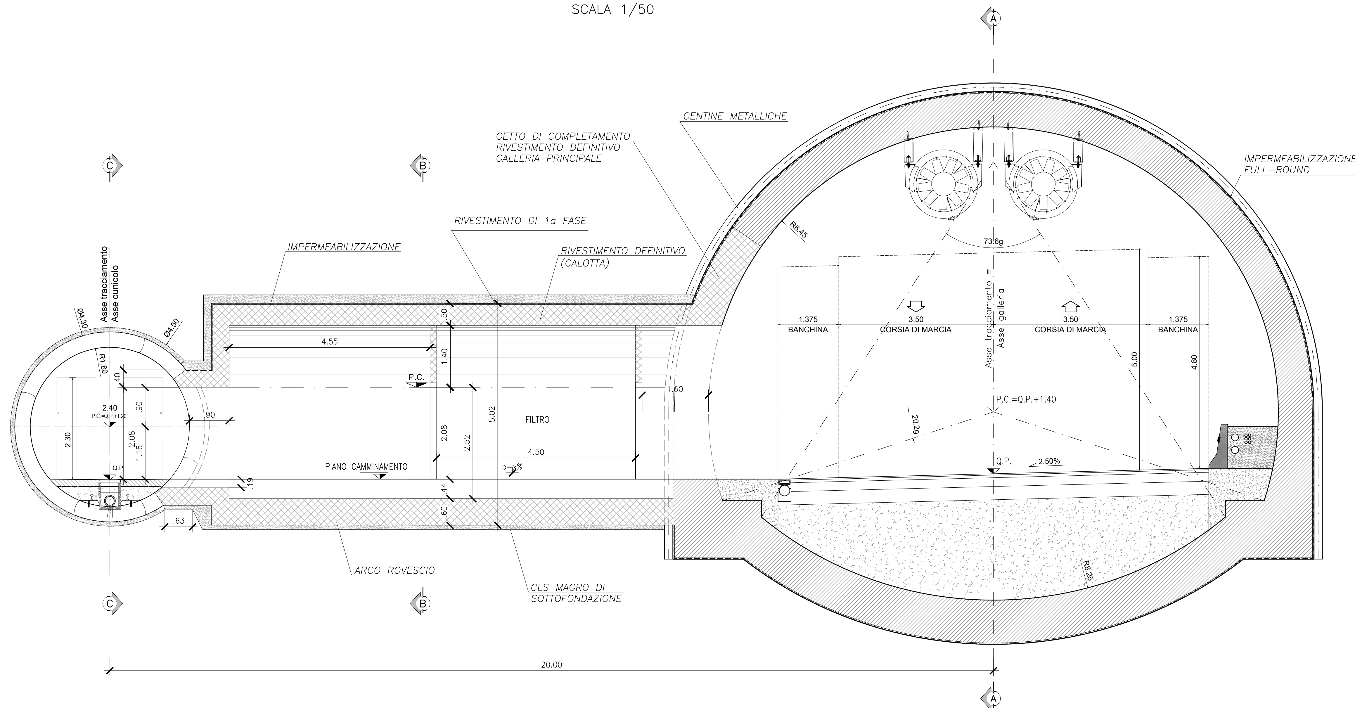
BY-PASS PEDONALE CARPENTERIA DEFINITIVA SEZIONE TRASVERSALE SCALA 1/50
