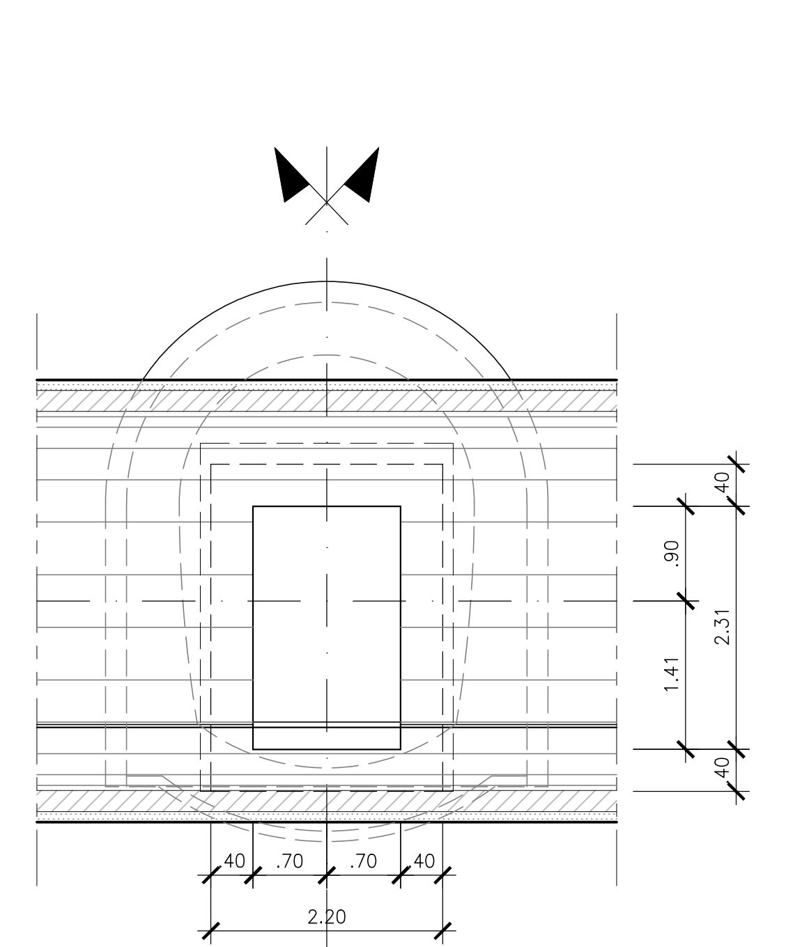
BY-PASS PEDONALE CARPENTERIA DEFINITIVA SEZIONE C-C SCALA 1/50
