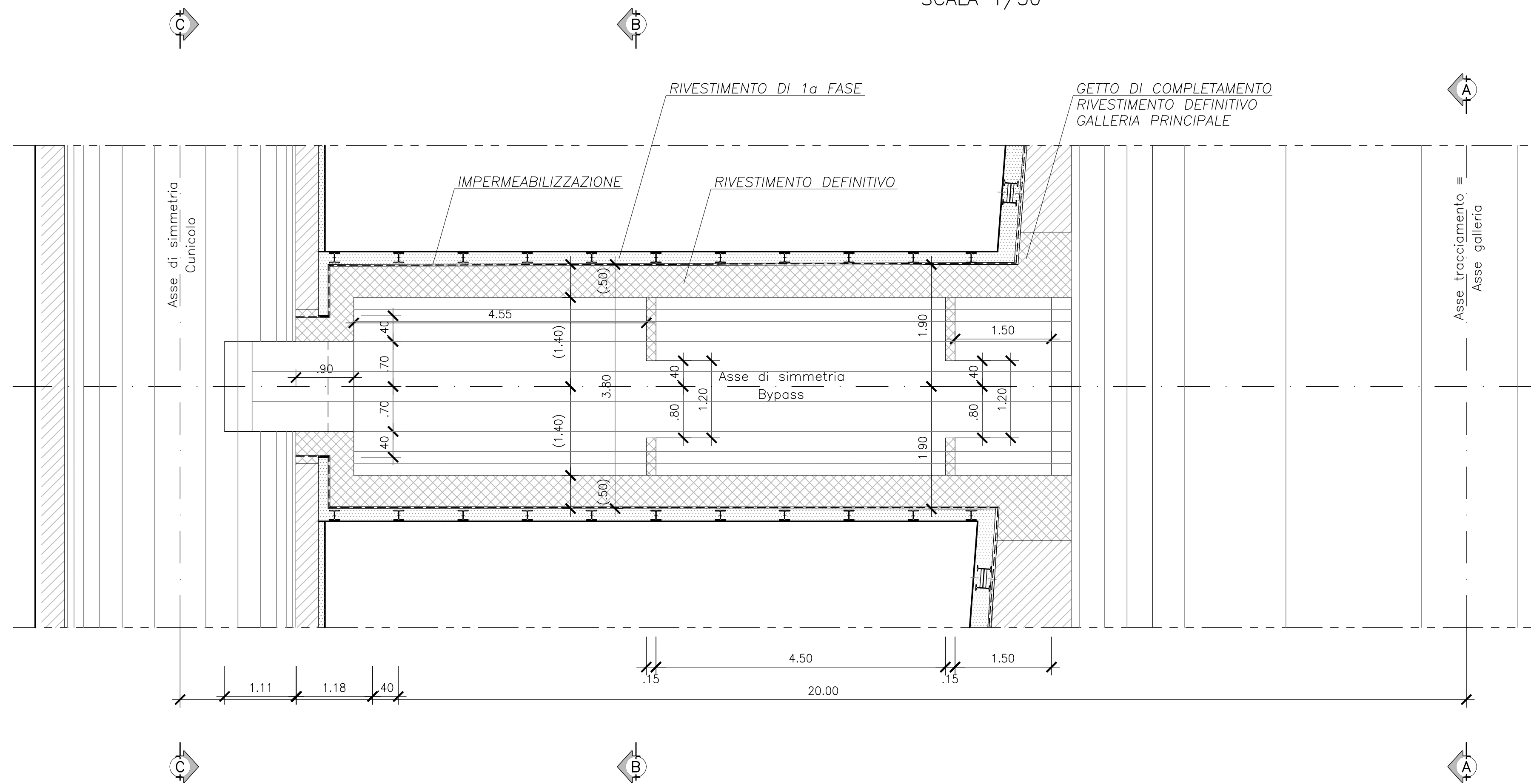
PIANTA CARPENTERIA DEFINITIVA SCALA 1/50
