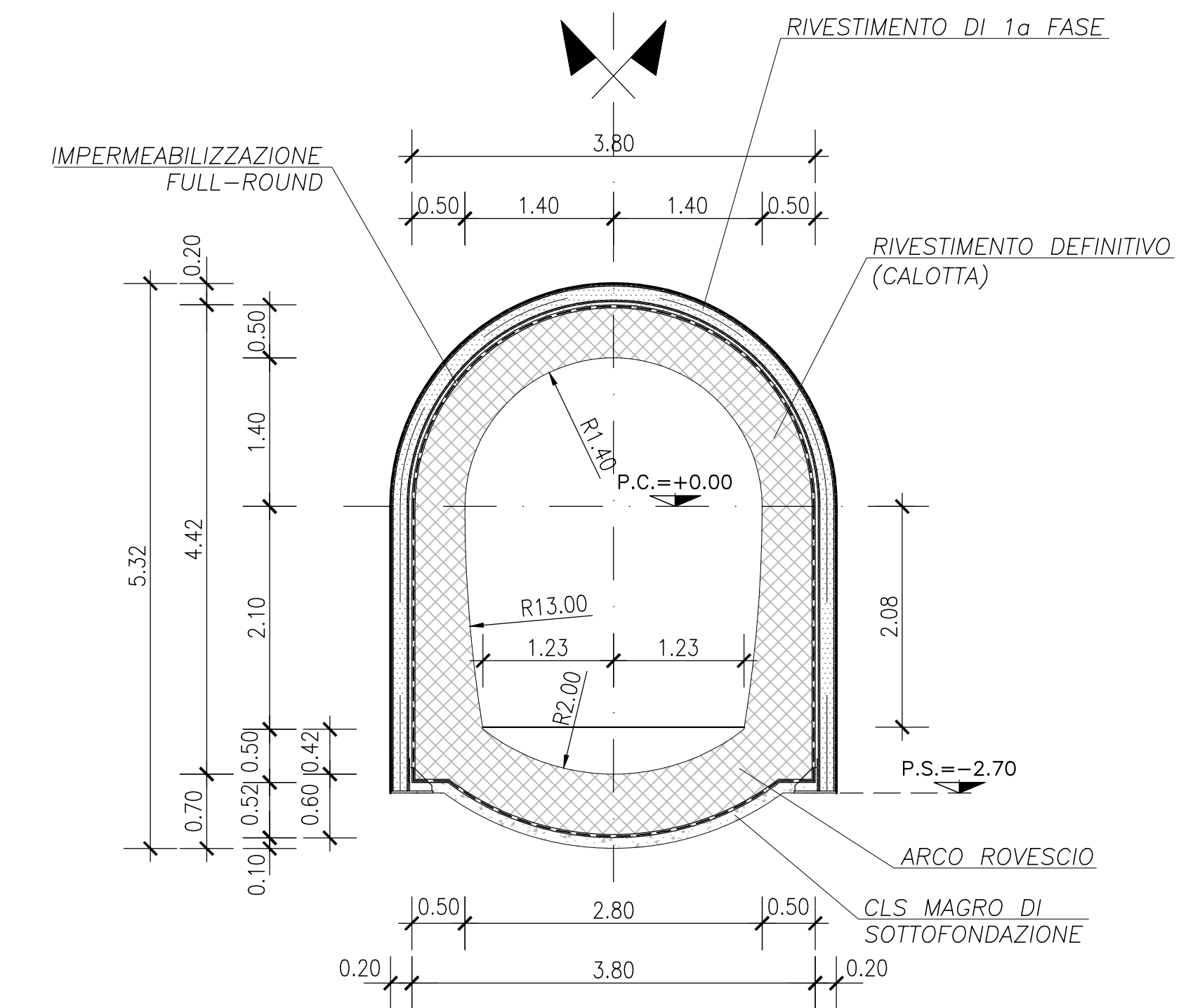
BY-PASS PEDONALE CARPENTERIA DEFINITIVA SEZIONE B-B SCALA 1/50
