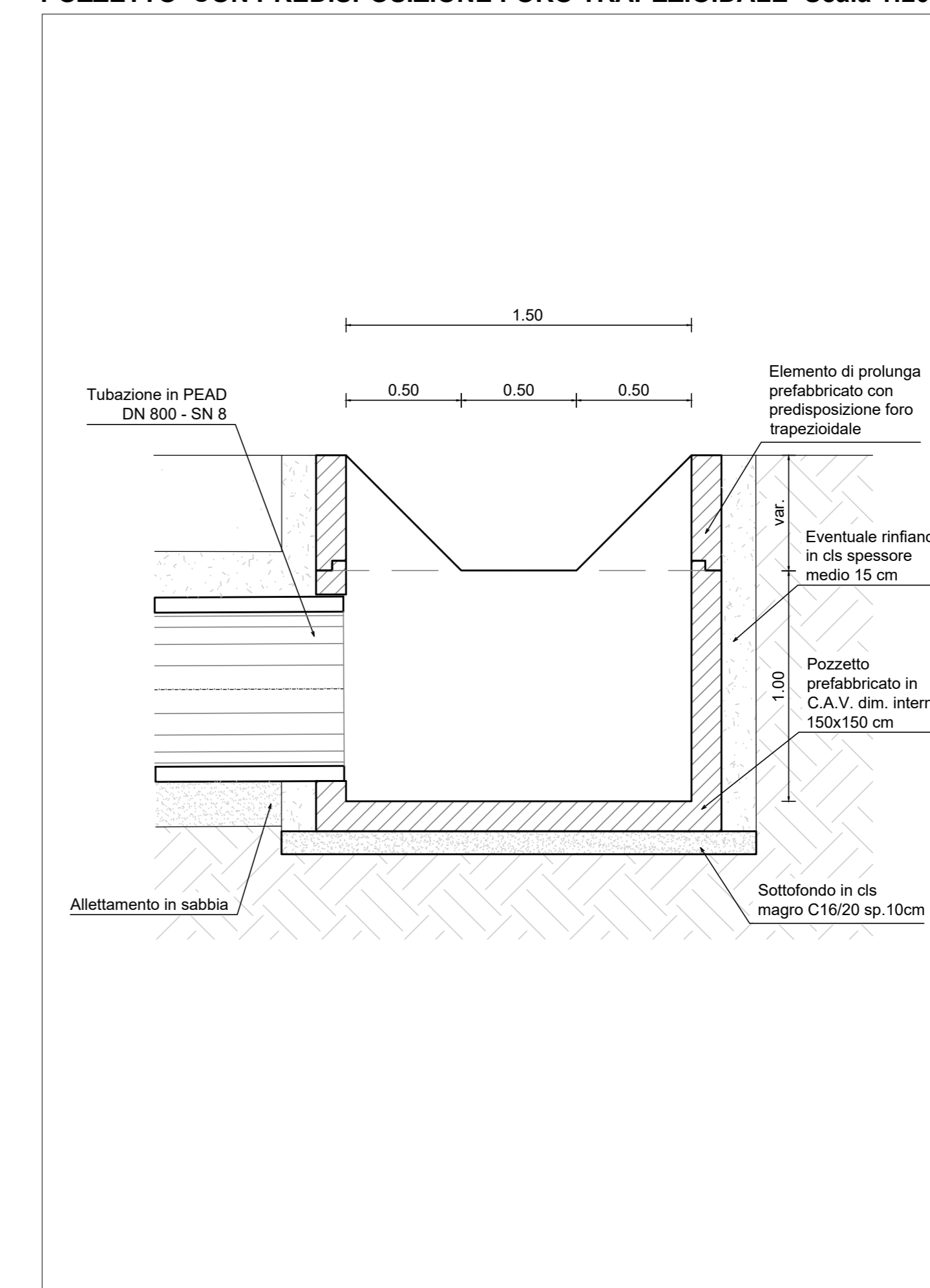
POZZETTO CON PREDISPOSIZIONE FORO TRAPEZIOIDALE - Scala 1:20
