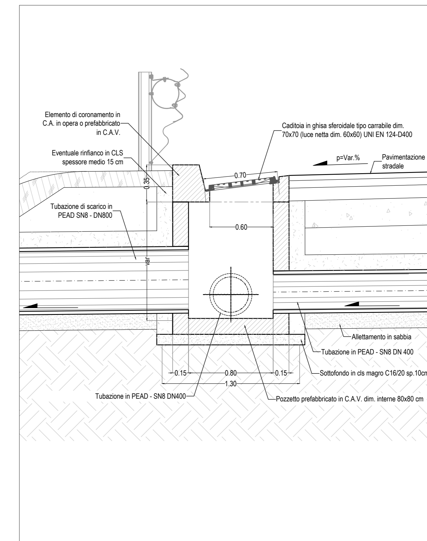
POZZETTO DI LINEA/SCARICO E ISPEZIONE - Scala 1:20
