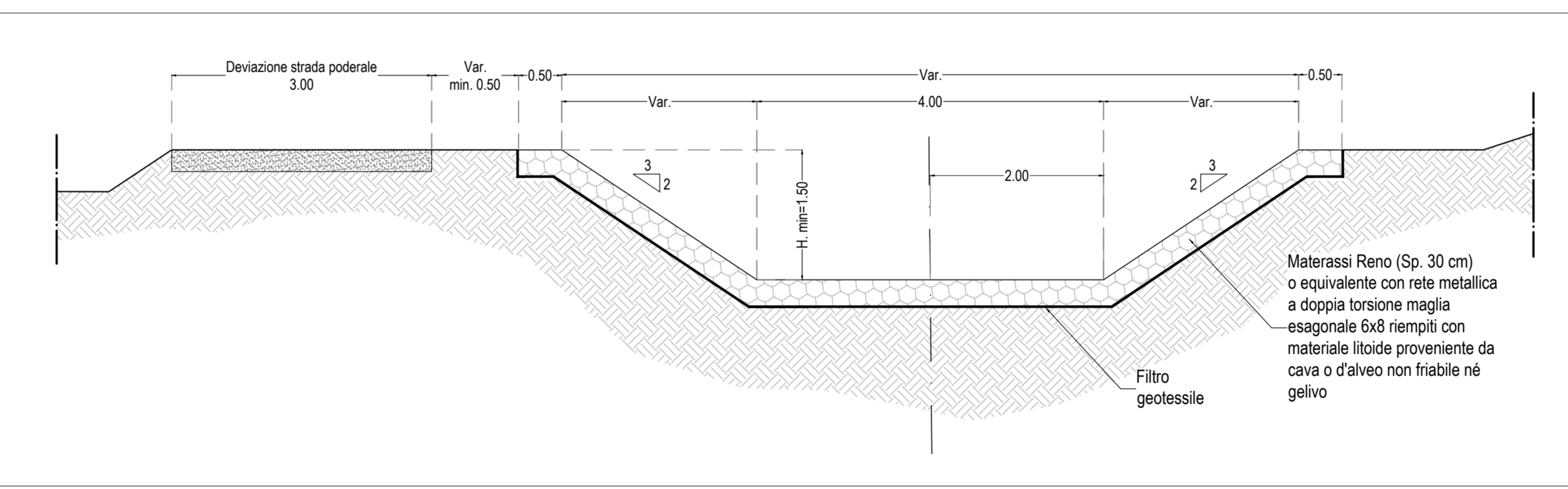
Sezione tipologica di sistemazione dell'asta secondaria Scala 1:50
