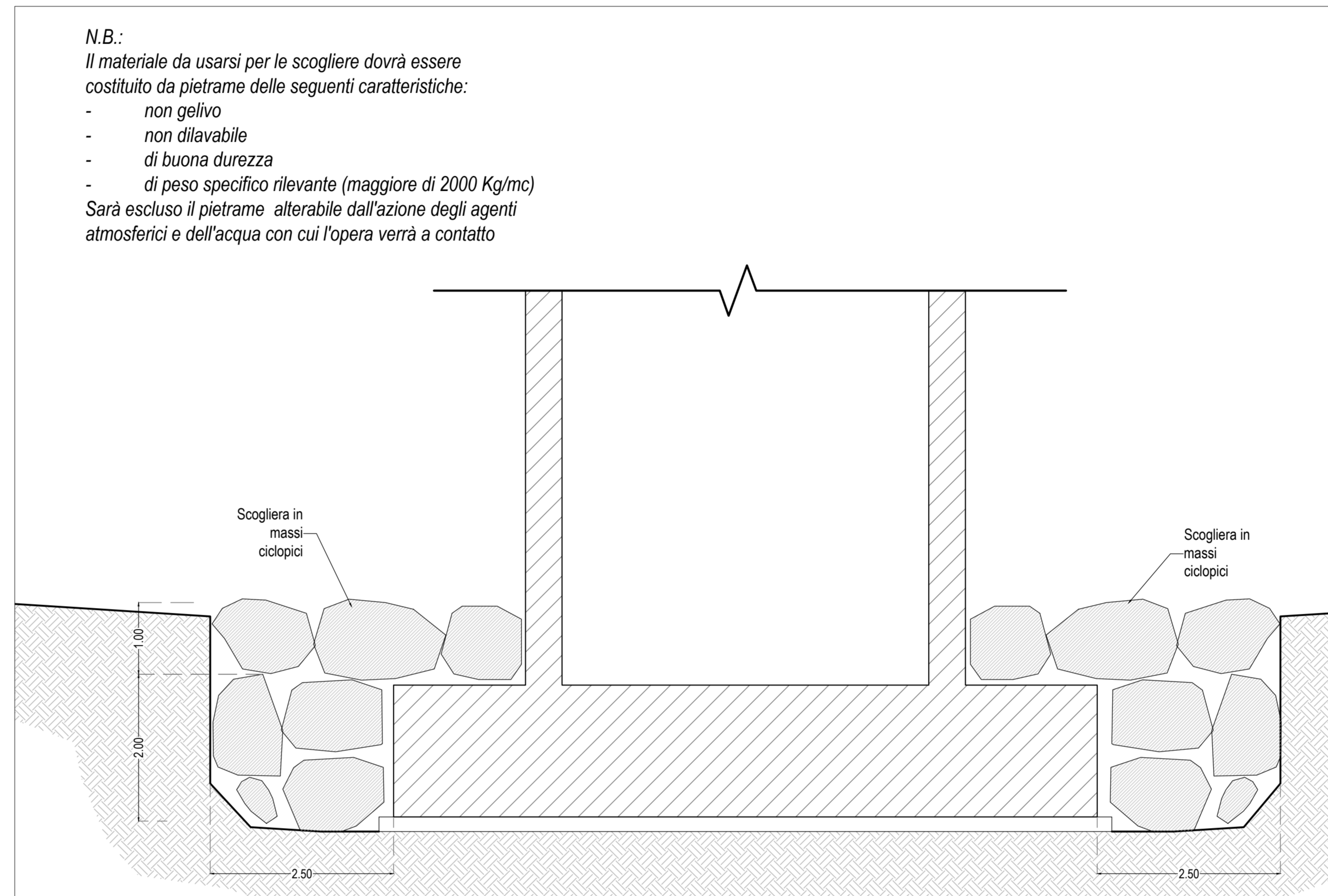
Sezione tipologica di sistemazione dell'asta principale Scala 1:50
