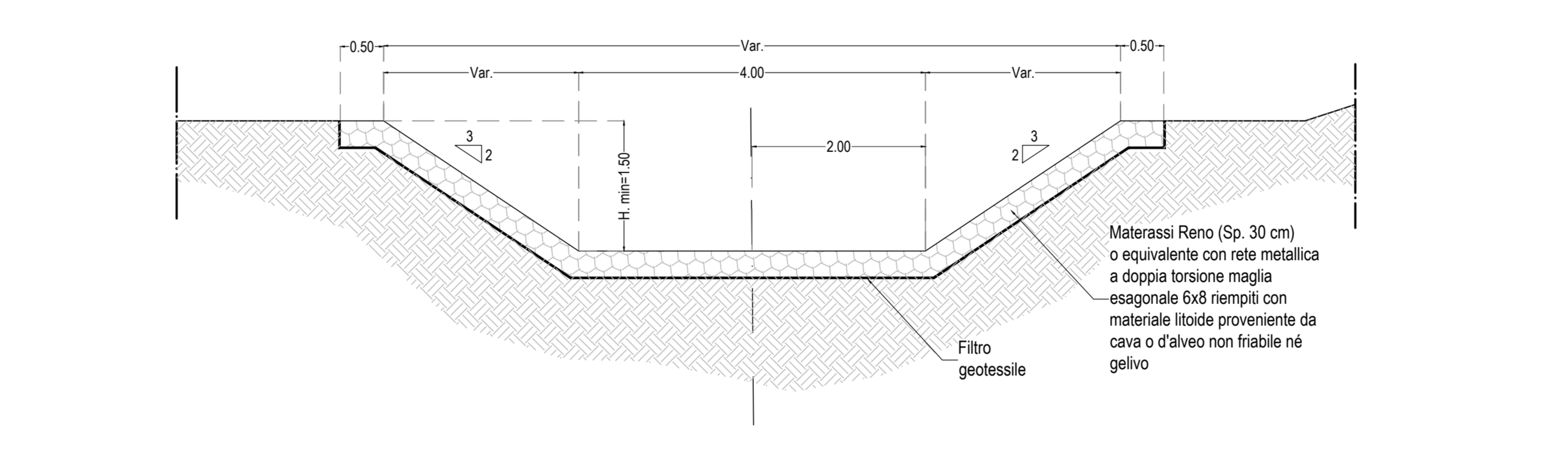
Sezione tipologica di sistemazione dell'asta secondaria Scala 1:50
