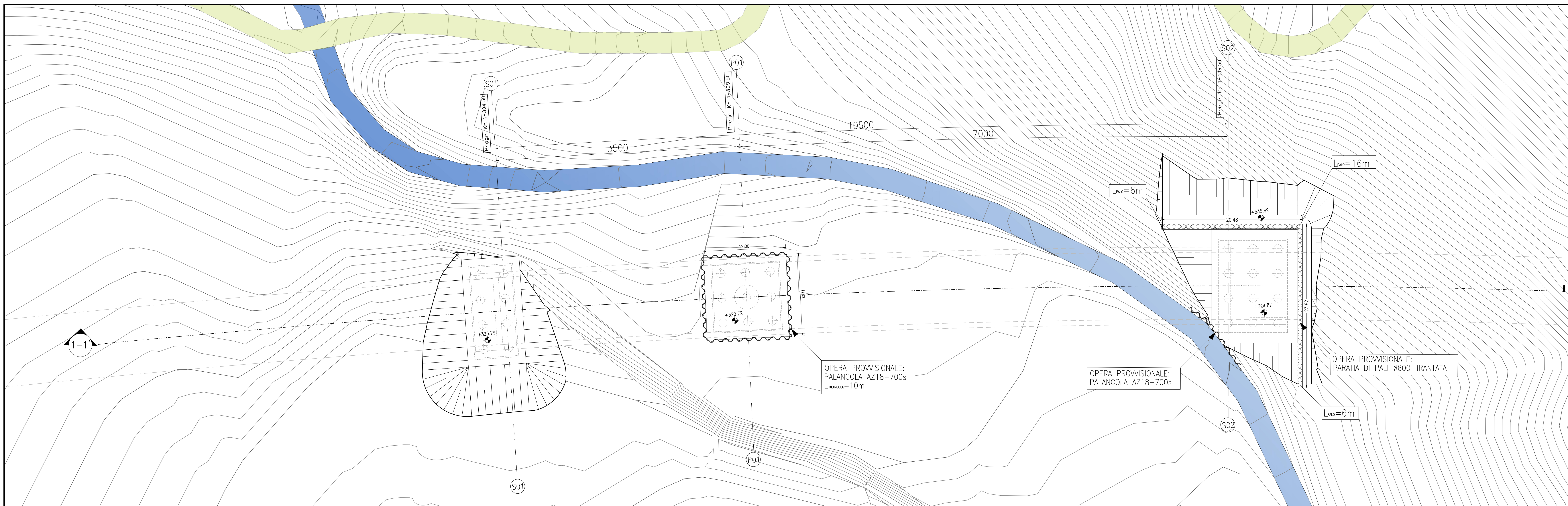
PIANTA SCAVI Scala 1:200
