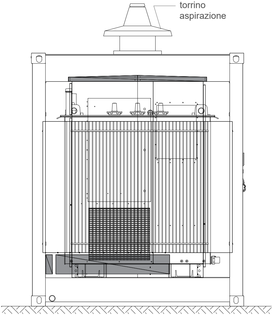
PROSPETTO OVEST
