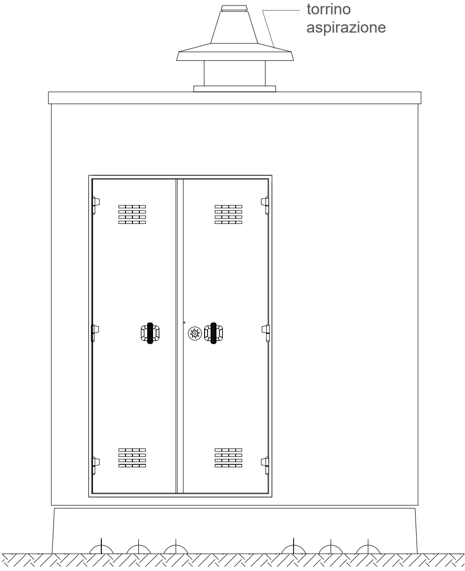
PROSPETTO EST
