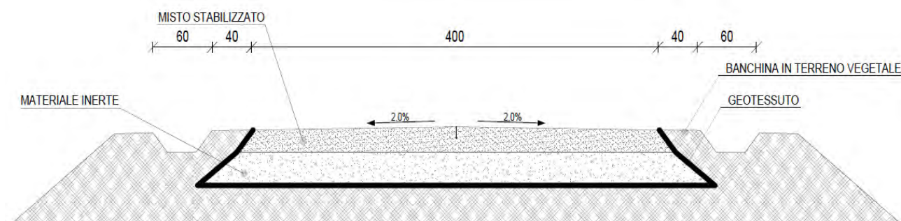
Figura 4-9 sezione tipo viabilità interna
