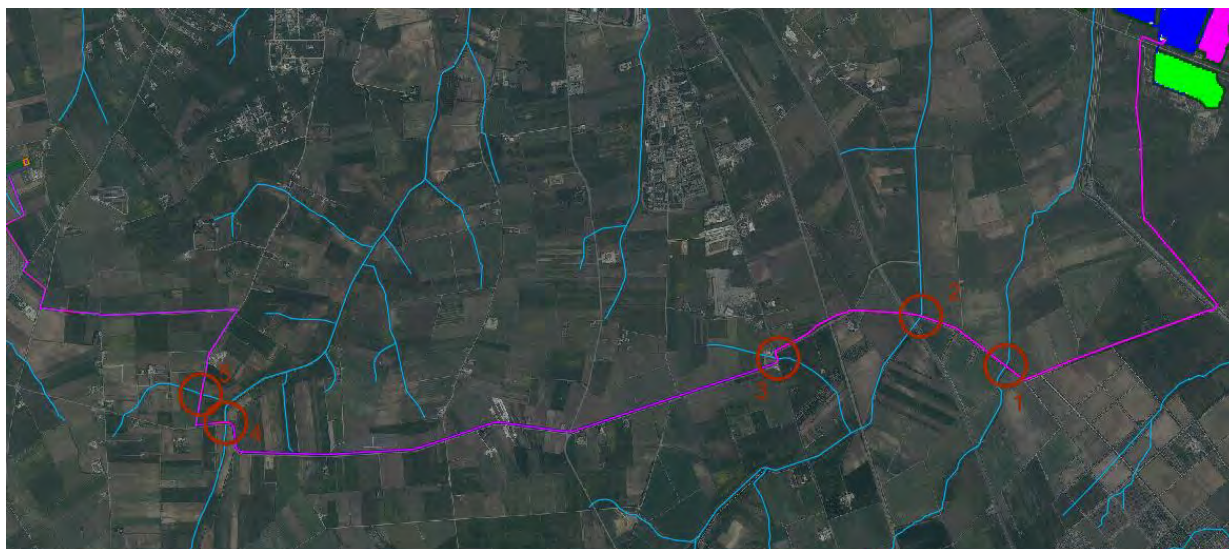
Figura 10- Intersezioni cavidotto con reticolo idrogeomorfologico
