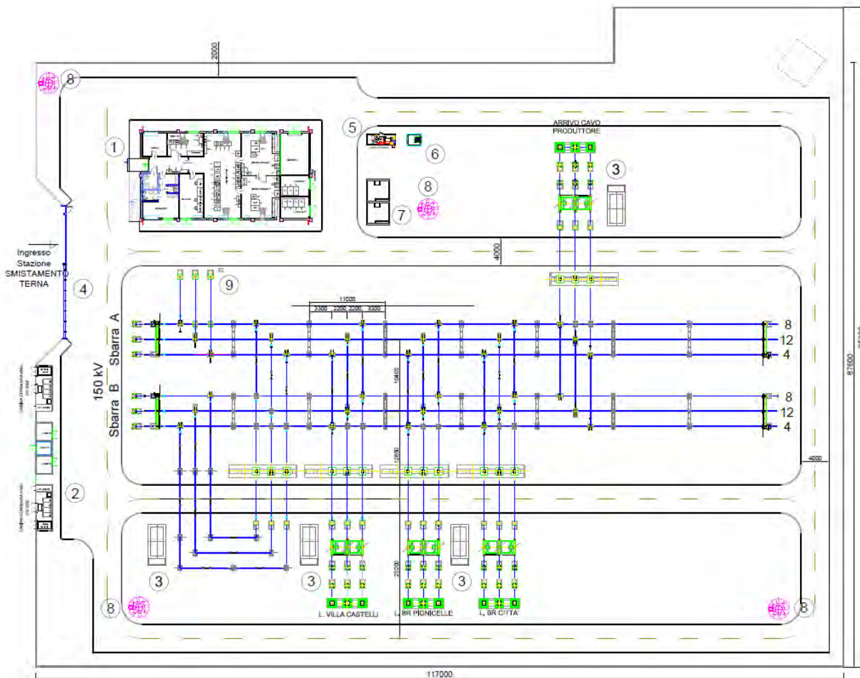
Figura 4-13 - Stazione di smistamento 150kV
