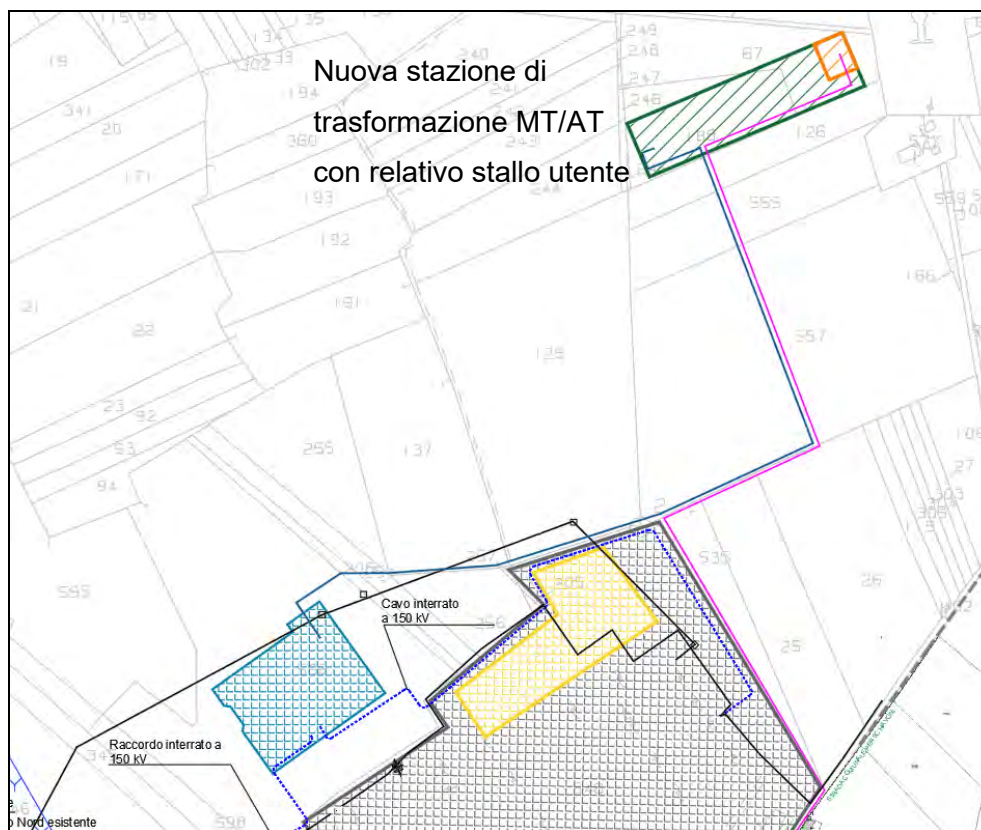
Figura 4-12 Stazione di elevazione MT/AT
