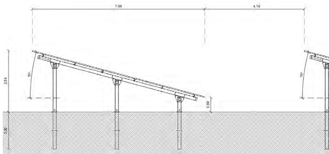
Figura 4-5 Struttura di fondazione dei moduli fotovoltaici
