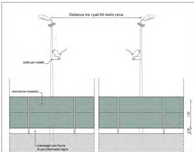
Figura 4-11 Sistema illuminazione e videosorveglianza
