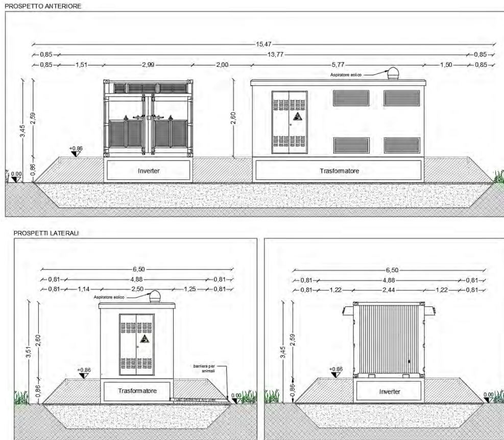
Figura 4-6 Cabine di campo
