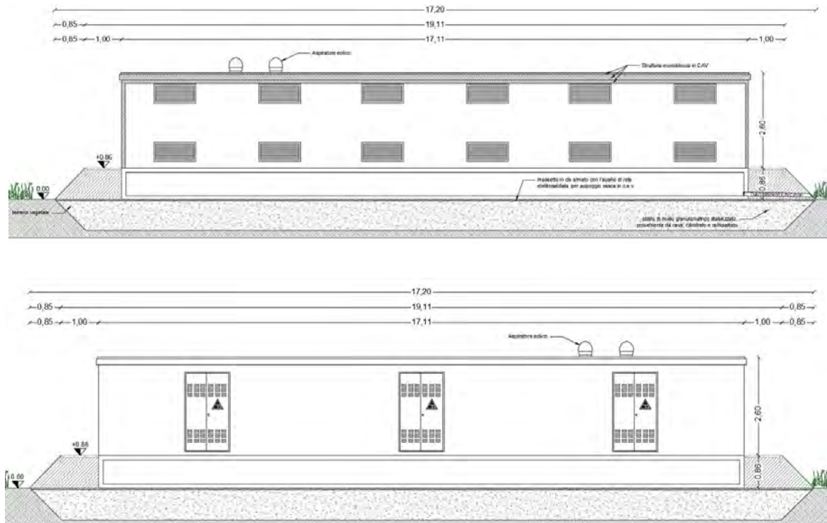
Figura 4-6 Cabine di campo
