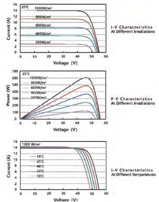
Figura 4-4 Scheda tecnica moduli fotovoltaici di progetto
