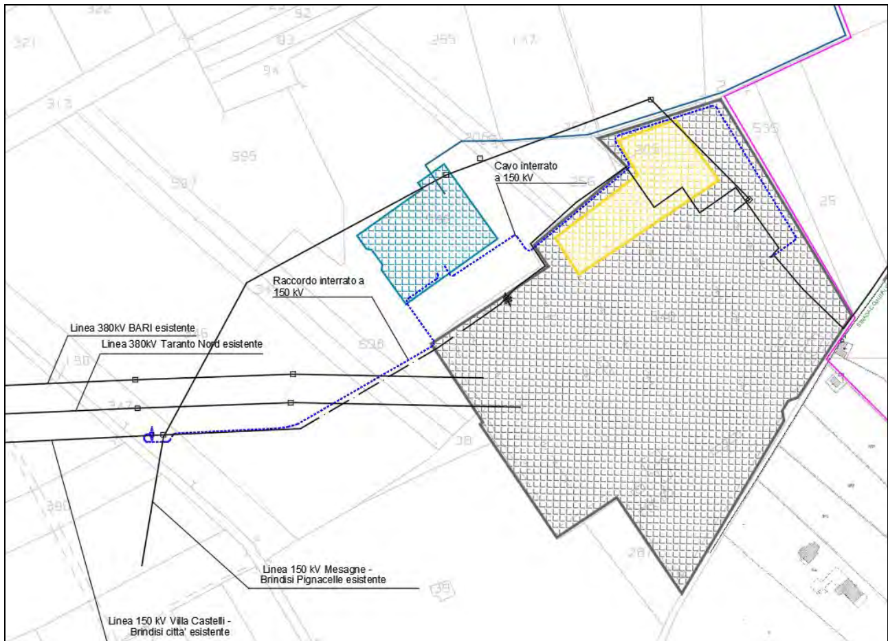
Figura 4-14 - Nuovi raccordi in entra-esce sulla linea Villa Castelli-Brindisi Città
