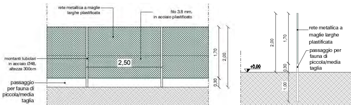
Figura 4-10 Stralcio elaborato AR06-Strutture di supporto dei pannelli fotovoltaici e recinzione
