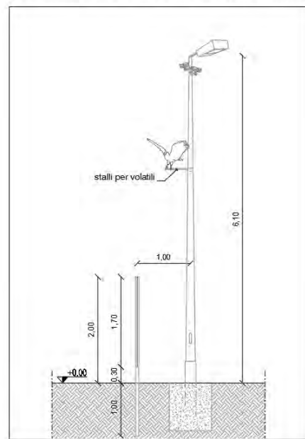
Figura 4-11 Sistema illuminazione e videosorveglianza
