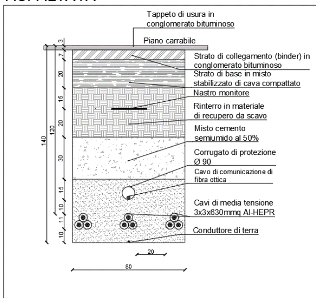
Figura 4-3 Sezioni tipo di posa del Cavidotto interrato
