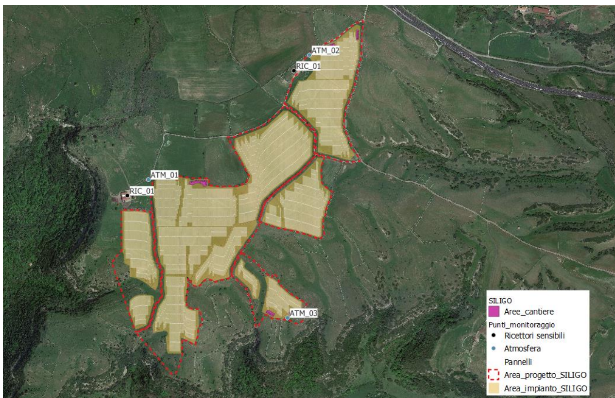
FIGURA 3 – INDIVIDUAZIONE PUNTI DI MONITORAGGIO DELLA QUALITÀ DELL'ARIA (IMMAGINE AGGIORNATA)
