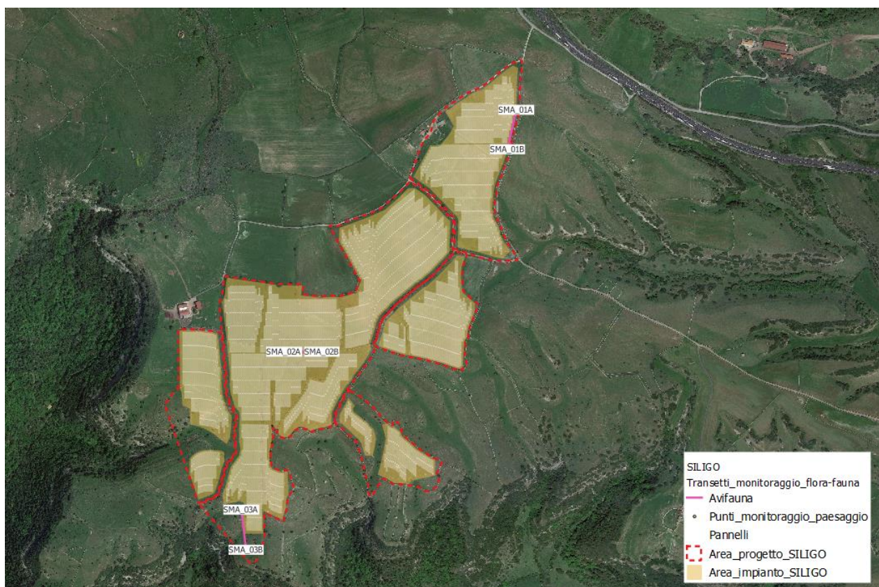
FIGURA 8 - INDIVIDUAZIONE DEI TRANSETTI PER IL MONITORAGGIO DELL'AVIFAUNA (IMMAGINE AGGIORNATA)
