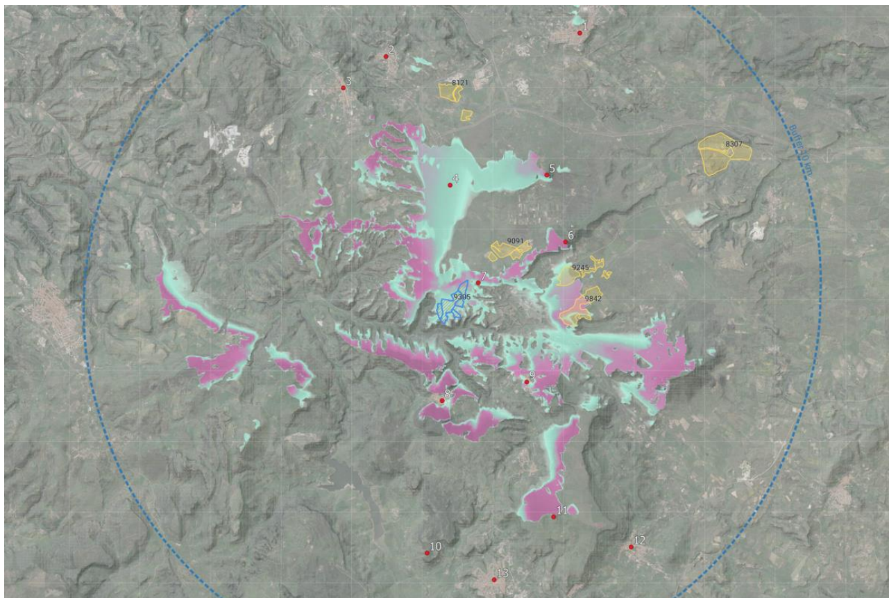
FIGURA 11 – INDIVIDUAZIONE PUNTI DI MONITORAGGIO COMPONENTE PAESAGGIO
