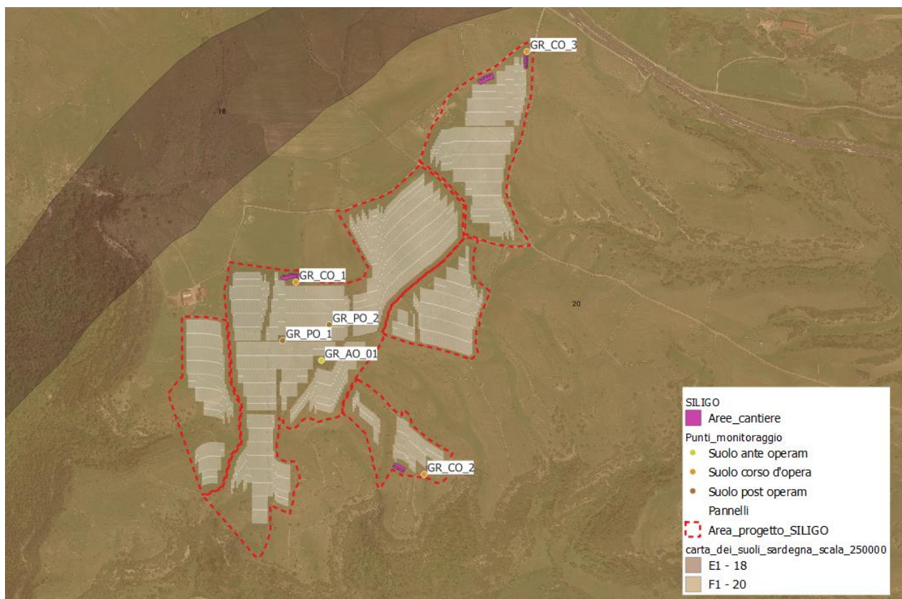
FIGURA 6 – INDIVIDUAZIONE PUNTI DI MONITORAGGIO COMPONENTE SUOLO E SOTTOSUOLO (IMMAGINE AGGIORNATA)
