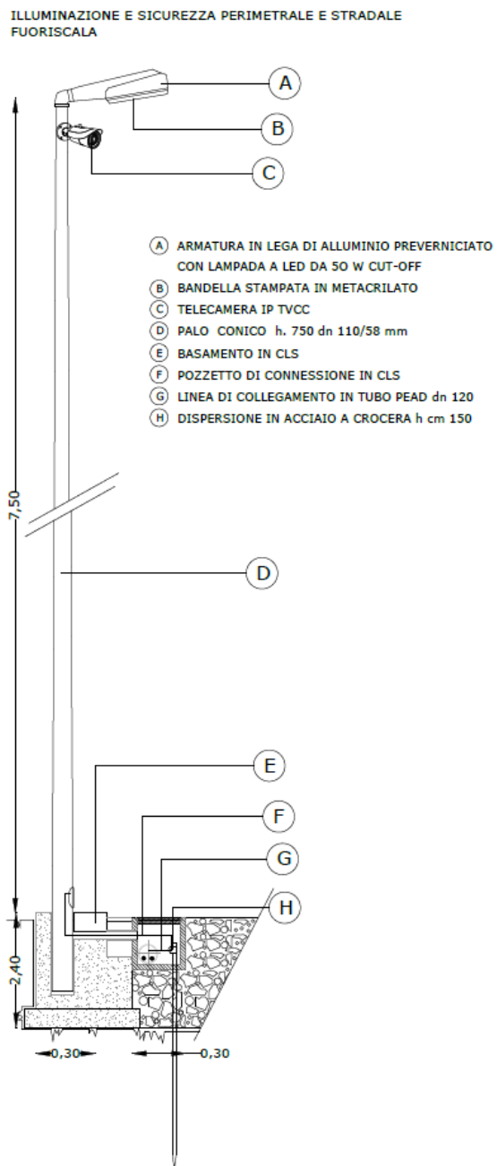
FIGURA 13 – ESEMPIO IMPIANTO DI ILLUMINAZIONE INTEGRATO CON SISTEMA DI VIDEOSORVEGLIANZA – ESTRATTO DALL'ELABORATO TECNICO SIL-PDR02-R1
