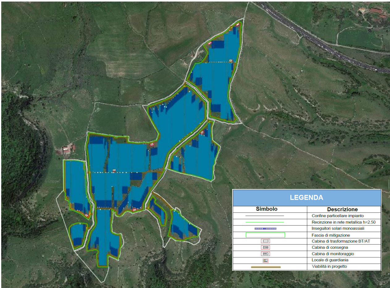
FIGURA 1 – LAYOUT PLANIMETRICO DELL'AREA D'IMPIANTO (IMMAGINE AGGIORNATA)
