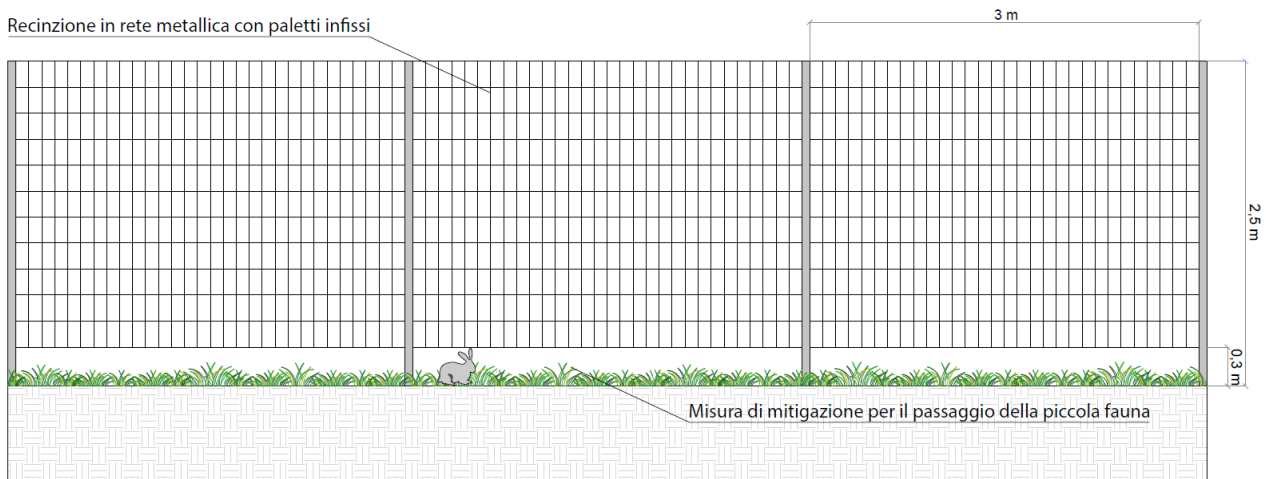
FIGURA 12 – RECINZIONE METALLICA CHE DELIMITA L'AREA DI PERTINENZA DELL'IMPIANTO
