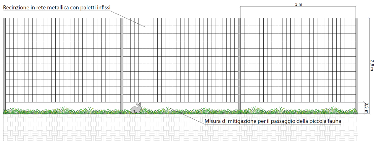
FIGURA 44 - RECINZIONE METALLICA A DELIMITAZIONE DELL'AREA DI IMPIANTO
