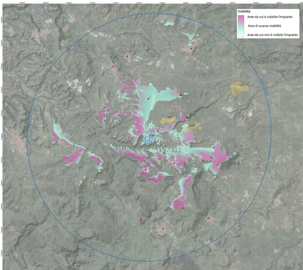
FIGURA 38 - ESTRATTO MAPPA DI INTERVISIBILITÀ TEORICA IMPIANTO - CODICE ELABORATO SIL-IAT18-R1 (IMMAGINE AGGIORNATA)
