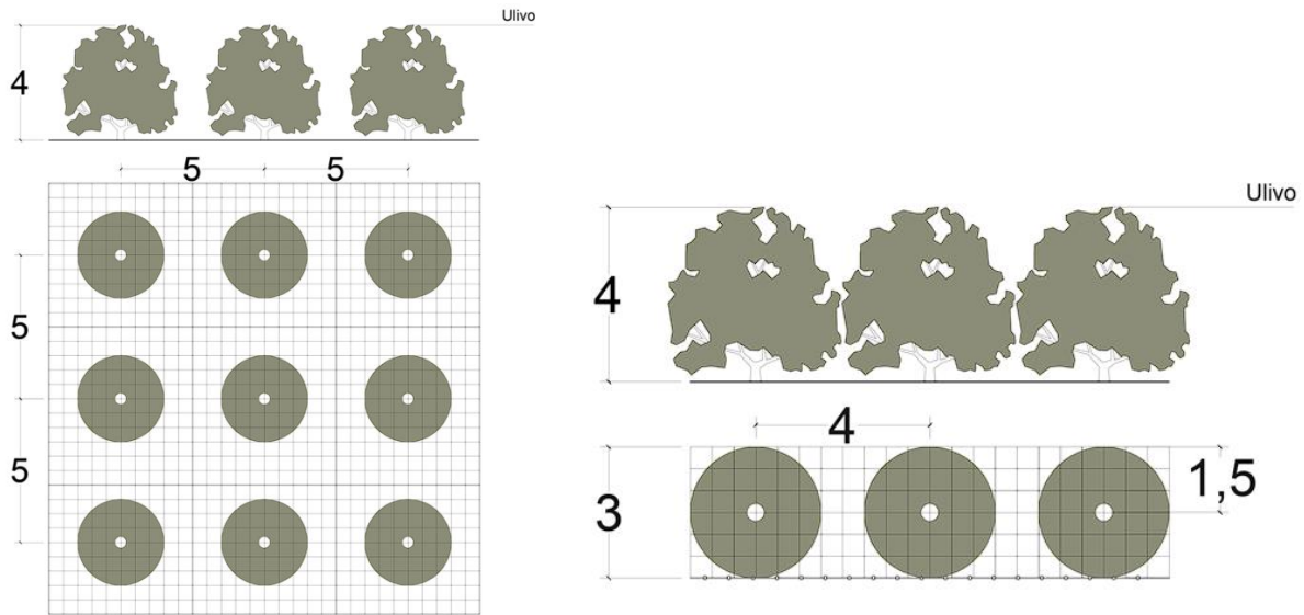
FIGURA 28 – SCHEMA D’IMPIANTO (ESTRATTO DALL’ELABORATO GRAFICO SIL-PDT11-R1 ) (IMMAGINE AGGIORNATA)
