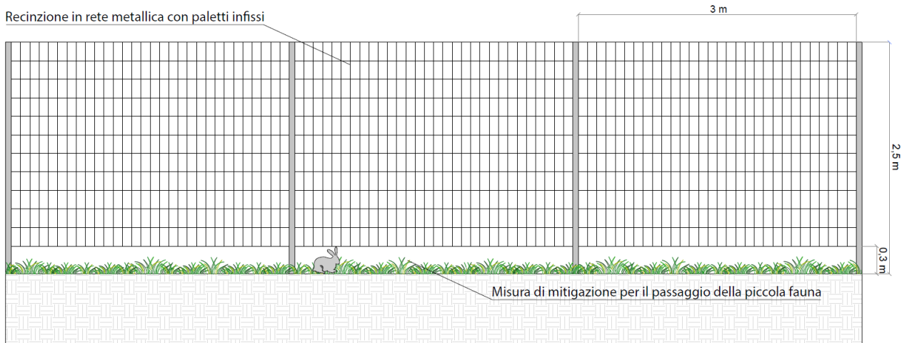
FIGURA 43 - RECINZIONE METALLICA A DELIMITAZIONE DELL'AREA DI IMPIANTO
