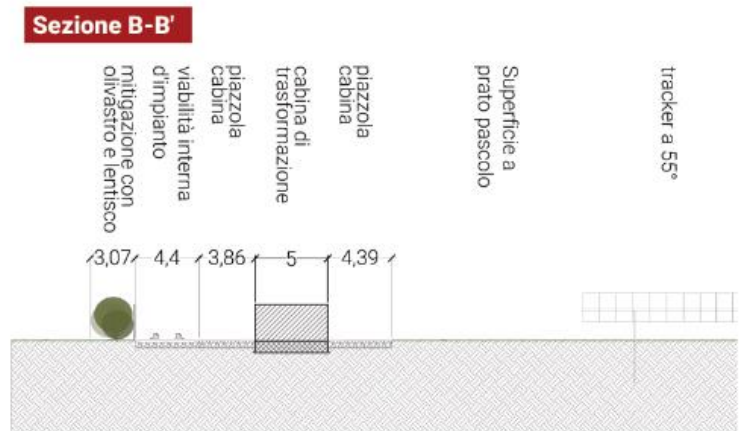
FIGURA 30 – PARTICOLARE FASCIA DI MITIGAZIONE E CABINA DI TRASFORMAZIONE – SEZIONE N-S DELL’IMPIANTO – ESTRATTO DALL’ELABORATO GRAFICO SIL-PDT11-R1 ) (IMMAGINE AGGIORNATA)
