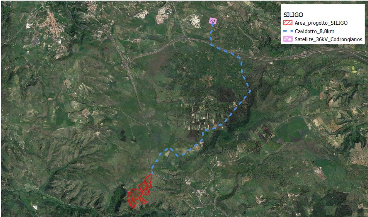
FIGURA 24 – ALTERNATIVA 2 DI IMPIANTO PER IL PROGETTO SILIGO (IMMAGINE AGGIORNATA)
