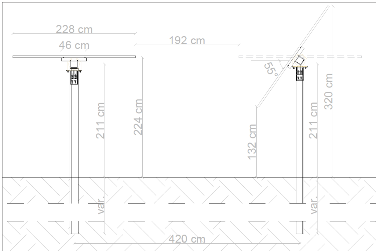
FIGURA 25 – TRACKER TIPO AD ASSE VARIABILE (IMMAGINE AGGIORNATA)
