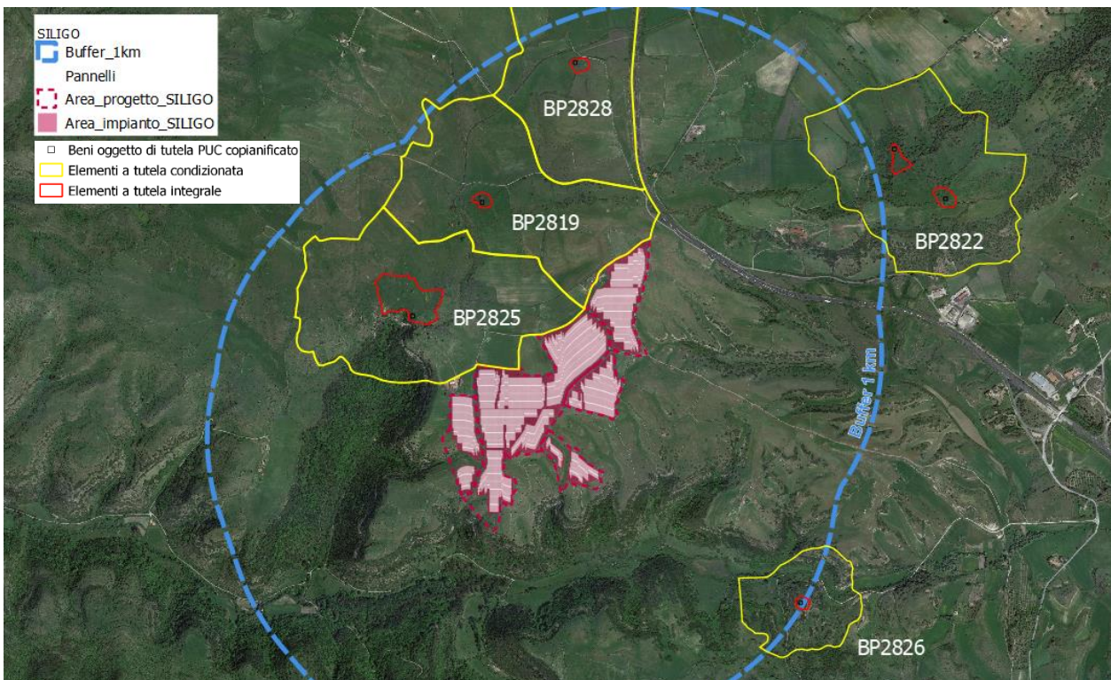
FIGURA 18 - RISOLUZIONE DELL'INTERFERENZA TRA L'AREA DI PROGETTO E LE ZONE A TUTELA CONDIZIONATA
