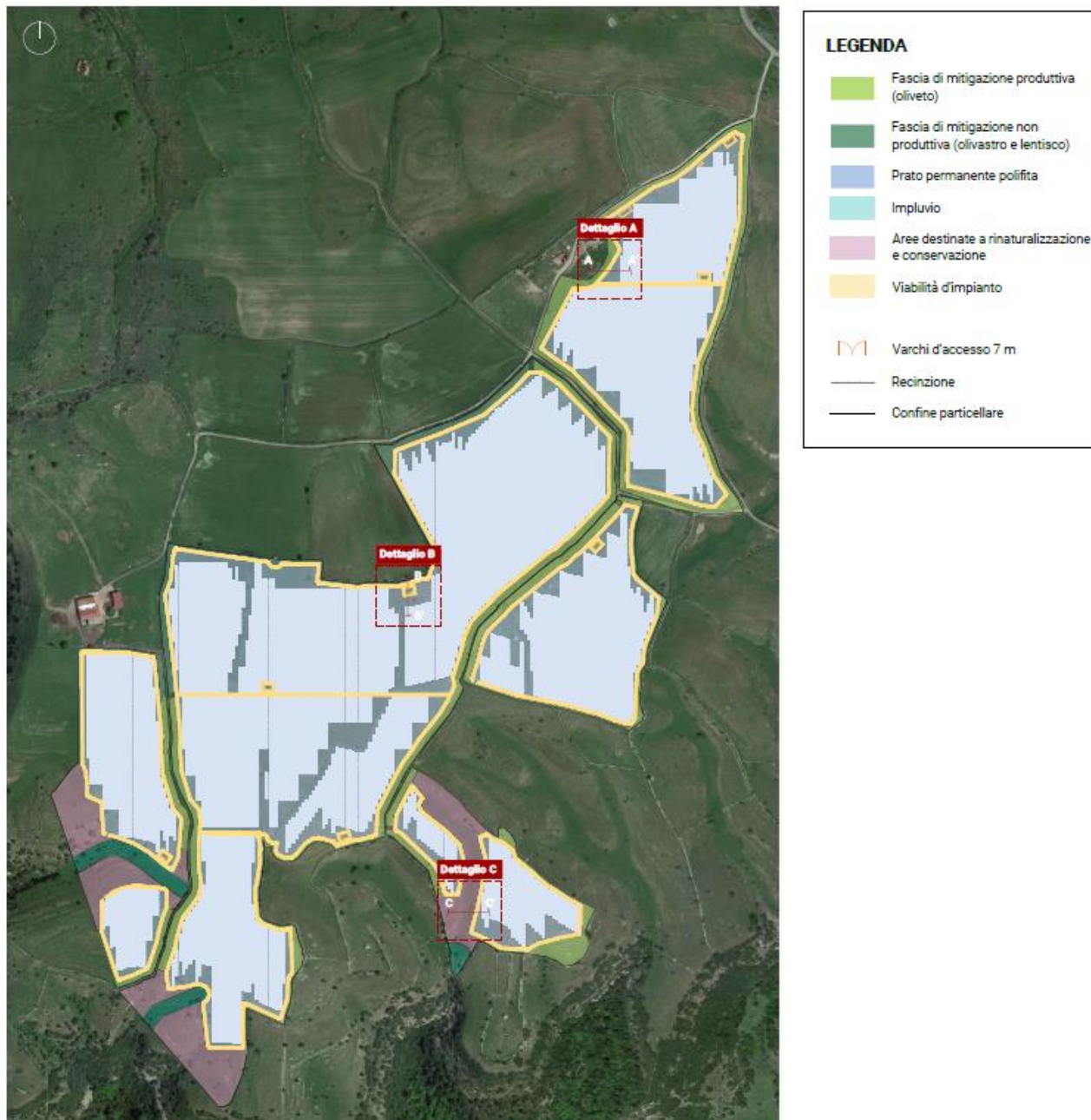
FIGURA 27 – PLANIMETRIA SISTEMAZIONE A VERDE OPERE DI MITIGAZIONE (ESTRATTO DALL'ELABORATO GRAFICO SIL-PDT11-R1 ) (IMMAGINE AGGIORNATA)
