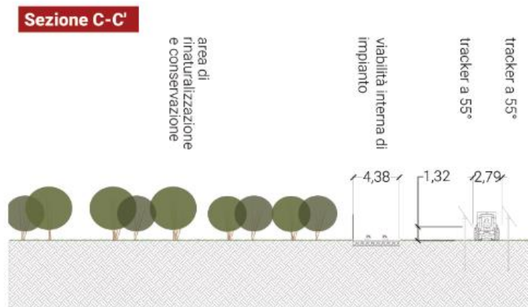
FIGURA 29 – PARTICOLARE FASCIA DI MITIGAZIONE E AREA DI COMPENSAZIONE – SEZIONE O-E DELL’IMPIANTO (ESTRATTO DALL’ELABORATO GRAFICO SIL-PDT11-R1 ) (IMMAGINE AGGIORNATA)
