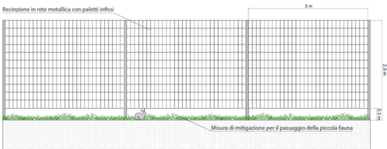
FIGURA 9: RECINZIONE TIPO
