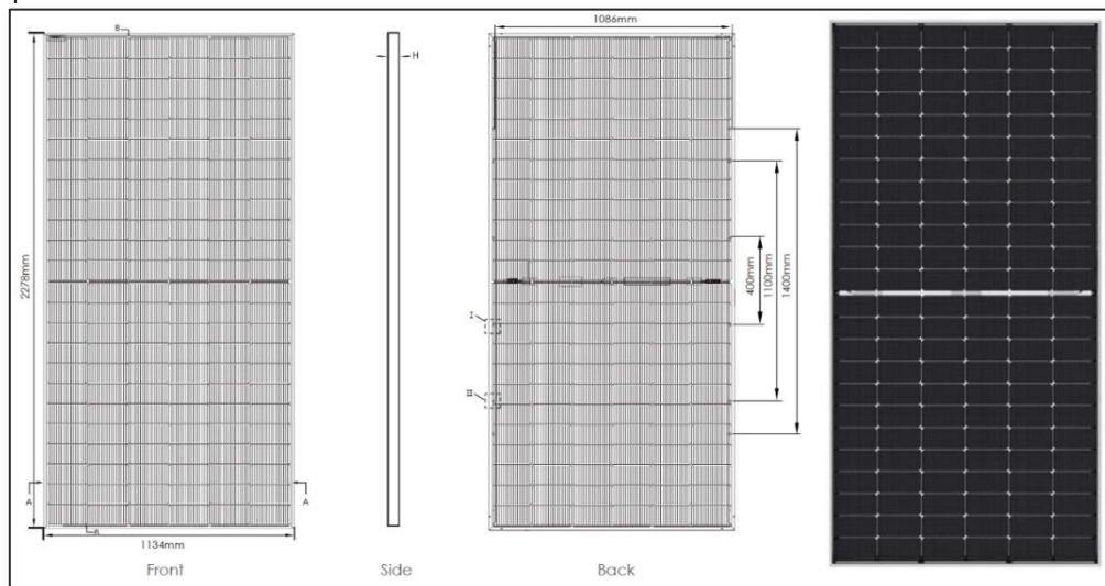
FIGURA 1 PANNELLO FV PARI A 570 WP – IN CONDIZIONI STANDARD - CON DIMENSIONI 2278 x 1134 x 30 MM
