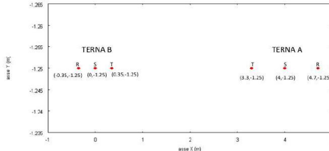
Figura 5: Geometria sorgenti
