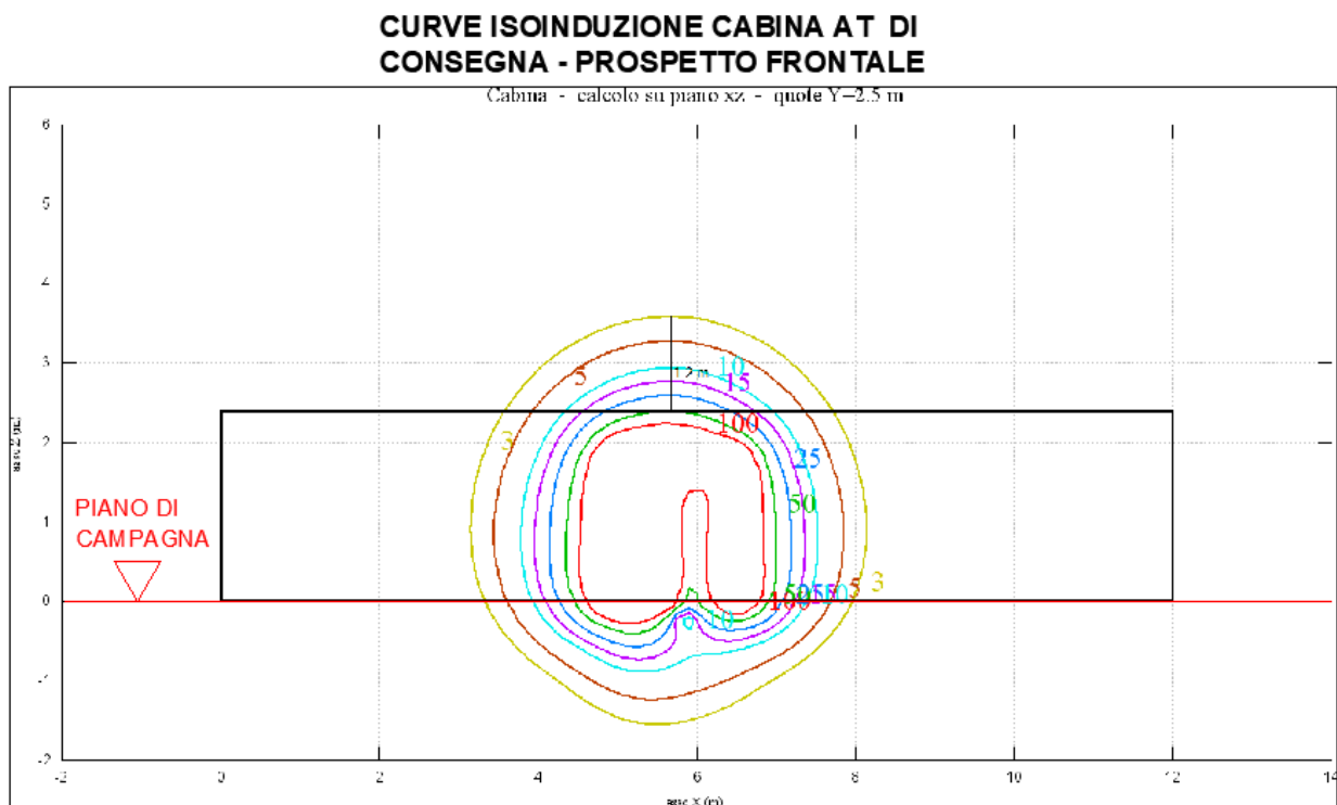
FIGURA 4: CURVE ISOINDUZIONE CABINA AT DI CONSEGNA (PROSPETTO FRONTALE)
