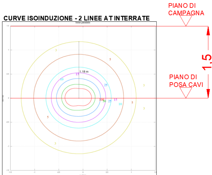
FIGURA 2: CURVE ISOINDUZIONE – 2 LINEE AT INTERRATE
