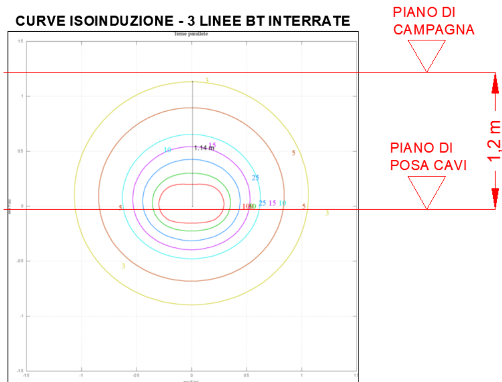
FIGURA 1: CURVE ISOINDUZIONE – 3 LINEE BT INTERRATE
