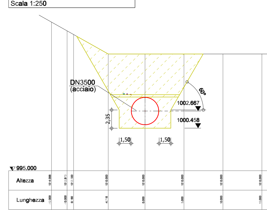
Sezione: 0+600 Scala 1:250
