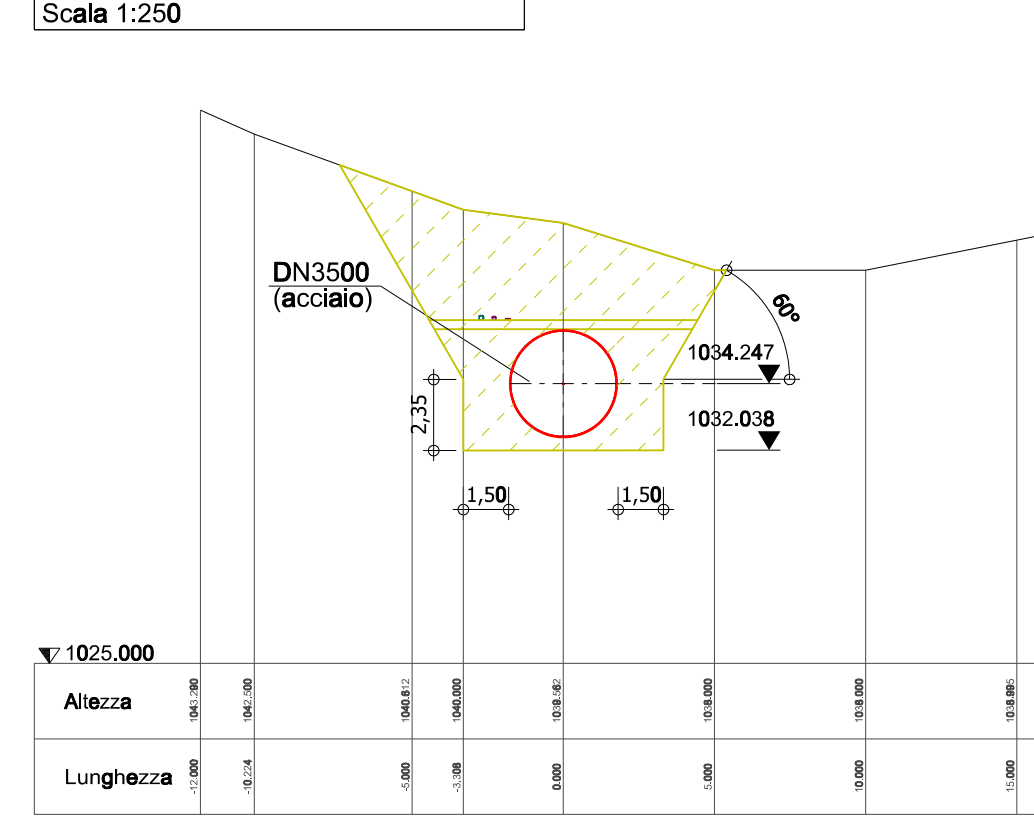
Sezione: 0+400 Scala 1:250
