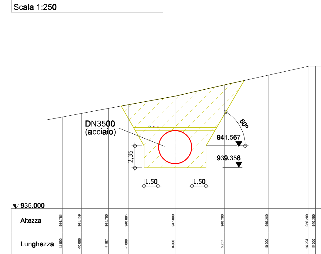
Sezione: 1+300 Scala 1:250
