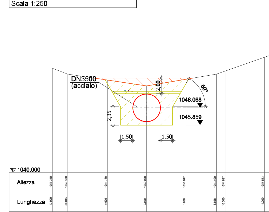
Sezione: 0+300 Scala 1:250
