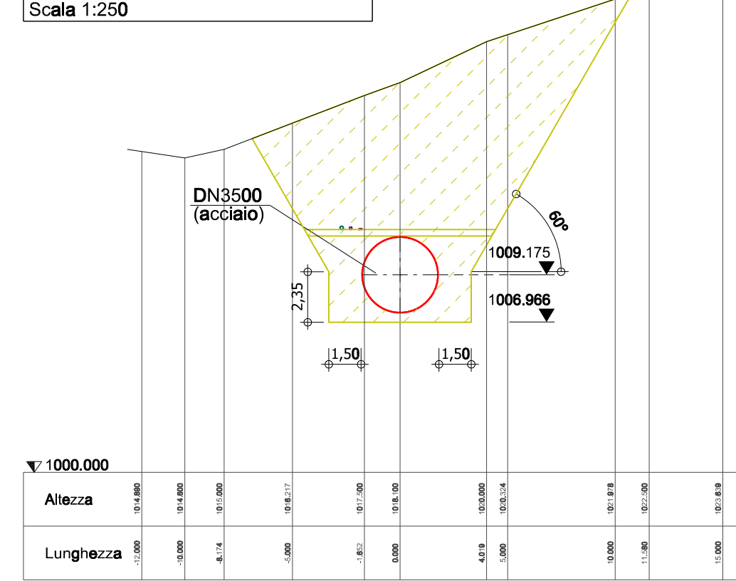
Sezione: 0+500 Scala 1:250
