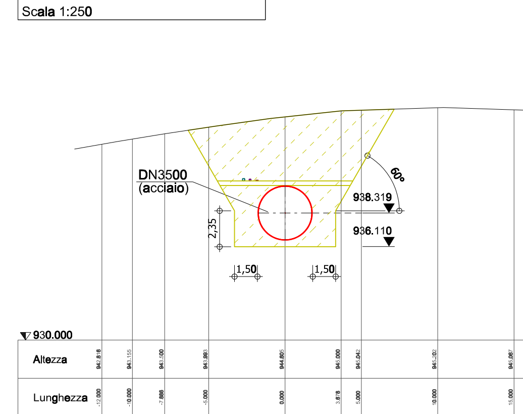
Sezione: 1+400 Scala 1:250
