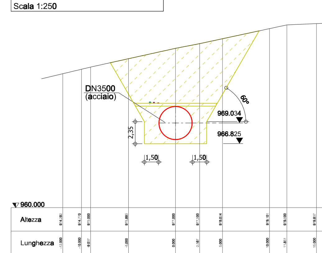
Sezione: 0+900 Scala 1:250
