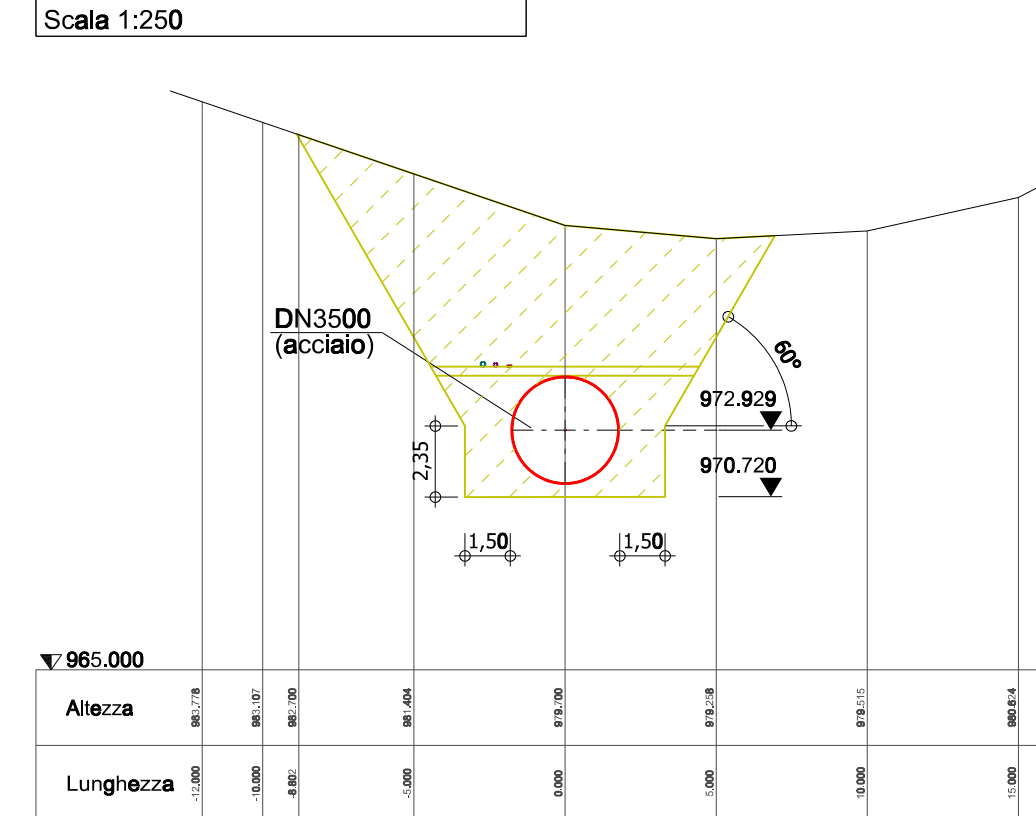
Sezione: 0+800 Scala 1:250
