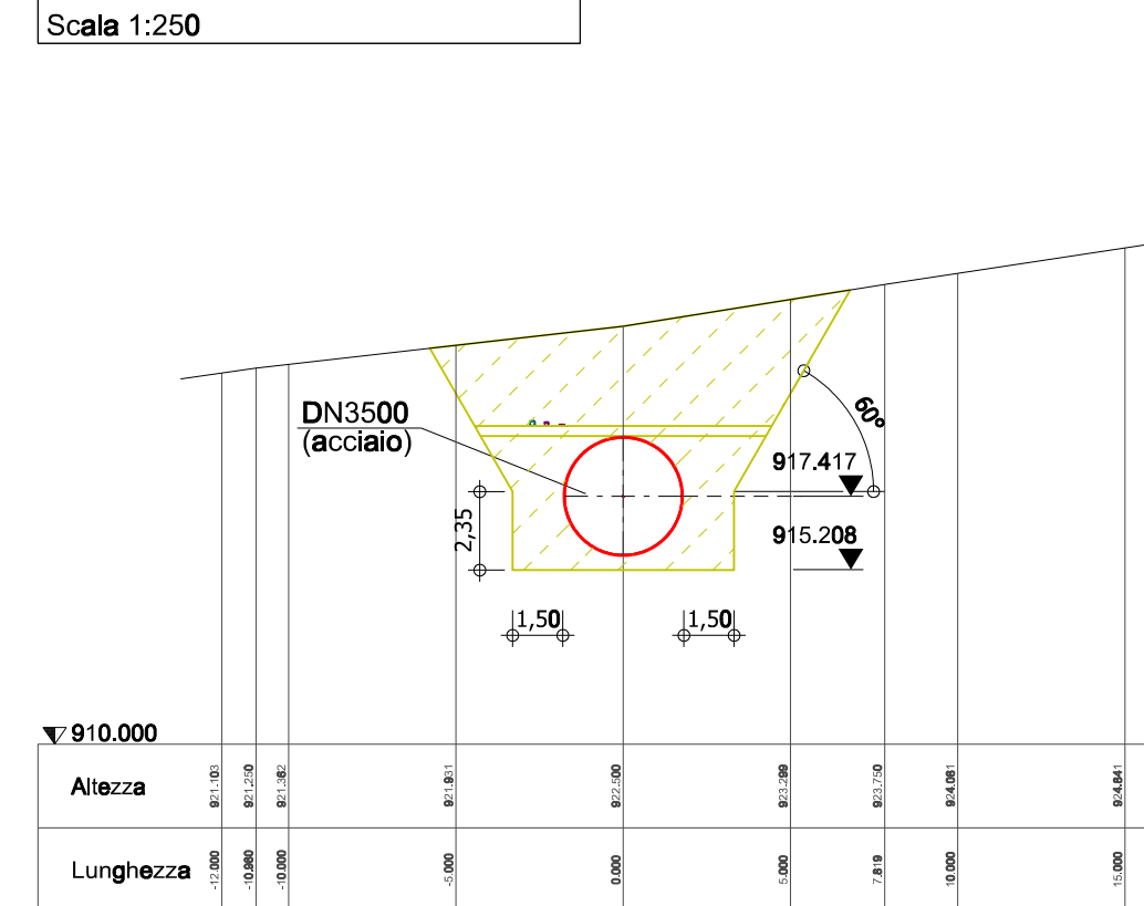
Sezione: 1+500 Scala 1:250
