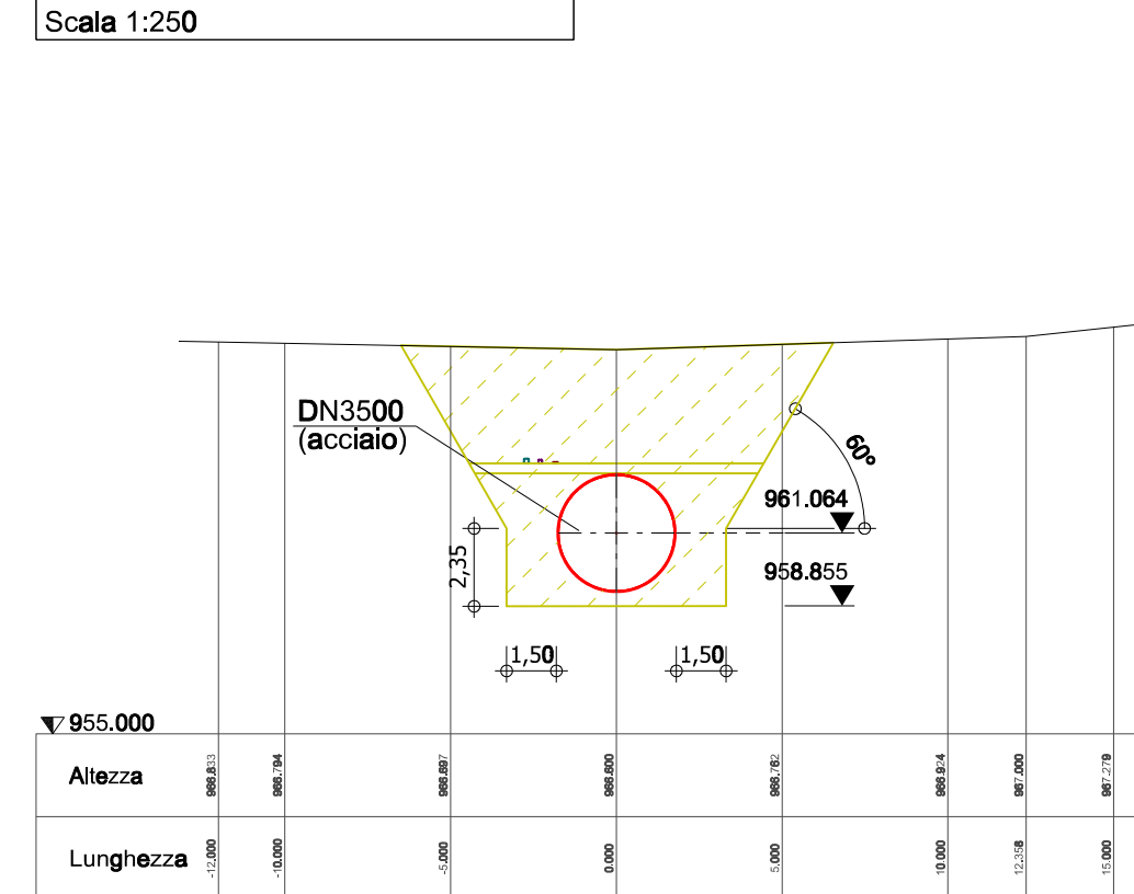
Sezione: 1+100 Scala 1:250
