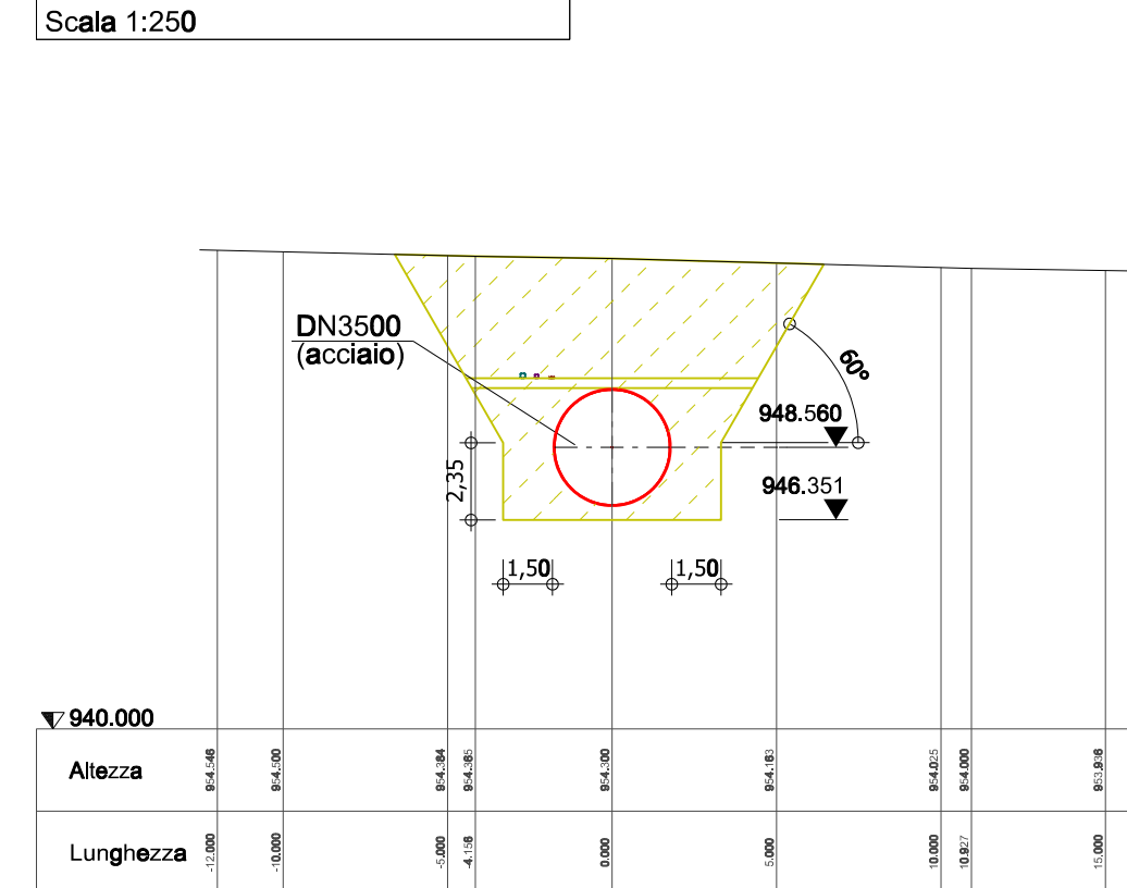
Sezione: 1+200 Scala 1:250
