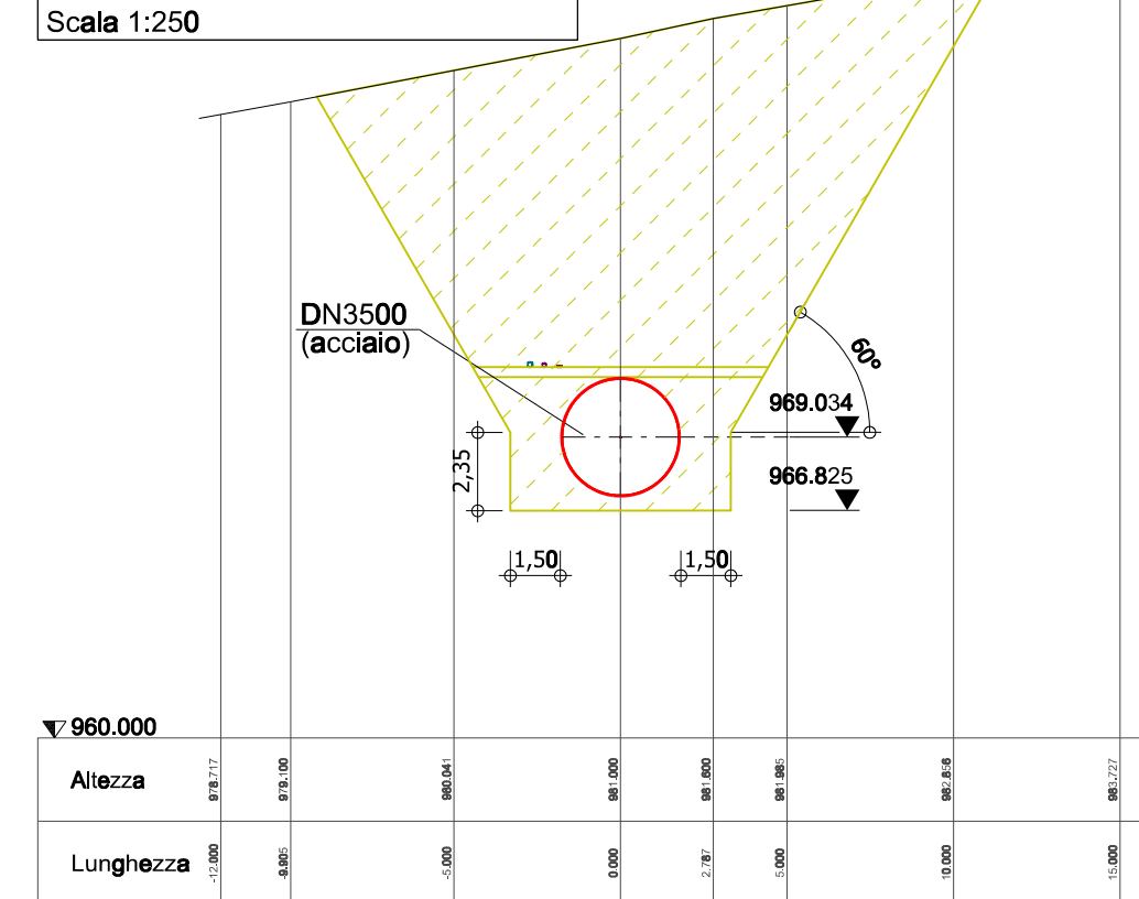
Sezione: 1+000 Scala 1:250
