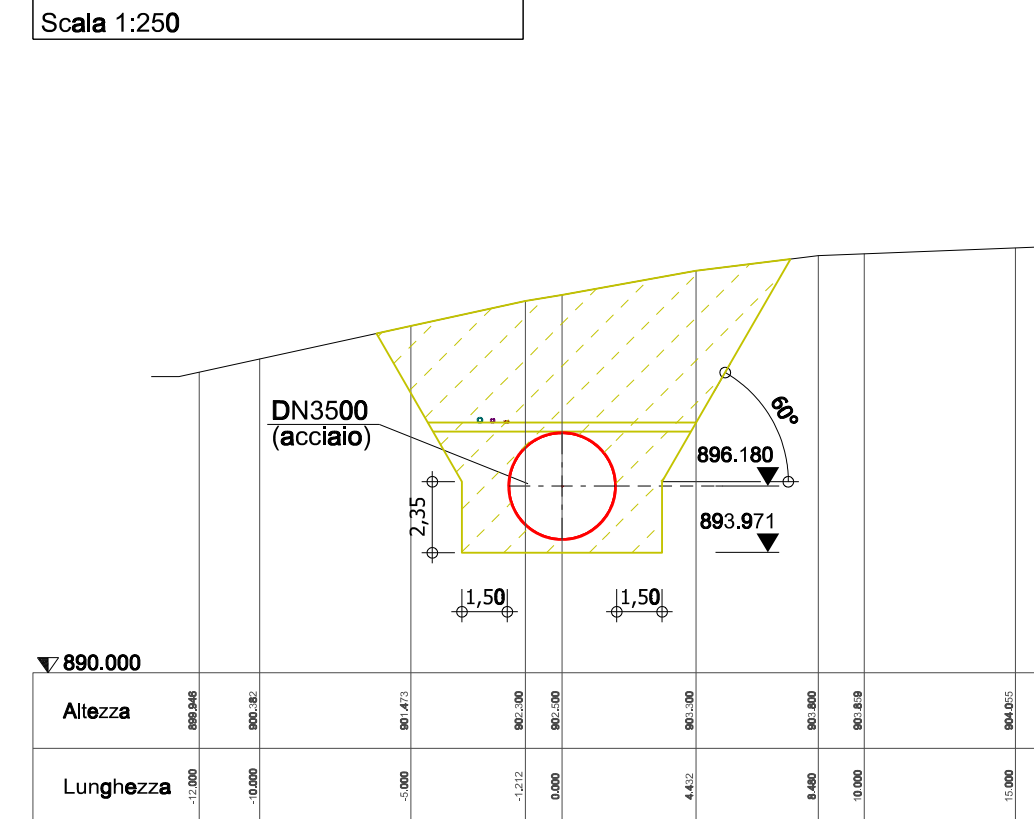
Sezione: 1+600 Scala 1:250
