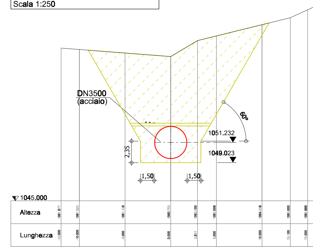
Sezione: 0+200 Scala 1:250
