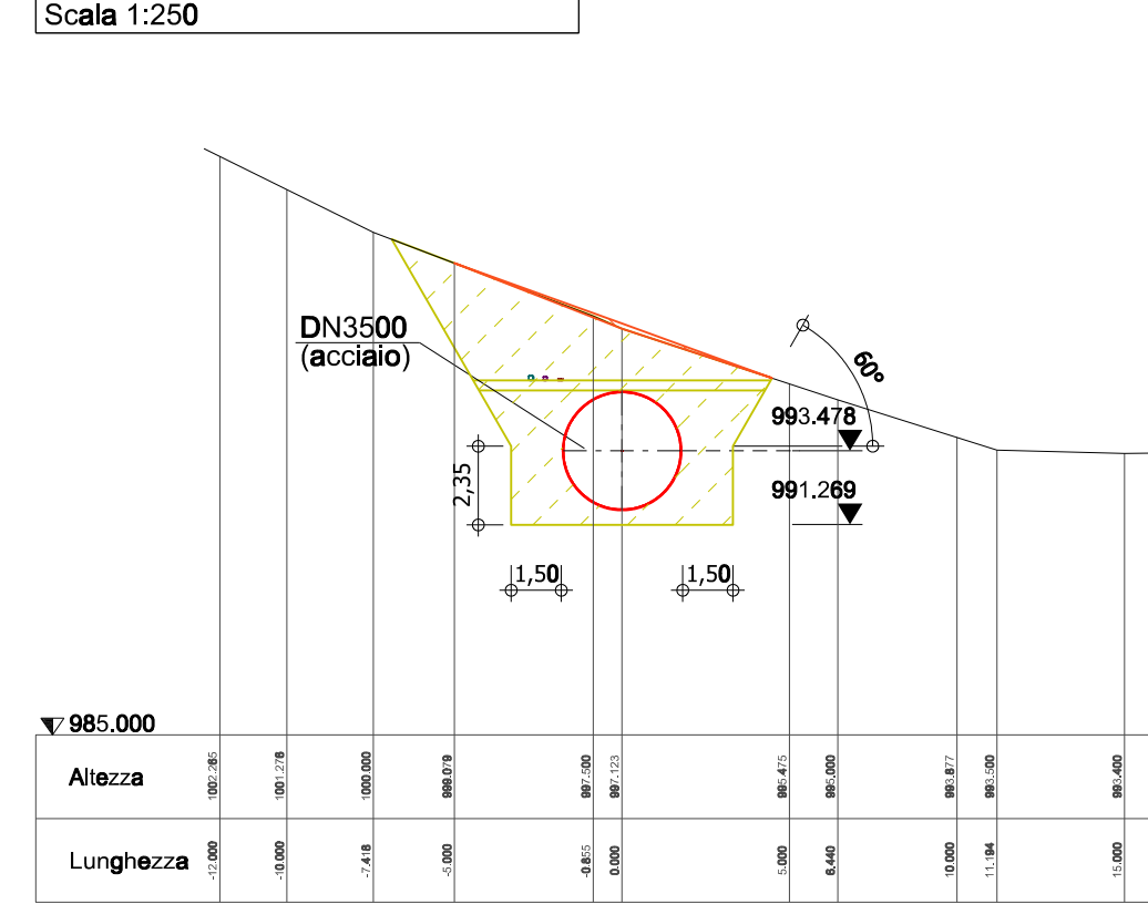
Sezione: 0+700 Scala 1:250
