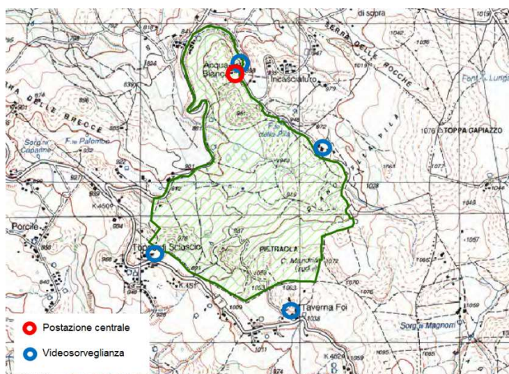
Figura 3. Installazioni di telerilevamento e videosorveglianza presso l'Abetina di Ruoti
