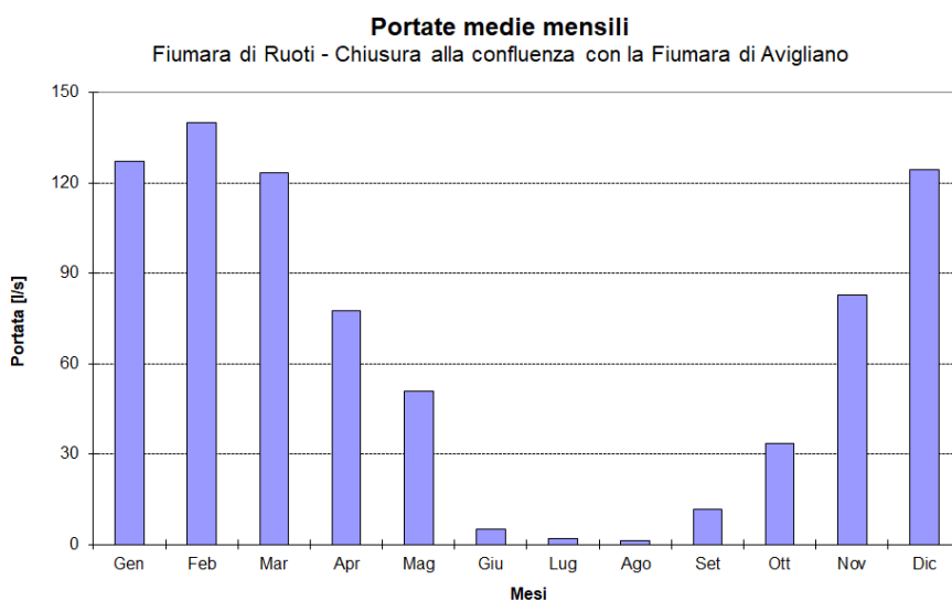
Figura 48. Portate medie mensili stimate all'imbocco del bacino di valle.
