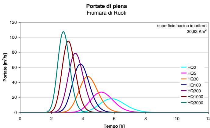
Figura 49. Idrogrammi di progetto per la fiumara di Ruoti determinati con la metodologia VAPI.
