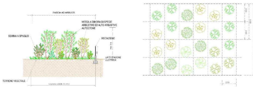
Figura 72. Zone tampone con fasce di arbusti in prossimità degli ingressi conduttori e schema di posa degli stessi.
