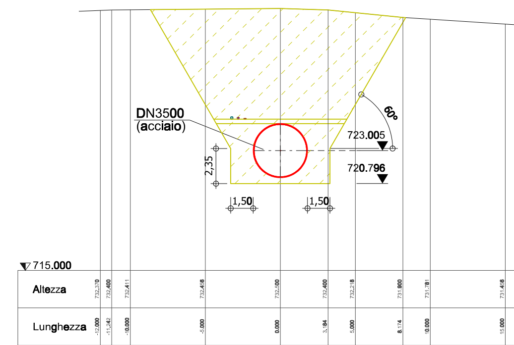
Sezione: 3+200 Scala 1:250
