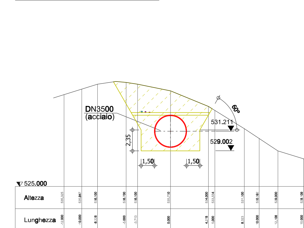
Sezione: 4+500 Scala 1:250
