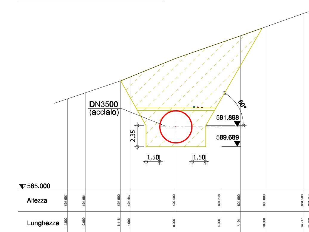
Sezione: 4+100 Scala 1:250
