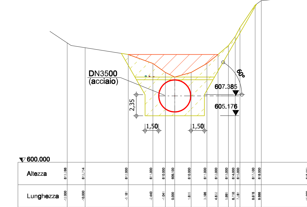
Sezione: 3+600 Scala 1:250
