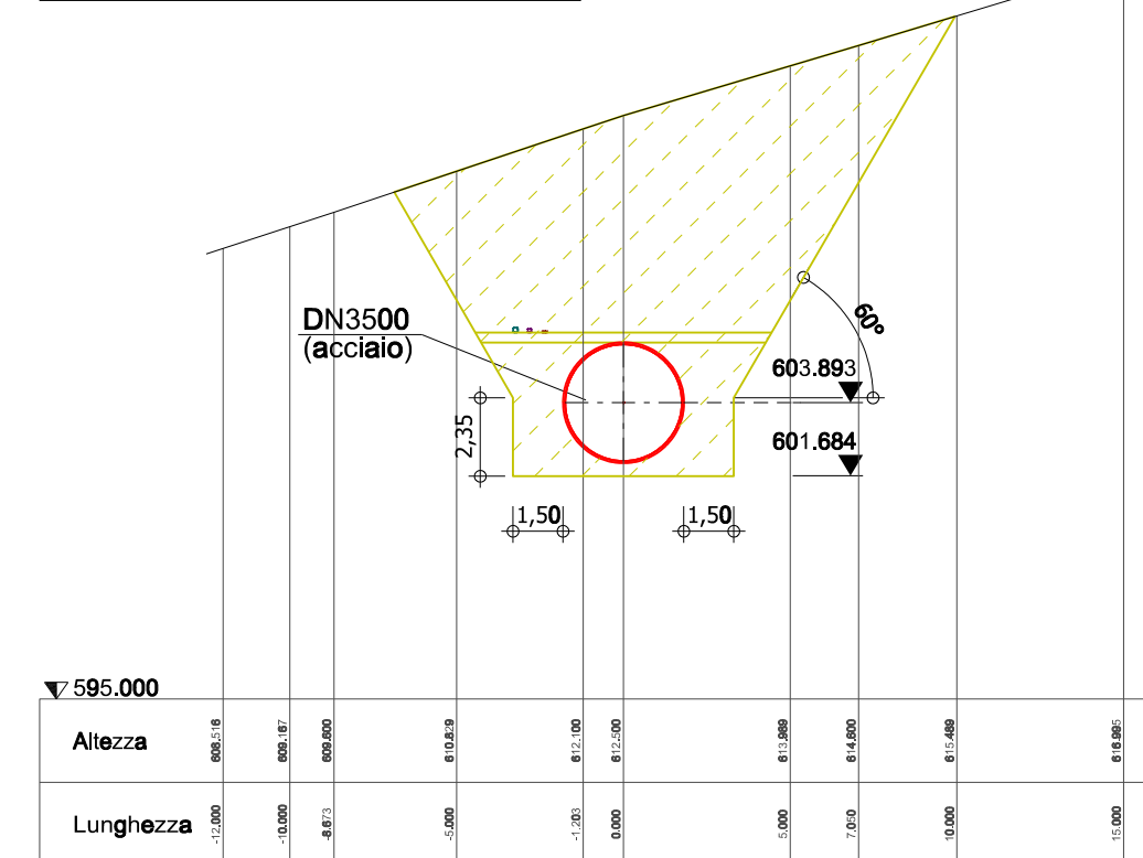
Sezione: 3+700 Scala 1:250
