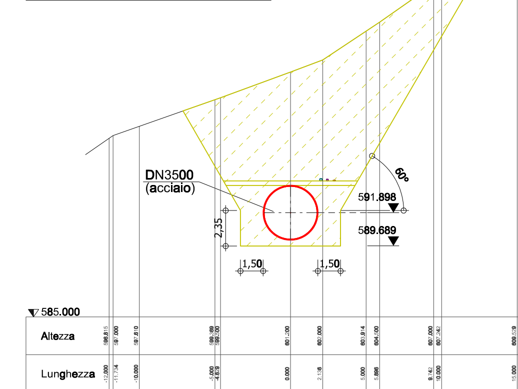
Sezione: 4+000 Scala 1:250
