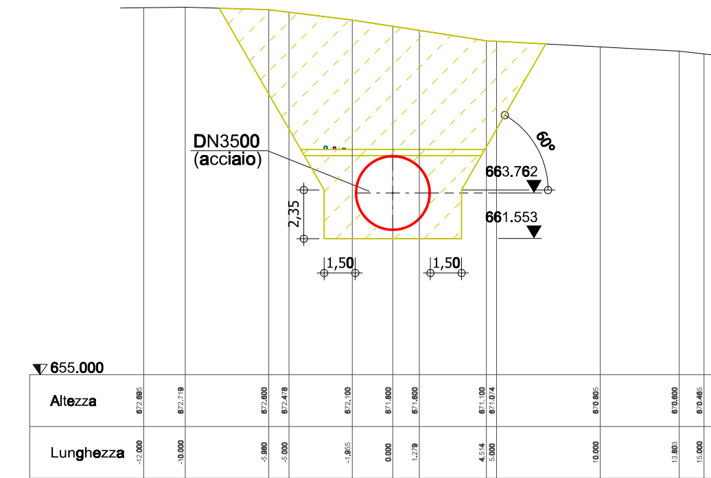
Sezione: 3+400 Scala 1:250
