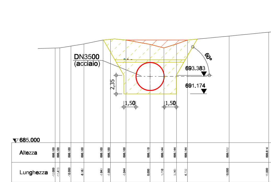
Sezione: 3+300 Scala 1:250
