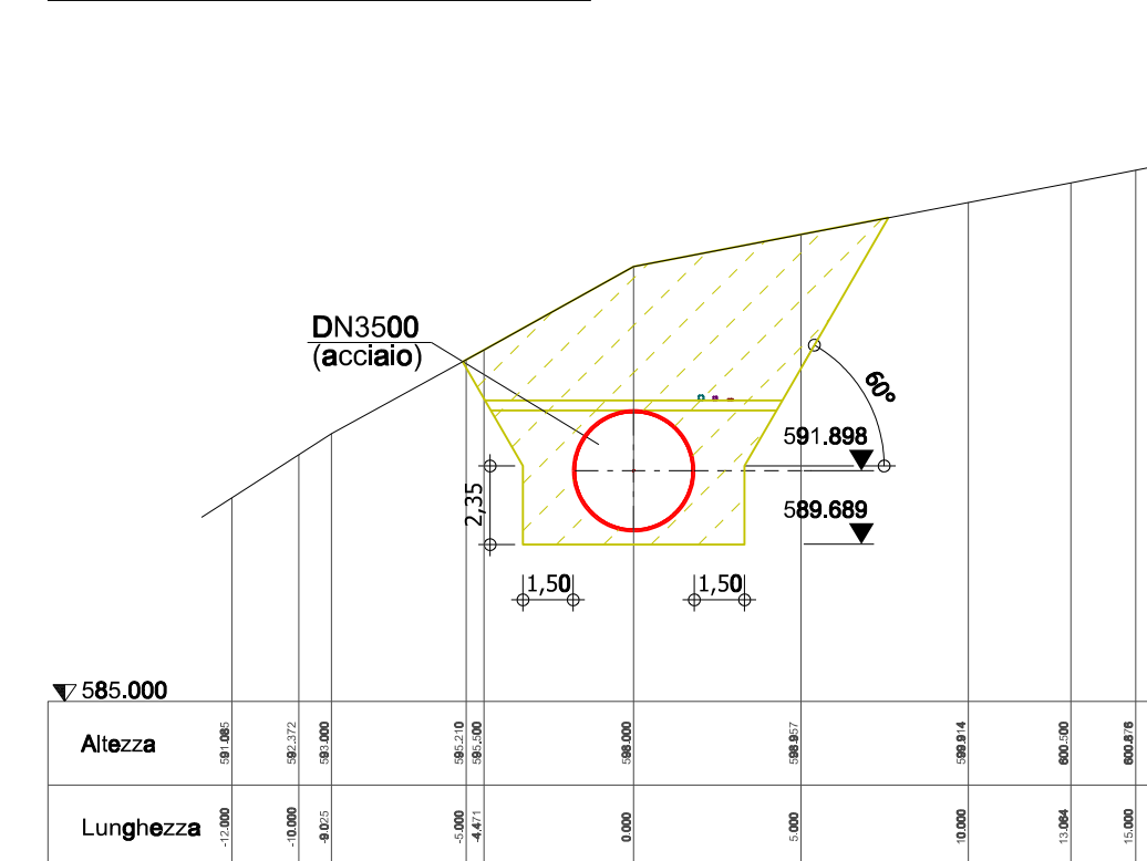
Sezione: 3+900 Scala 1:250
