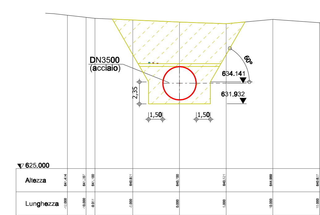
Sezione: 3+500 Scala 1:250
