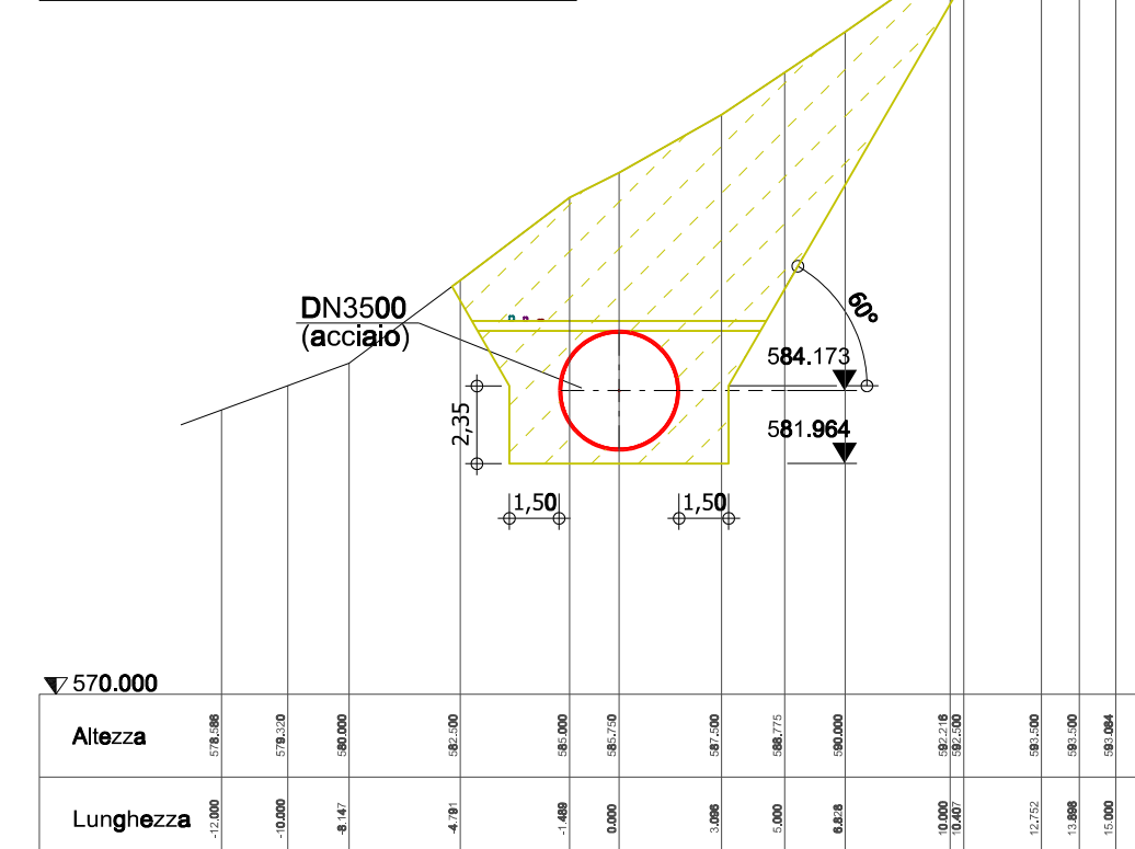
Sezione: 4+200 Scala 1:250
