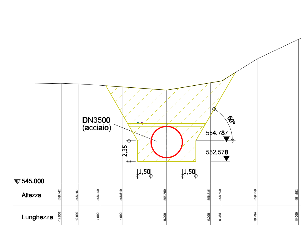
Sezione: 4+300 Scala 1:250
