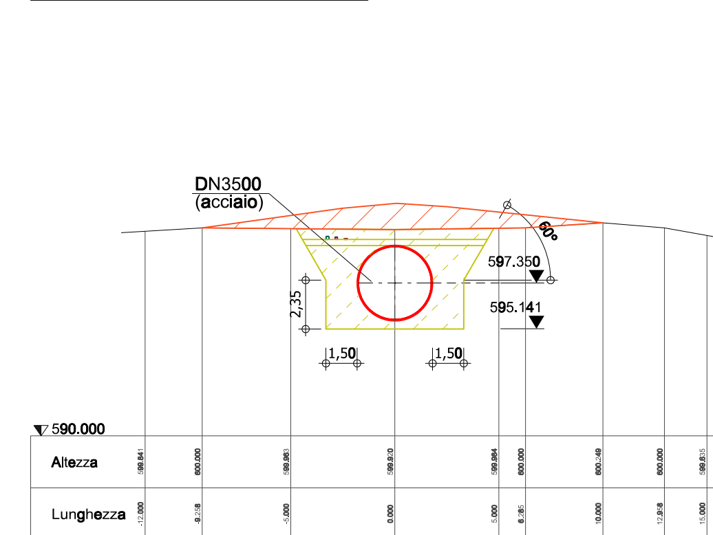
Sezione: 3+800 Scala 1:250
