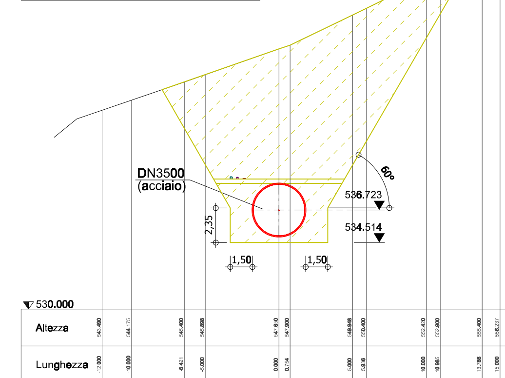
Sezione: 4+400 Scala 1:250
