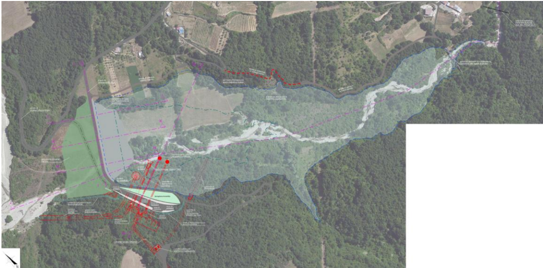
Figura 3. Planimetria di progetto dell'invaso di valle (estratto Tavola PD-EP.19.1).
