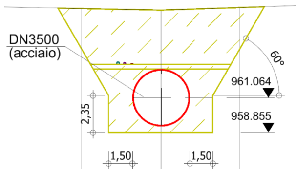
Figura 4. Sezione tipologia indicativa delle modalità di posa della condotta forzata (estratto Tavola PD-EP.21.4.1).
