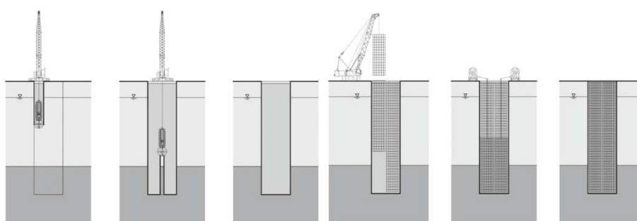
Figura 7. Procedimento multi-fase per una gestione ottimale dello scavo con stabilizzazione finale con gabbie in acciaio e strutture portanti in cemento armato.
