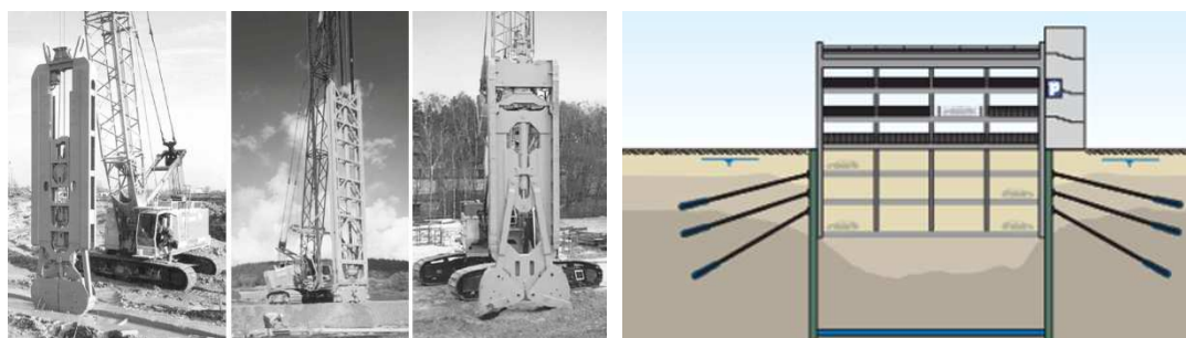
Figura 8. Un esempio dei macchinari che saranno utilizzati ed un esempio dello schema finale dei lavori applicabile all'intero corpo solido dell'edificio di centrale.
