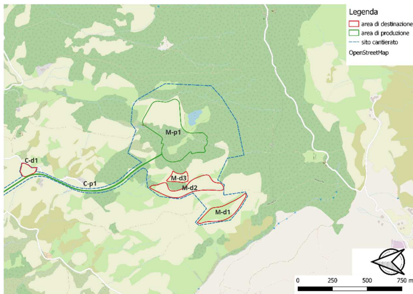
Figura 10. Identificazione del sito cantierato, delle aree di produzione e delle aree di destinazione dei materiali scavati presso l'areale del bacino di monte.
