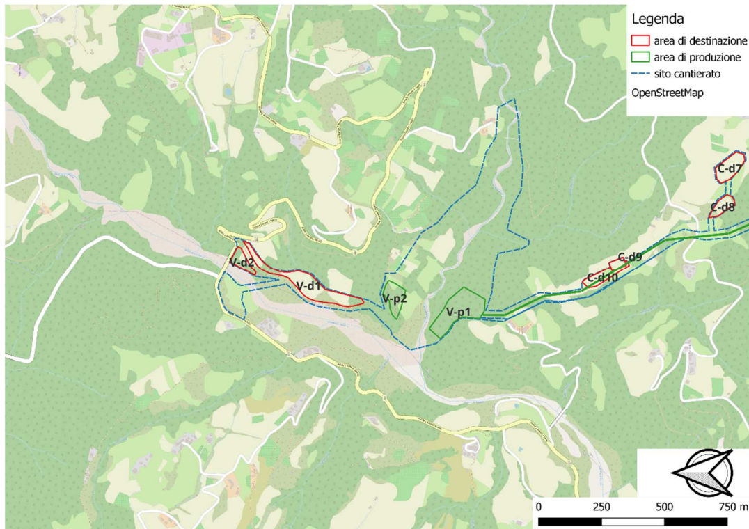
Figura 14. Identificazione del sito cantierato, delle aree di produzione e delle aree di destinazione dei materiali scavati per l'areale della centrale di produzione, della diga, dell'invaso di valle e della strada principale di accesso.
