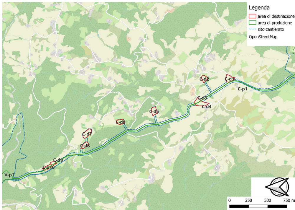
Figura 13. Identificazione del sito cantierato, delle aree di produzione e delle aree di destinazione dei materiali scavati lungo il tracciato della condotta forzata.
