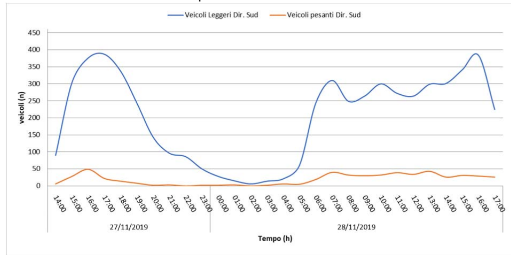
Evoluzione temporale del traffico in SS12 dir. Sud
