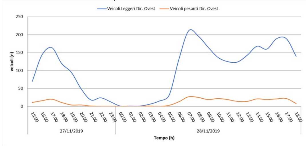
Evoluzione temporale del traffico in SS242 dir. Ovest
