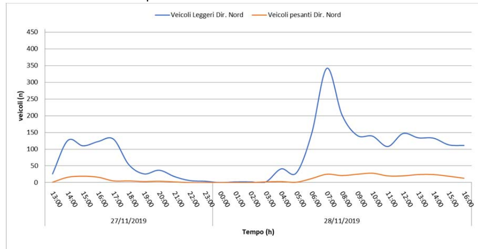
Evoluzione temporale del traffico in Via Julius Durst dir. Nord
