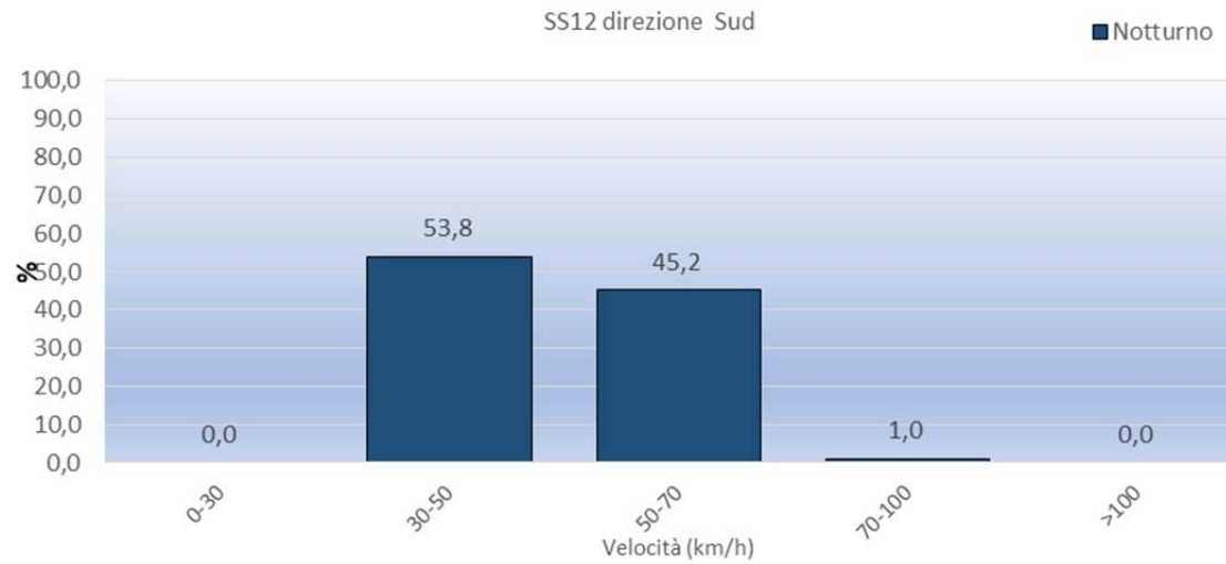
SS12: Percentuale di veicoli per classi di velocità nel periodo notturno
