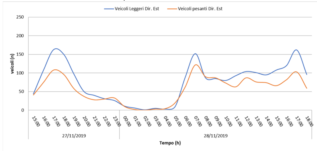
Evoluzione temporale del traffico in SS242 dir. Est
