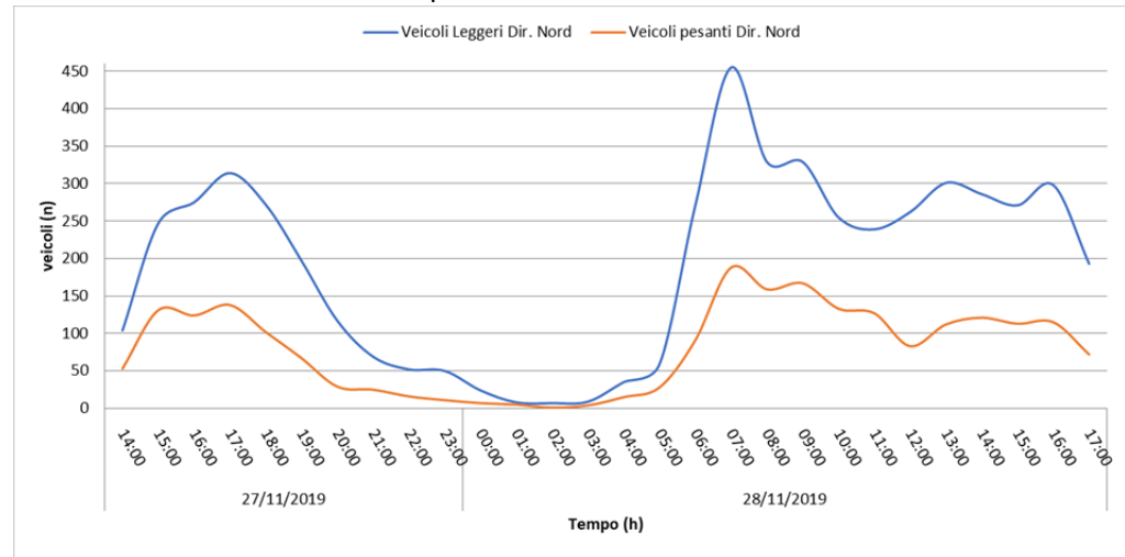
Evoluzione temporale del traffico in SS12 dir. Nord
