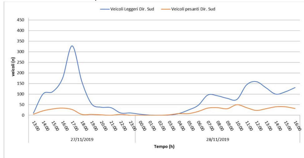
Evoluzione temporale del traffico in Via Julius Durst dir. Sud
