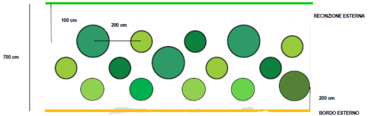
Figura 12.2 – Sezione tipo fascia di mitigazione.
