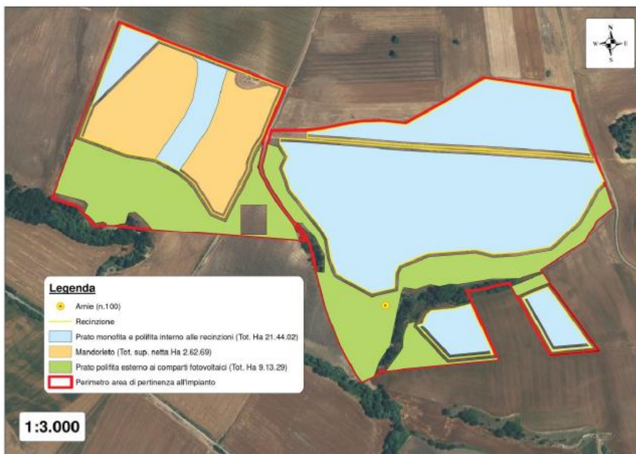
Figura 12.3 – Stralcio impianto grivoltaico.
