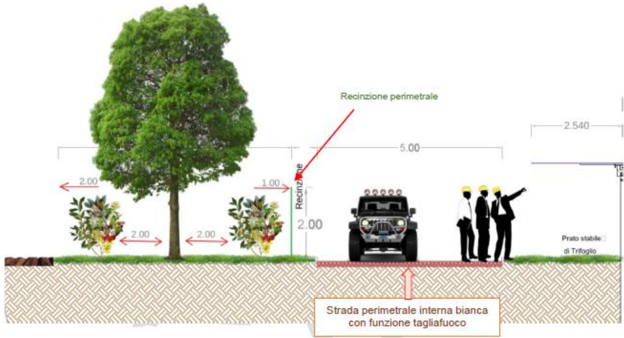
Figure 12.1. – Sezione tipo Aree coltivate.
