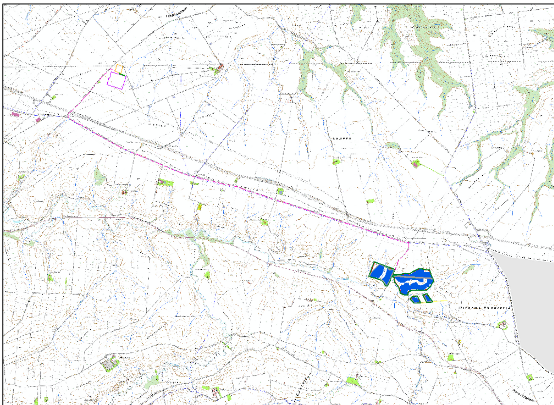
Figura 3.3 - Stralcio impianto su base CTR
