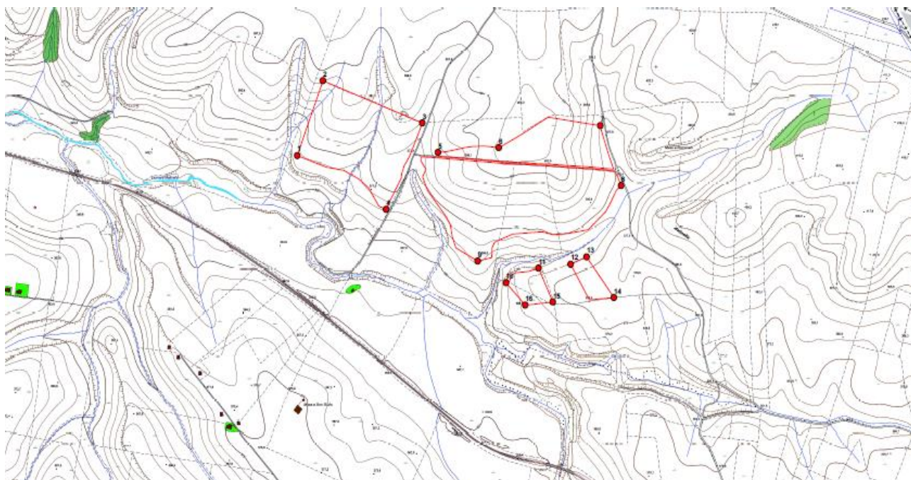
Figura 3.4 – Perimetrazione area impianto
