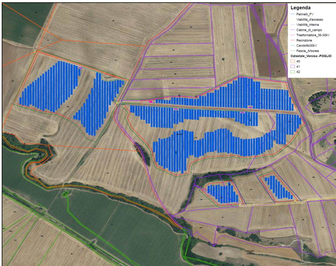
Figure 3.7 Progetto dell'impianto FV su ortofoto e catastale
