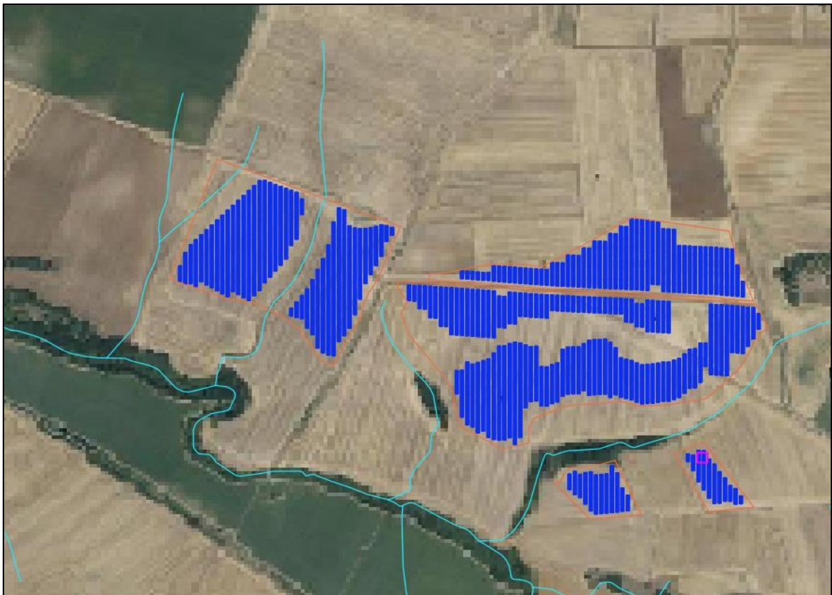
Figure 5.6 Dettaglio dell'Idrografia
