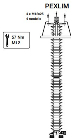
Fig. 16. Particolare di dettaglio dello scaricatore AT
