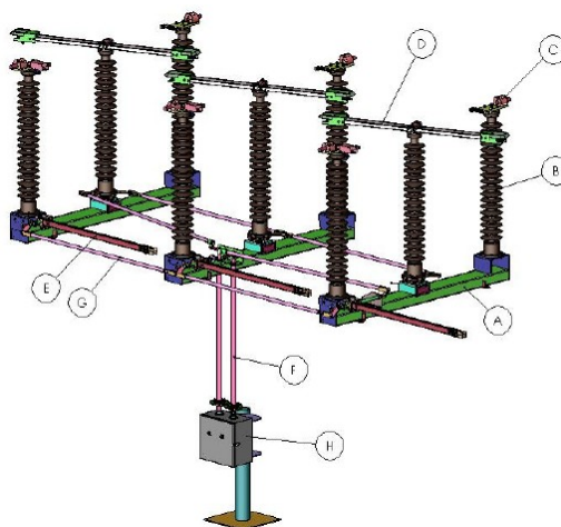
Fig. 17. Parti principali che compongono un sezionatore.
