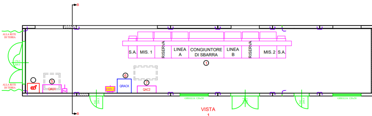
Fig. 8. Tipico PIANTA della Cabina di Raccolta: locale destinato a soli Quadri MT (dimensioni principali 15,00 x 3,00 x 4,50h).
