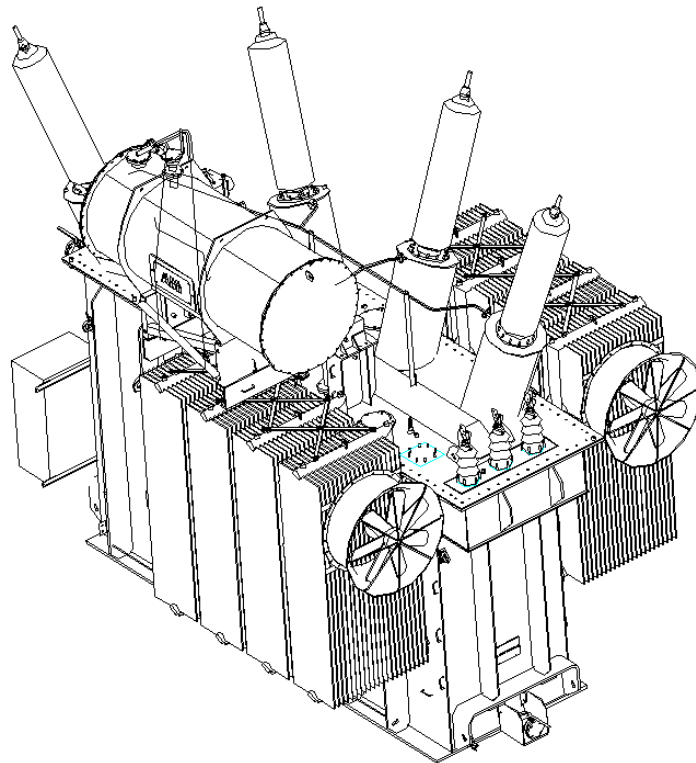
Fig. 22. Vista assometrica del trasformatore di progetto
