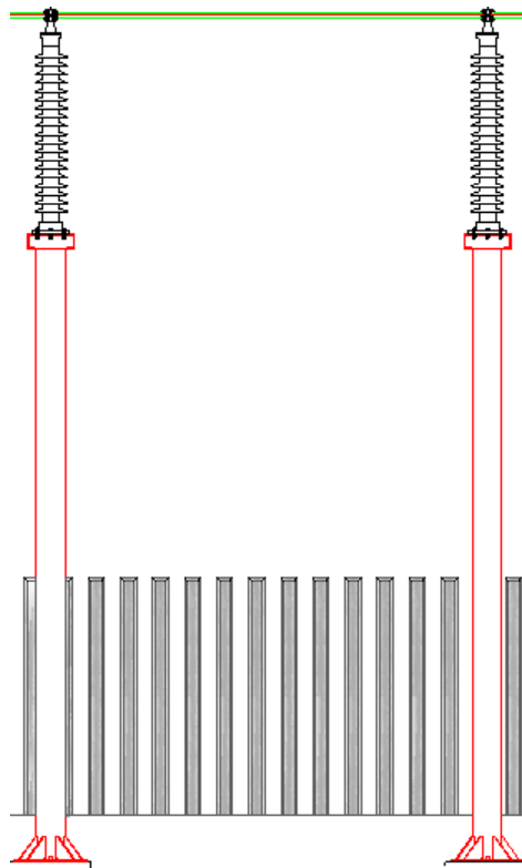
Fig. 20. Particolare prospettico dei supporti rompitratta unipolari
